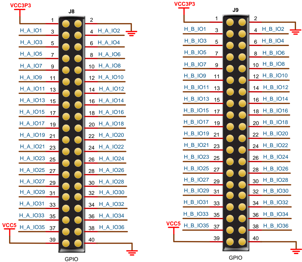
图 3-9 GPIO 电路
