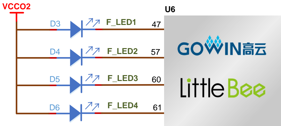
图 3-6 LED 电路
