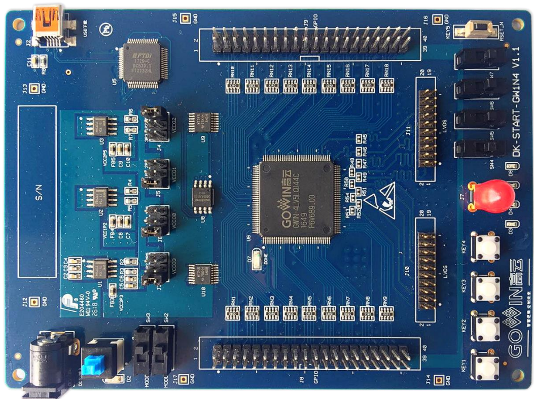
图 2-1 DK-START-GW1N V1.1 开发板
