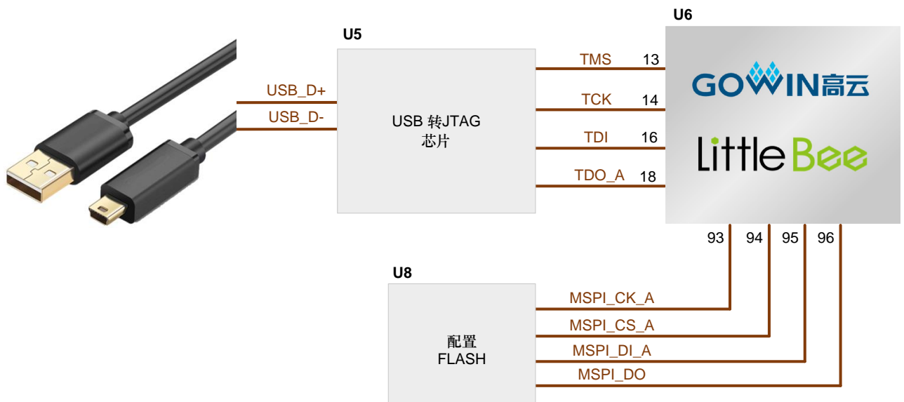
图 3-3 FPGA USB 下载与配置连接示意图
