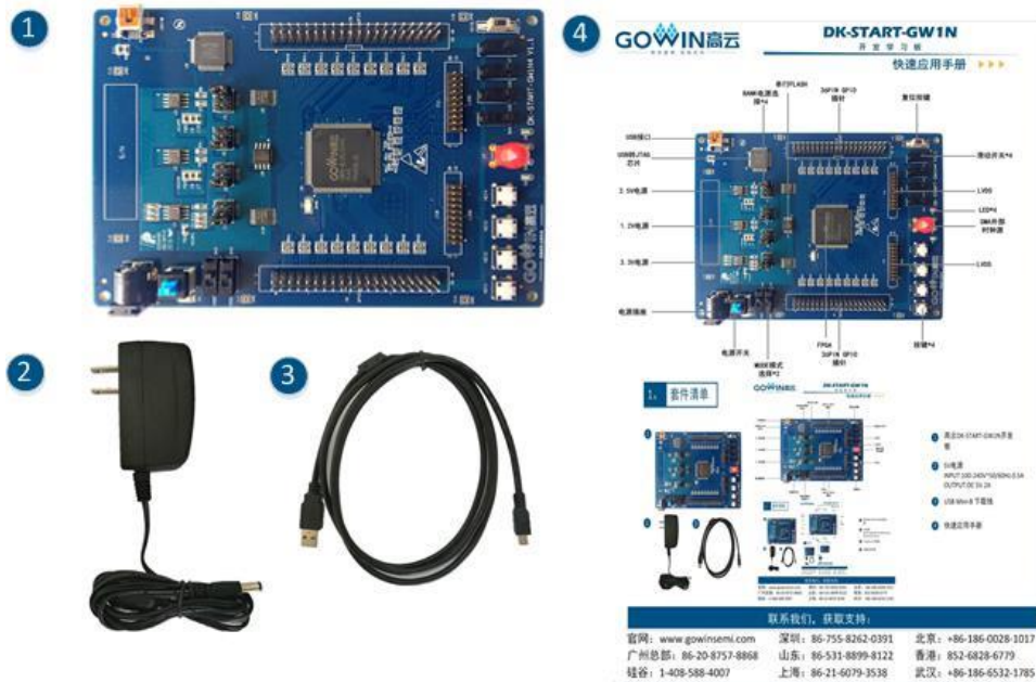
图 2-2 开发板套件
