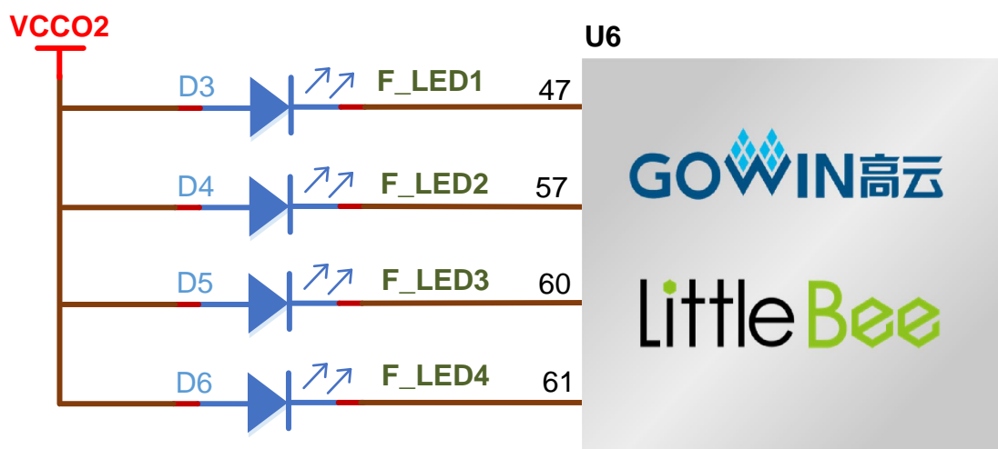
图 3-4 LED 电路
