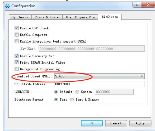
图 4-1 Download Speed
