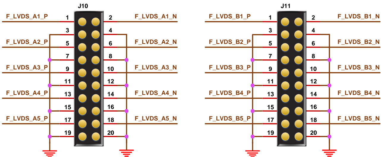
图 3-8 LVDS 电路
