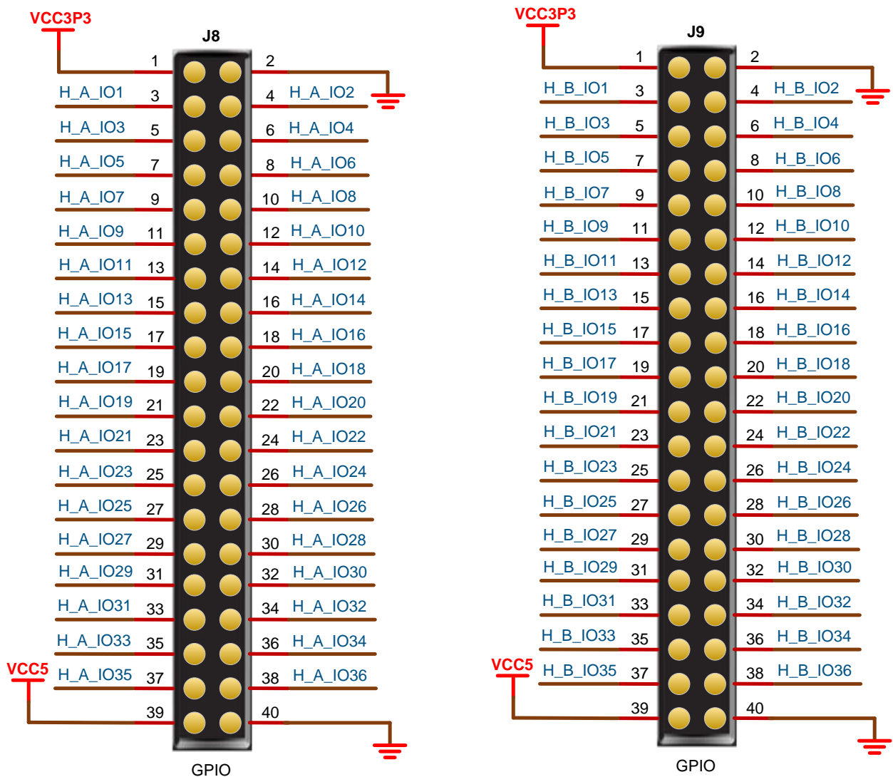
图 3-7 GPIO 电路
