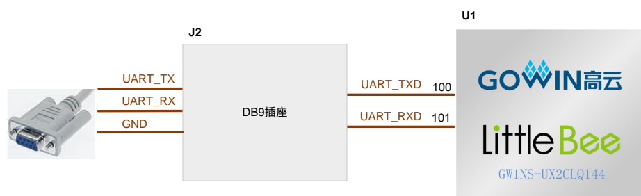
图 3-13 RS232 下载连接示意图
