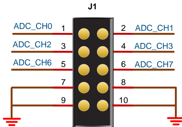
图 3-12 ADC 电路
