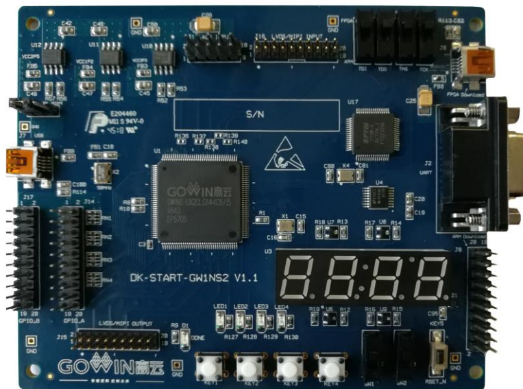
图 2-1 DK-START-GW1NS2 开发板
