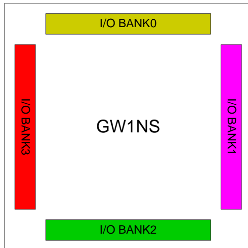
图 3-1 GW1NS 系列 FPGA 产品 I/O BANK 整体示意图
