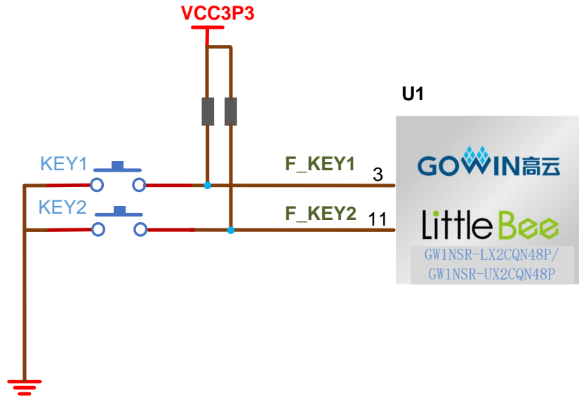
图 3-7 按键电路
