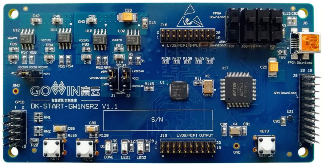
图 2-1 DK-START-GW1NSR2 V2.1 开发板
