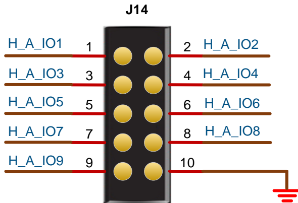
图 3-8 GPIO 电路
