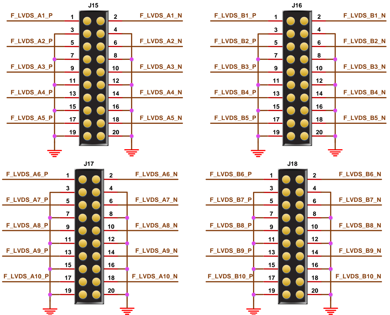
图 3-10 LVDS 电路
