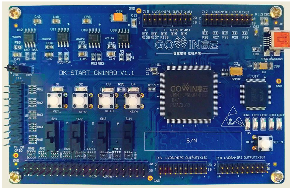
图 2-1 DK-START-GW1NR9 开发板
