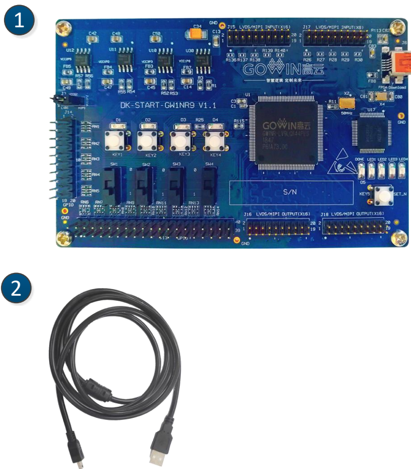
图 2-2 开发板套件
