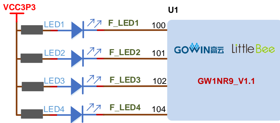
图 3-6 LED 电路
