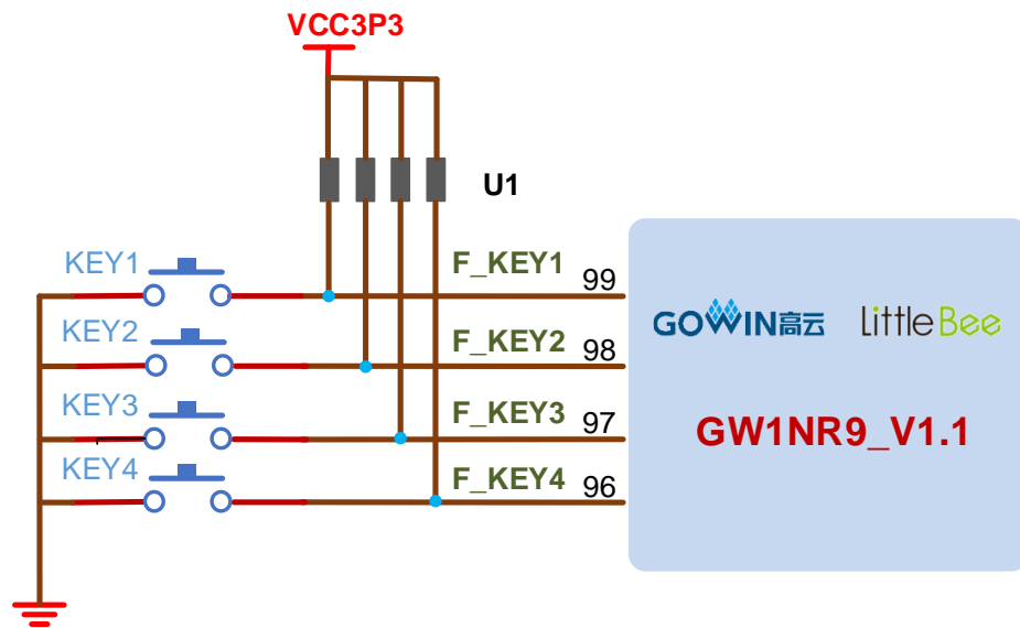
图 3-8 按键电路
