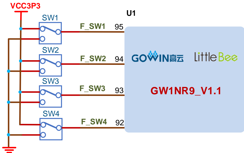
图 3-7 开关电路
