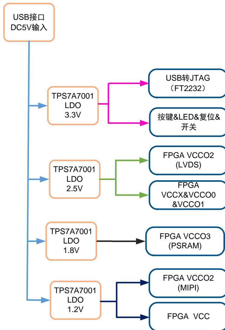
图 3-4 电源系统分配示意图
