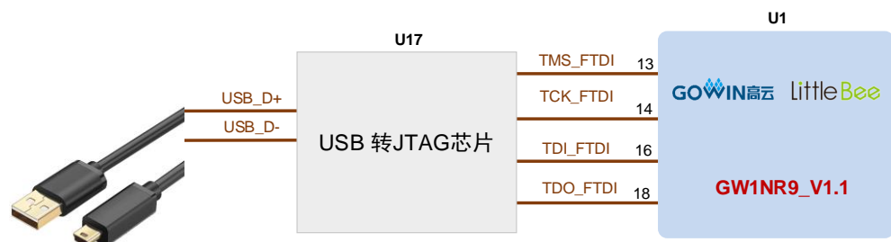
图 3-3 FPGA USB 下载连接示意图
