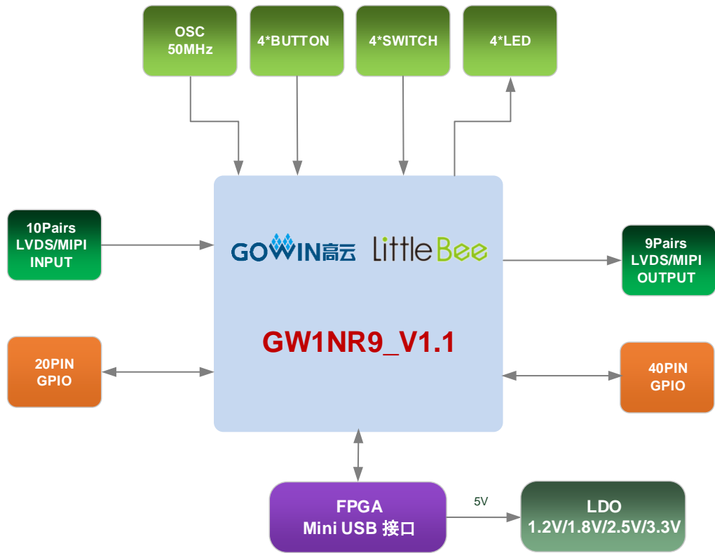
图 2-4 系统框图
