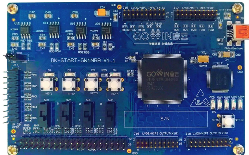
图 2-1 DK-START-GW1NR9 V1.1 开发板
