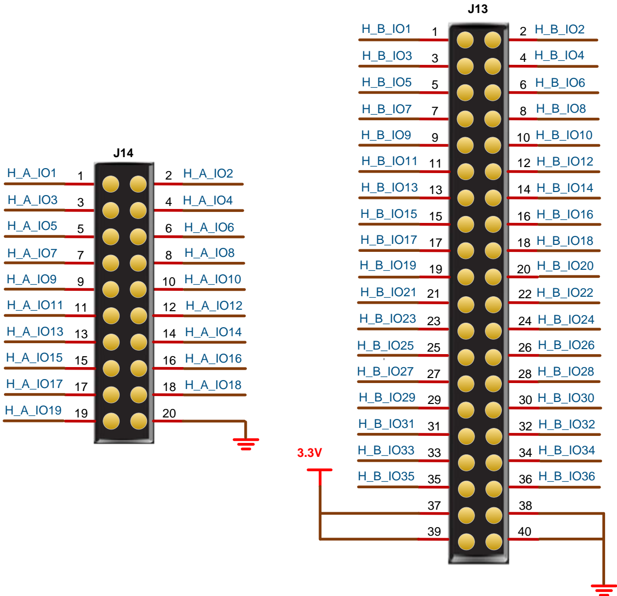
图 3-9 GPIO 电路
