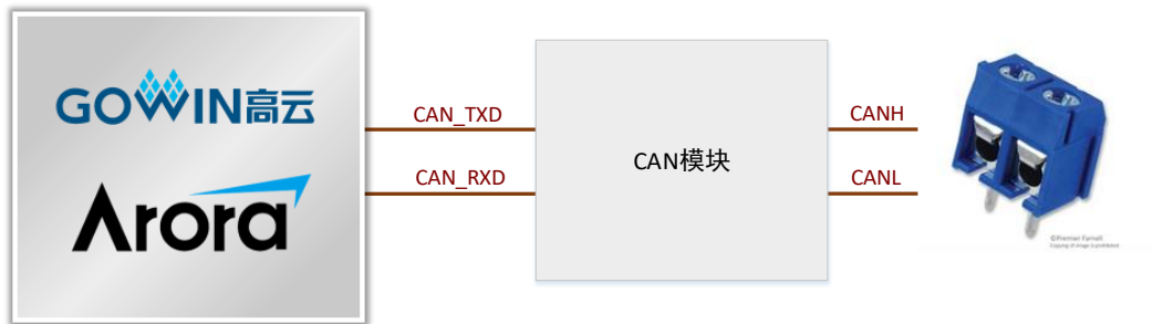
图 3-15 CAN 模块连接示意图
