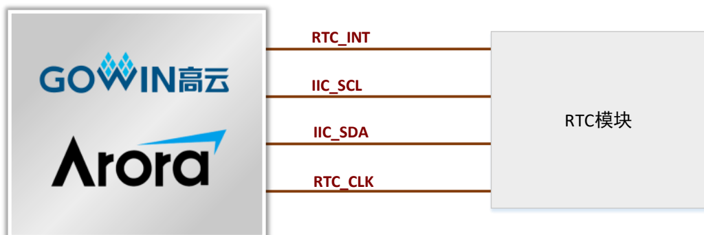
图 3-13 RTC 模块连接示意图
