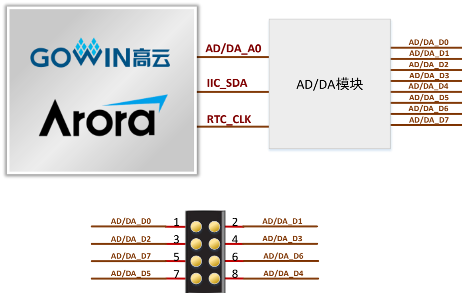
图 3-14 AD/DA 模块连接示意图
