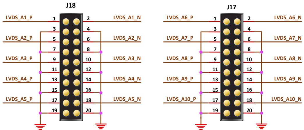
图 3-9 LVDS RX 接口示意图
