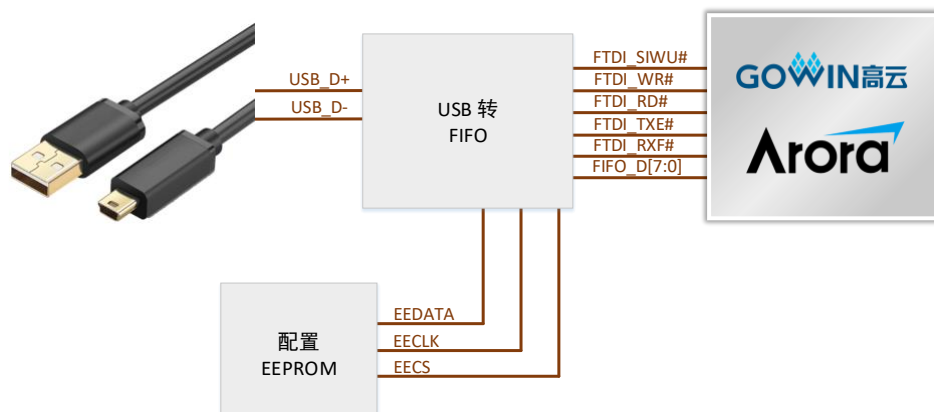
图 3-4 异步 FIFO 连接示意图
