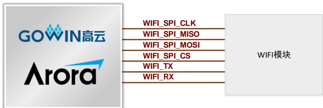
图 3-16 WIFI 模块连接示意图
