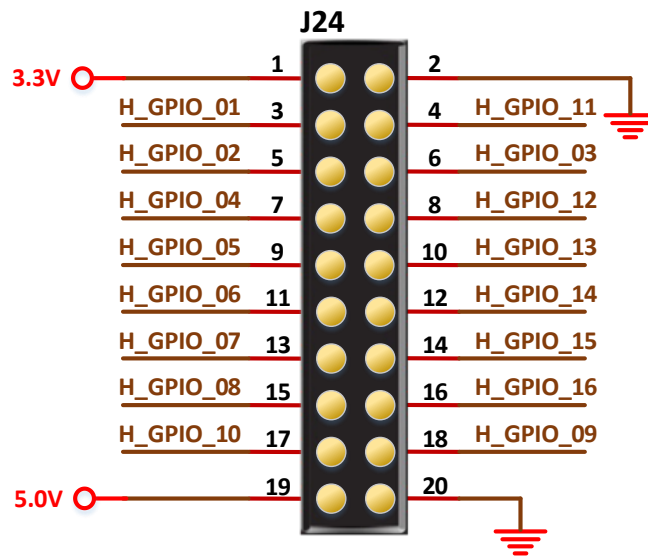
图 3-18 20pin 接口示意图
