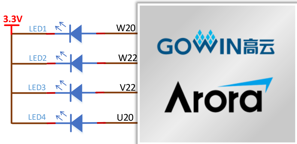
图 3-20 LED 连接示意图
