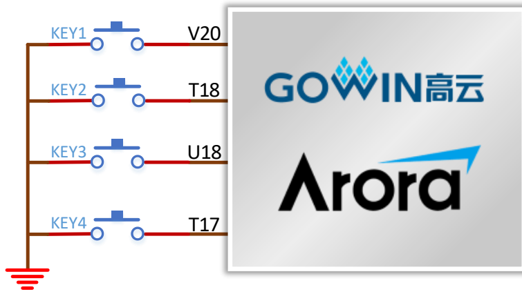
图 3-21 按键电路
