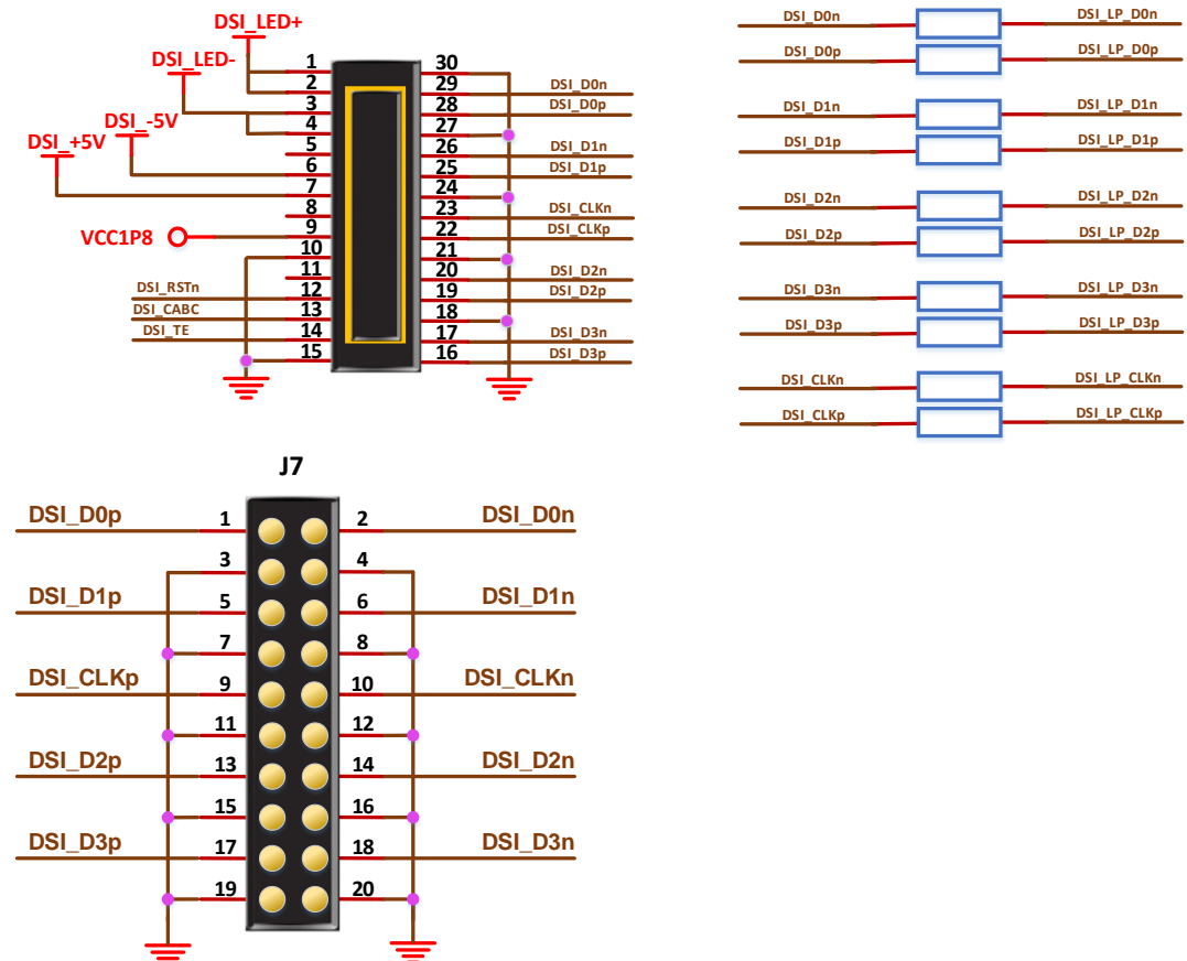
图 3-10 MIPI DSI 模块连接示意图
