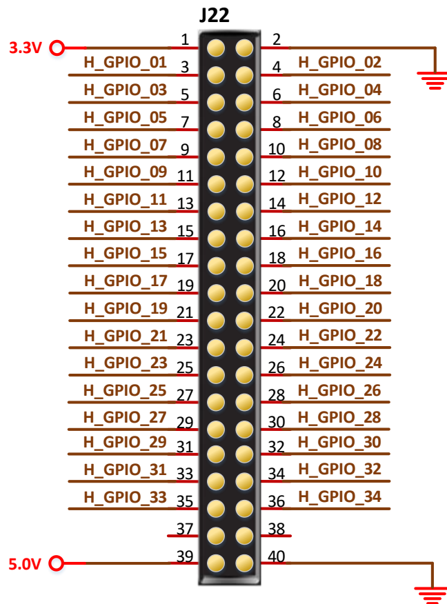
图 3-17 40pin 接口示意图
