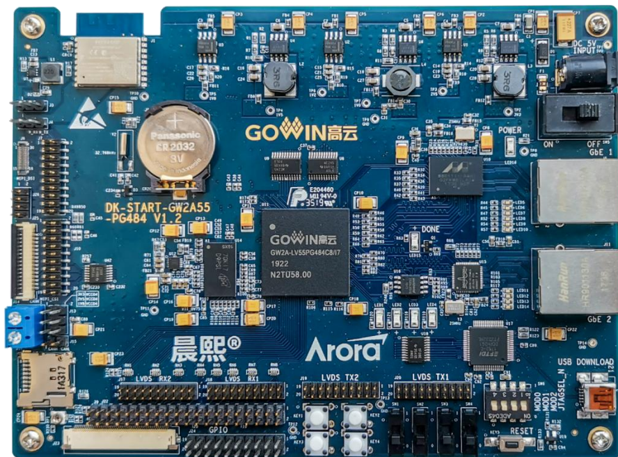
图 2-1 DK_START_GW2A55-PG484_V1.2 开发板
