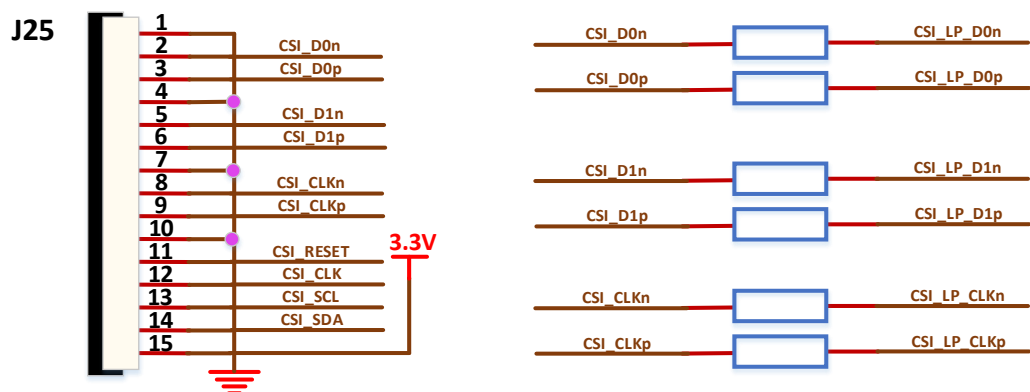
图 3-11 MIPI CSI 模块连接示意图
