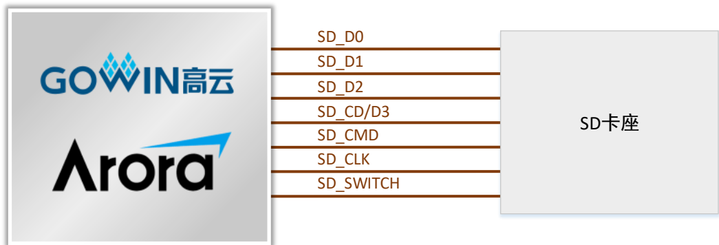
图 3-12 SD 卡模块连接示意图
