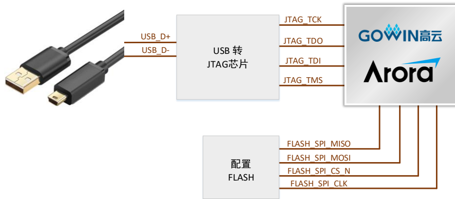
图 3-3 FPGA 下载与配置连接示意图
