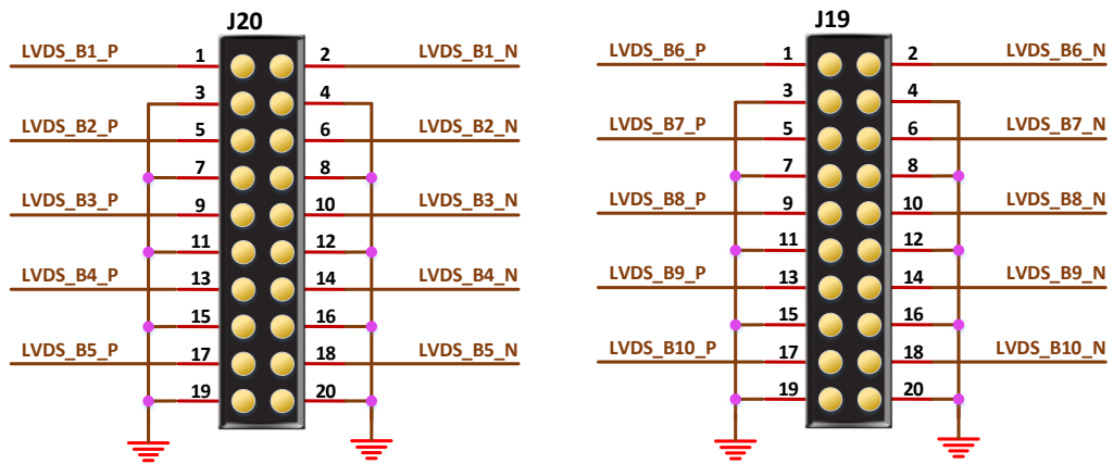
图 3-8 LVDS TX 接口示意图
