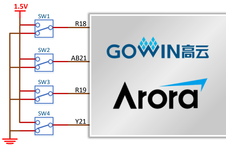
图 3-22 开关电路
