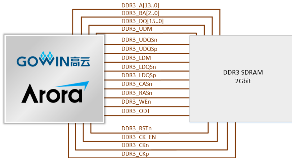
图 3-6 FPGA 与 DDR3 连接示意图
