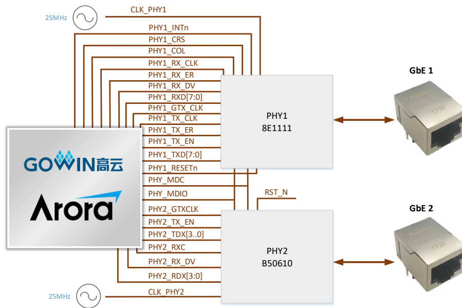
图 3-7 FPGA 与以太网模块连接示意图
