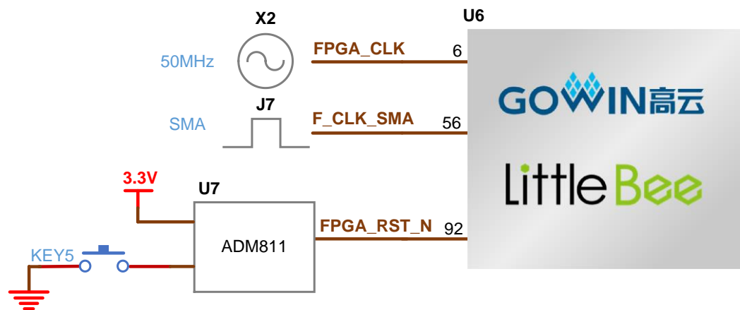
图 3-3 时钟、复位电路
