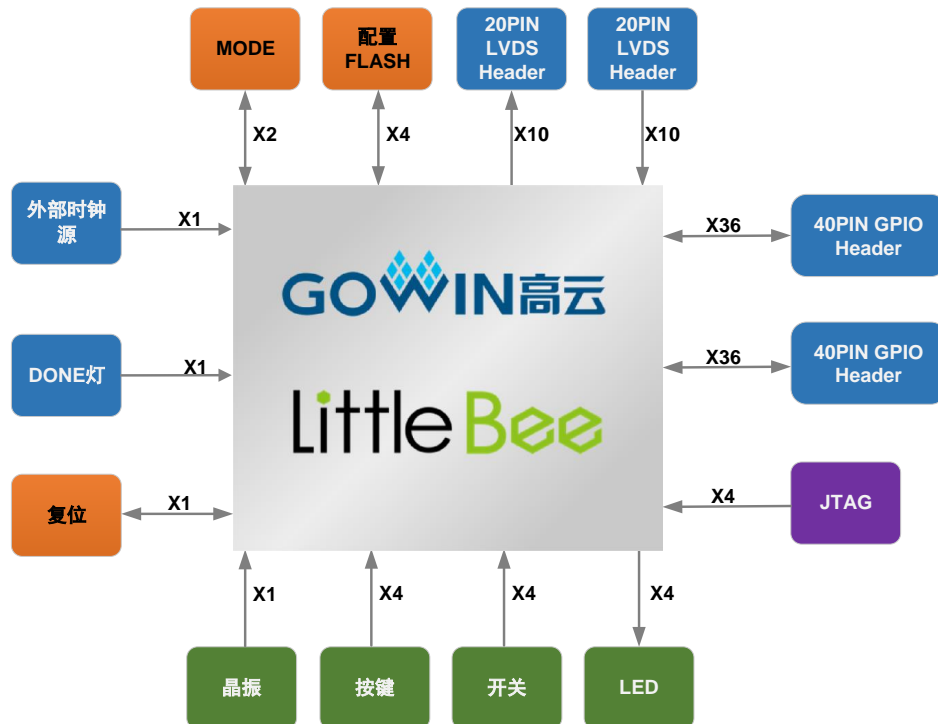
图 2-4 系统框图
