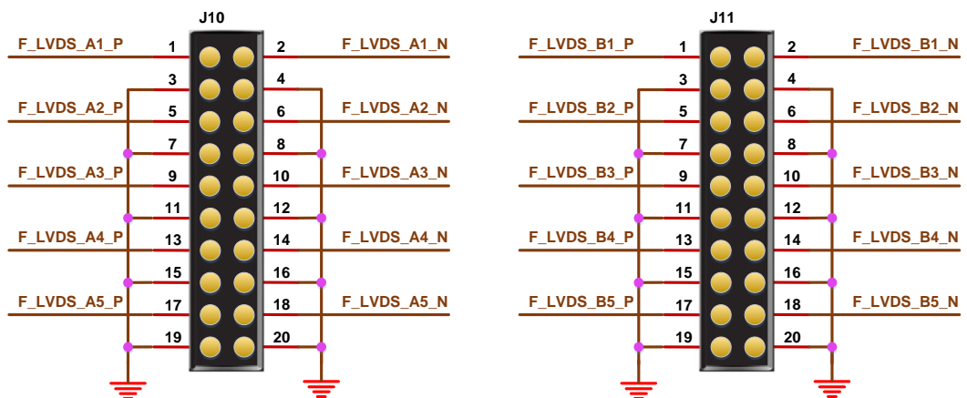
图 3-8 LVDS 电路
