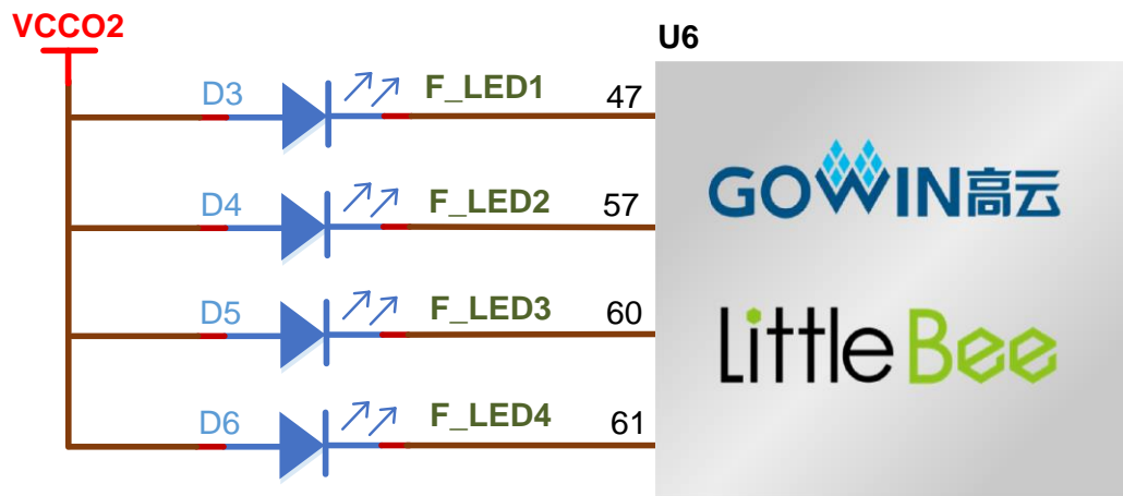
图 3-4 LED 电路
