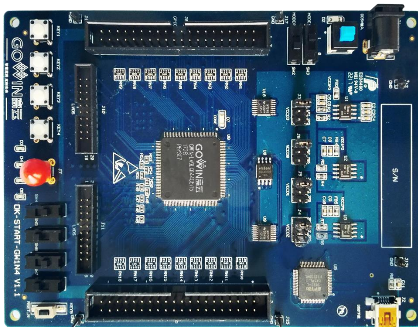
图 2-1 DK_START_GW1N9_V1.1 开发板
