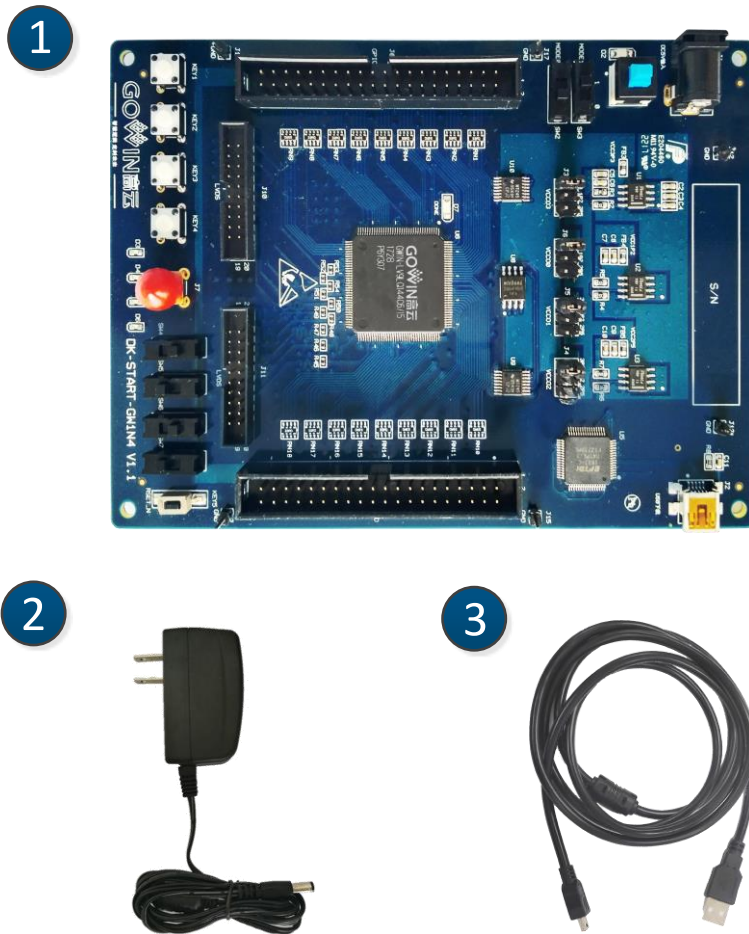
图 2-2 开发板套件
