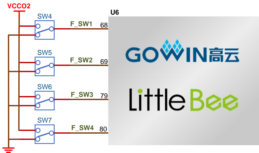
图 3-5 开关电路
