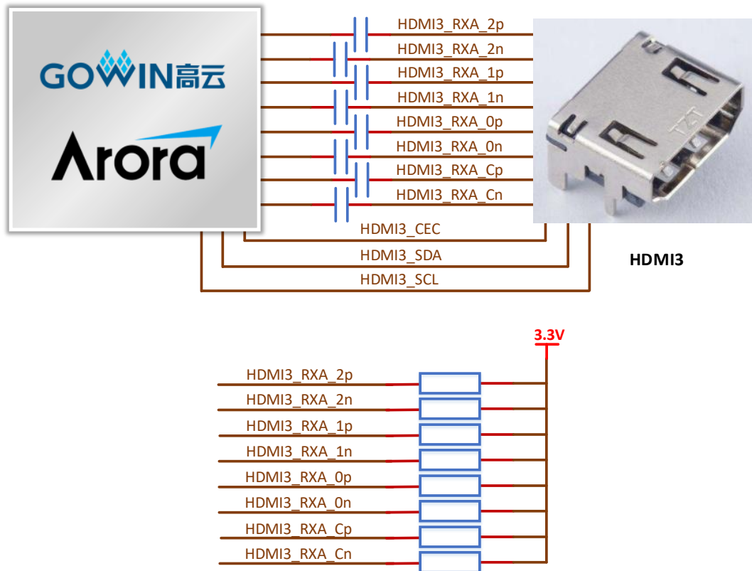
图 3-6 FPGA 与 HDMI3 接口连接示意图
