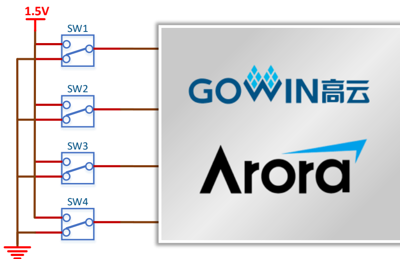
图 3-14 开关电路
