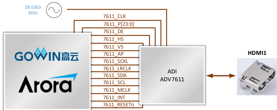
图 3-4 FPGA 与 HDMI1 接口连接示意图
