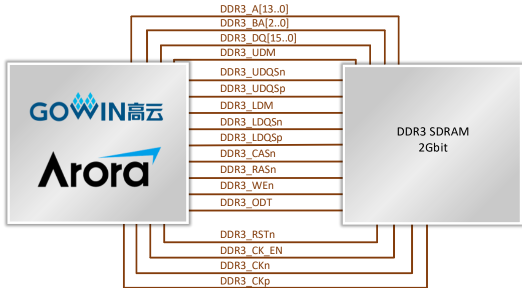
图 3-3 FPGA 与 DDR3 连接示意图
