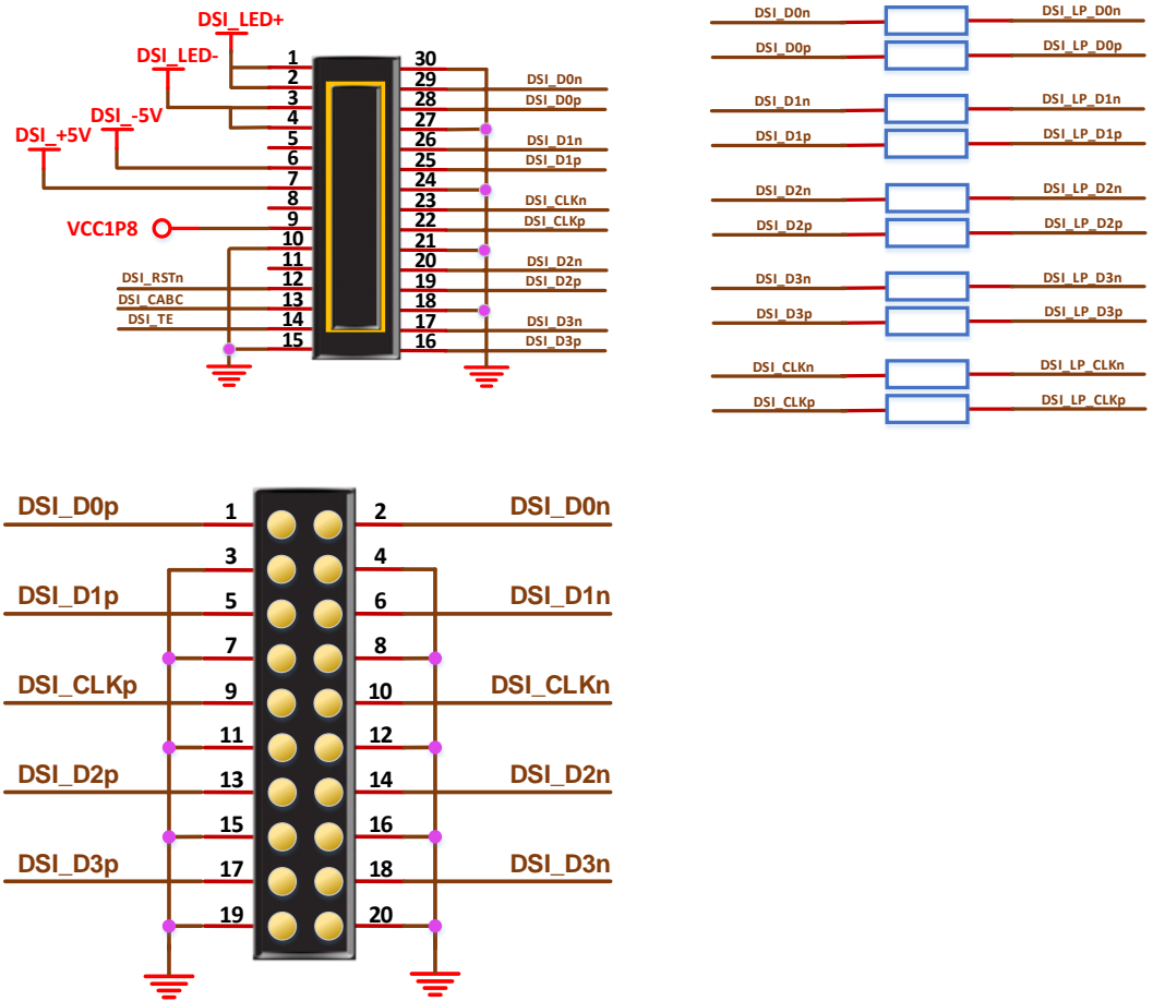
图 3-10 MIPI DSI 模块连接示意图
