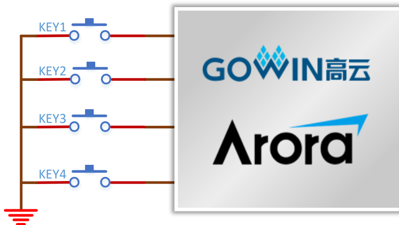
图 3-13 按键电路
