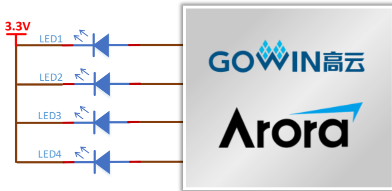
图 3-12 LED 连接示意图
