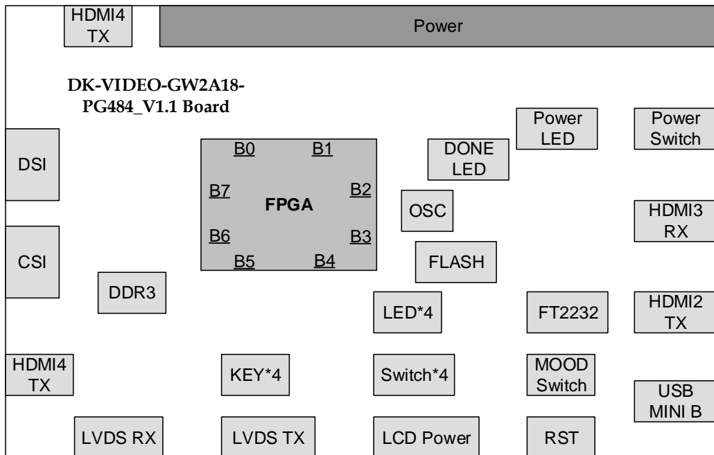
图 2-2 系统框图
