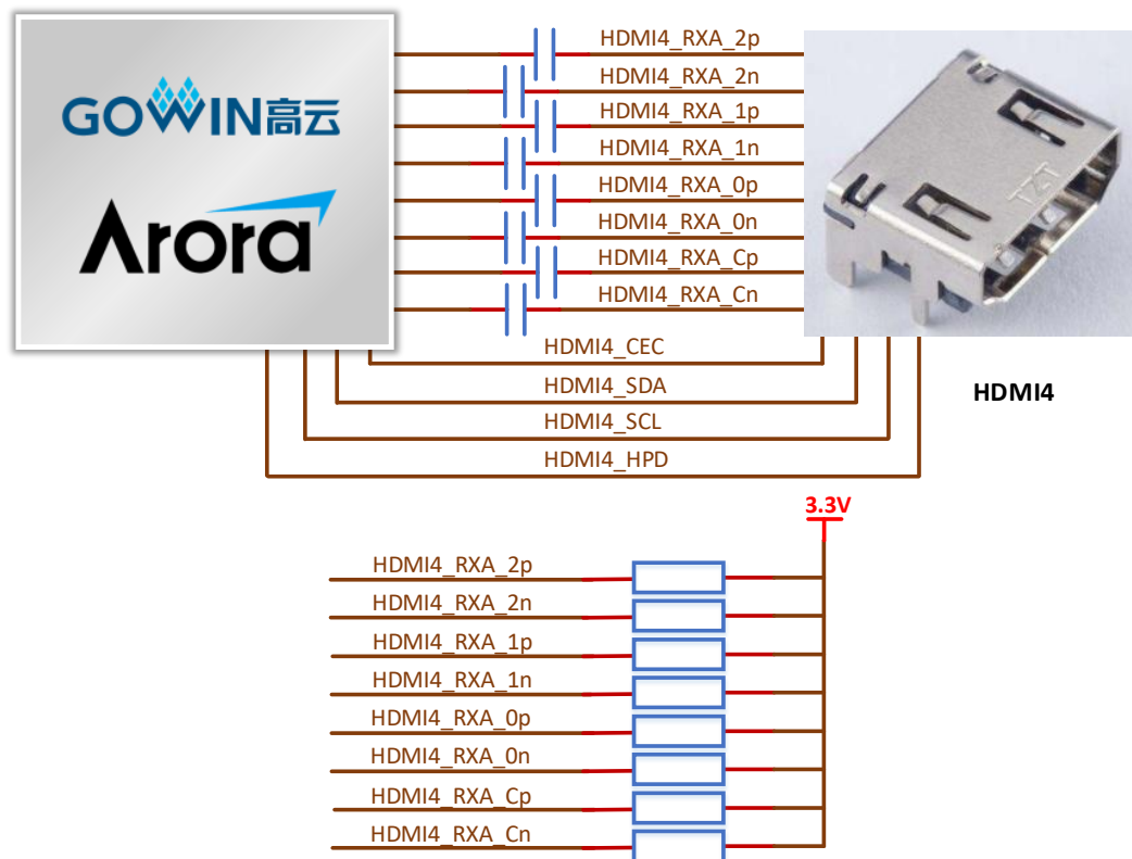
图 3-7 FPGA 与 HDMI4 接口连接示意图
