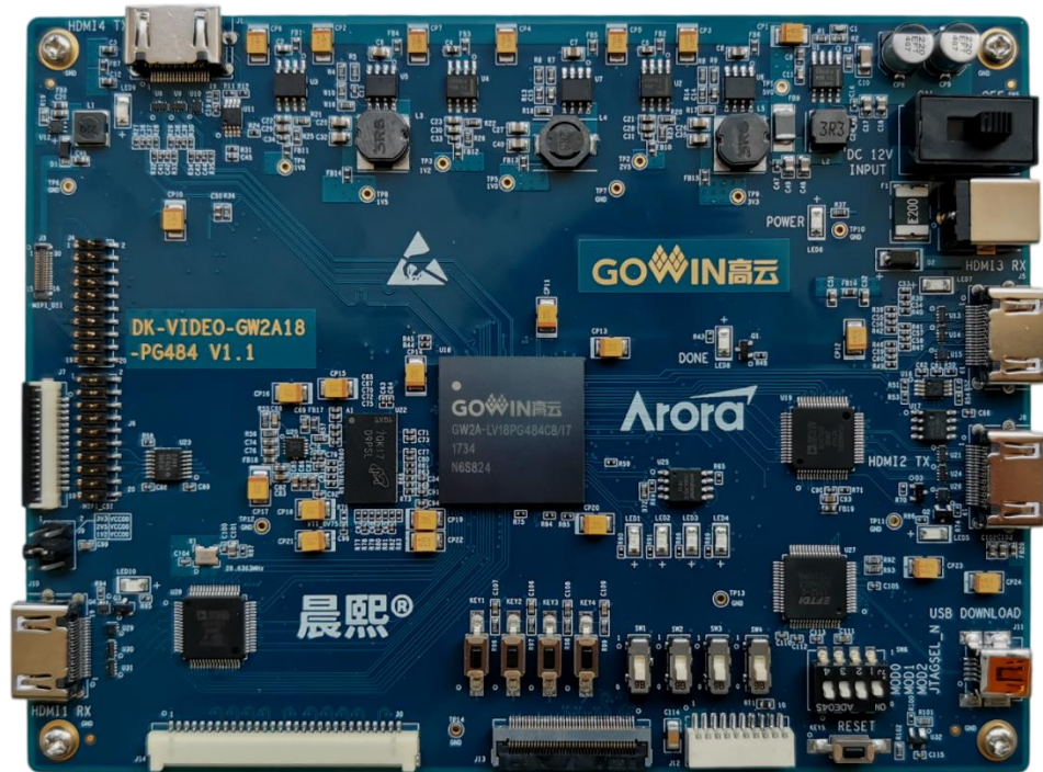
图 2-1 DK-VIDEO-GW2A18-PG484_V1.1 开发板
