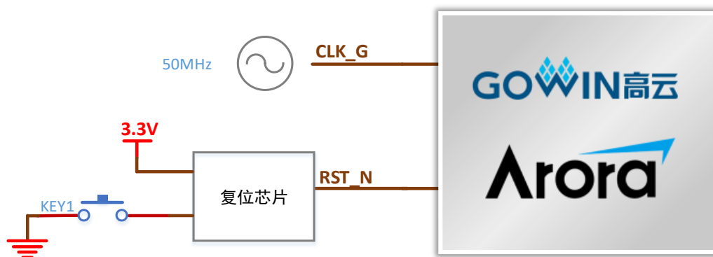
图 3-2 时钟、复位连接示意图
