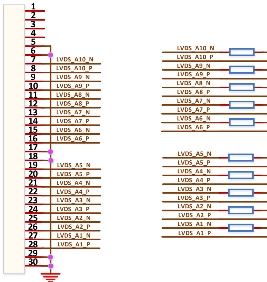
图 3-9 LVDS RX 接口示意图
