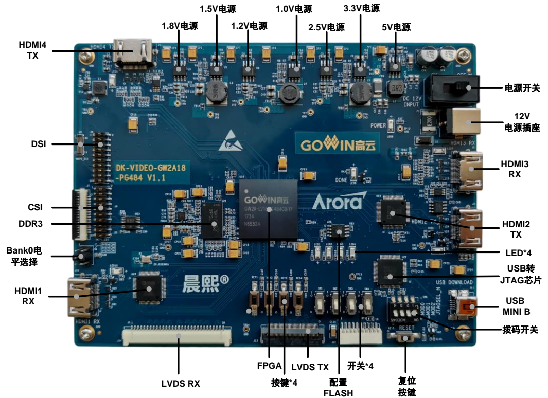
图 2-1 开发板 PCB 组件说明
