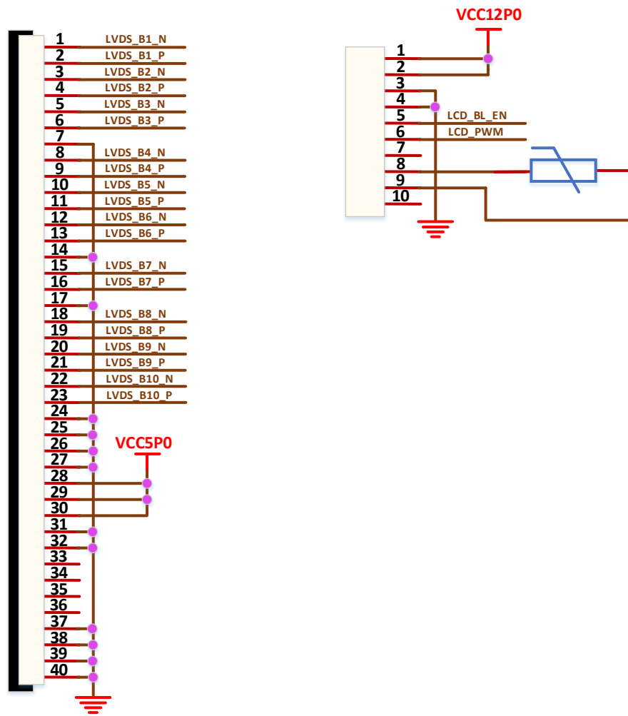
图 3-8 LVDS TX 接口示意图
