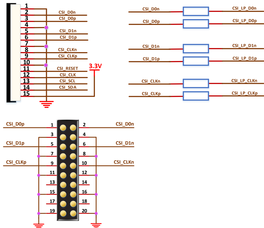
图 3-11 MIPI CSI 模块连接示意图
