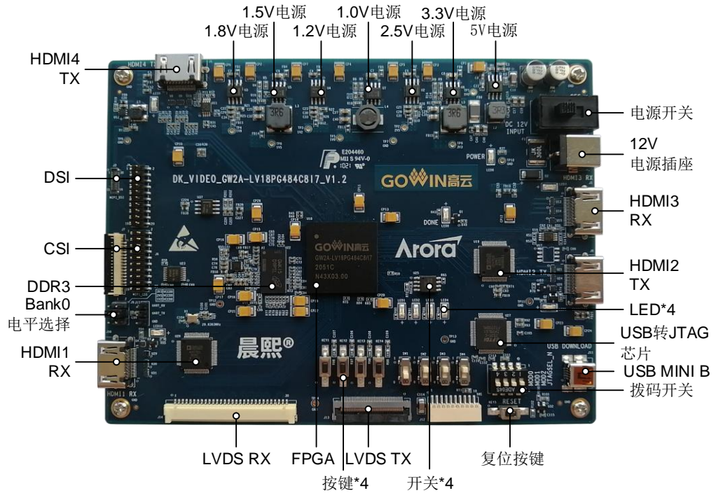
图 2-1 开发板 PCB 组件说明
