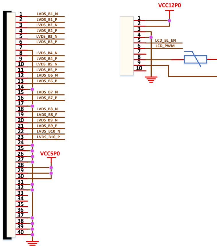
图 3-8 LVDS TX 接口示意图
