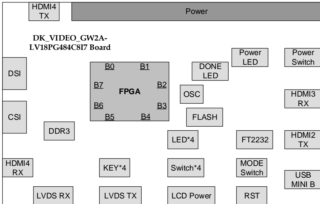
图 2-2 系统框图
