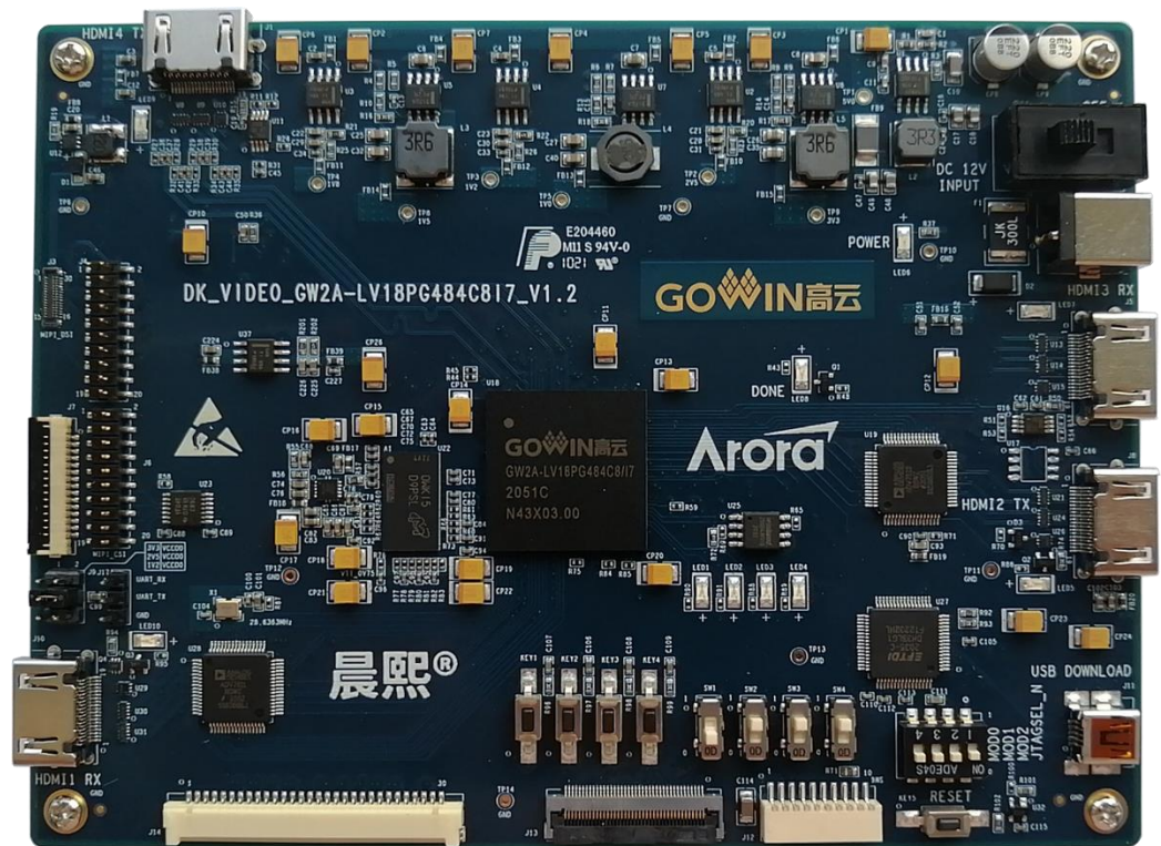
图 2-1 DK_VIDEO_GW2A-LV18PG484C8I7_V1.2 开发板
