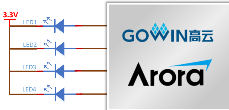
图 3-12 LED 连接示意图
