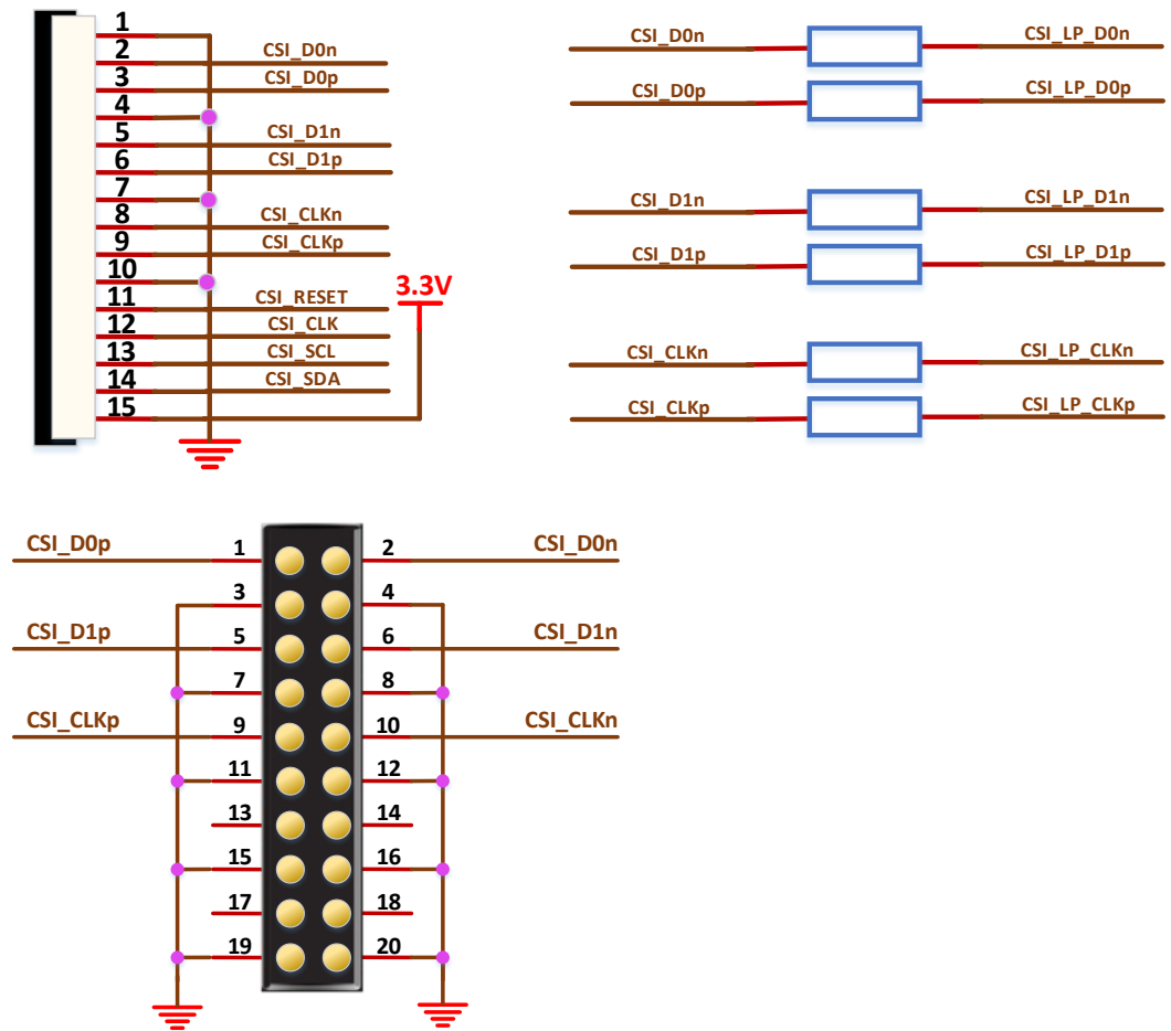
图 3-11 MIPI CSI 模块连接示意图
