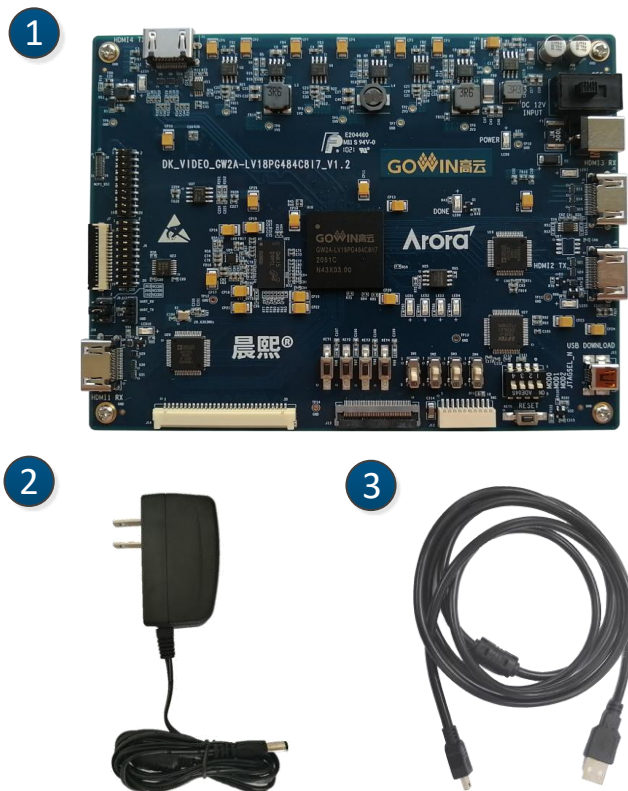
图 2-2 开发板套件
