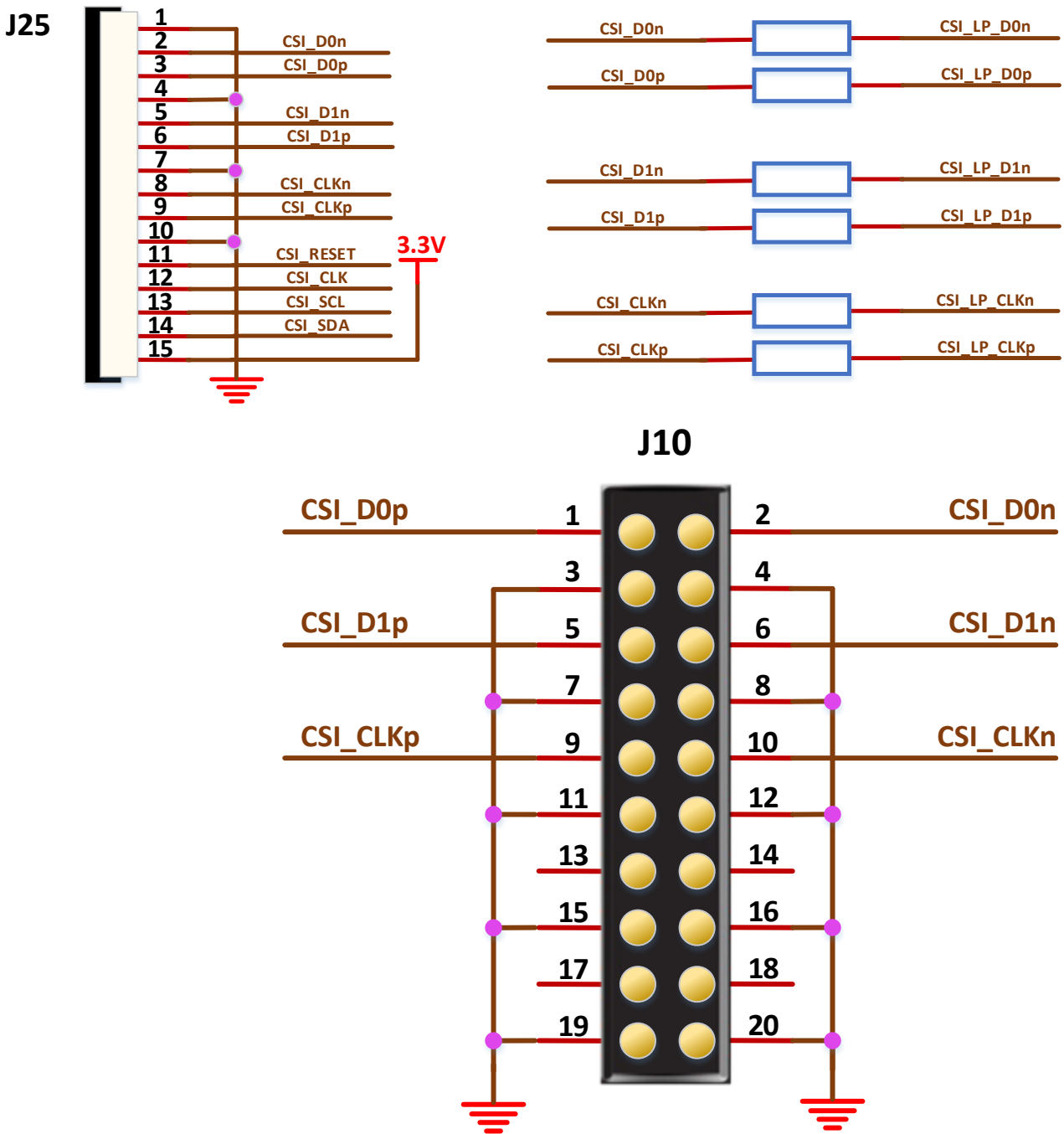
图 3-9 MIPI CSI 模块连接示意图
