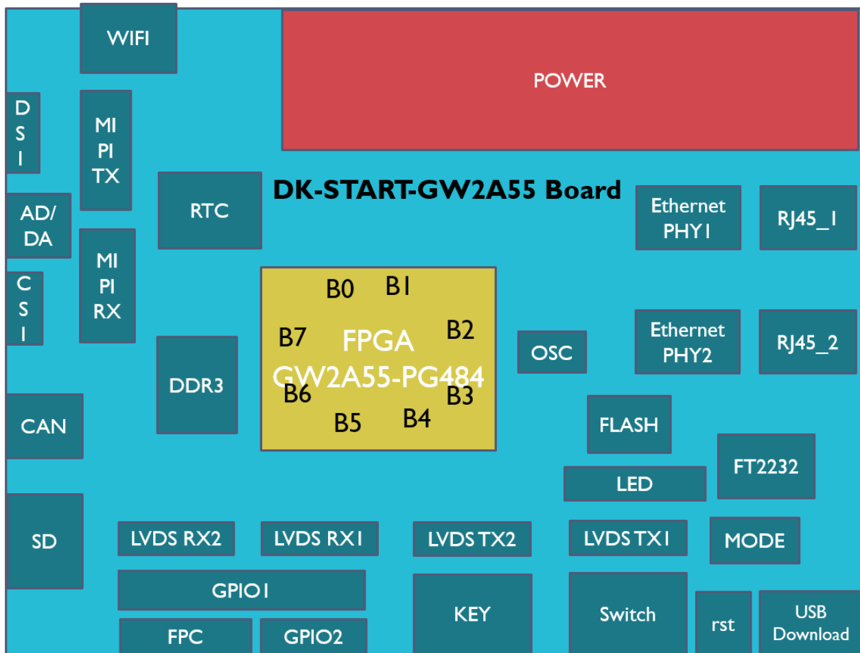
图 2-4 系统框图
