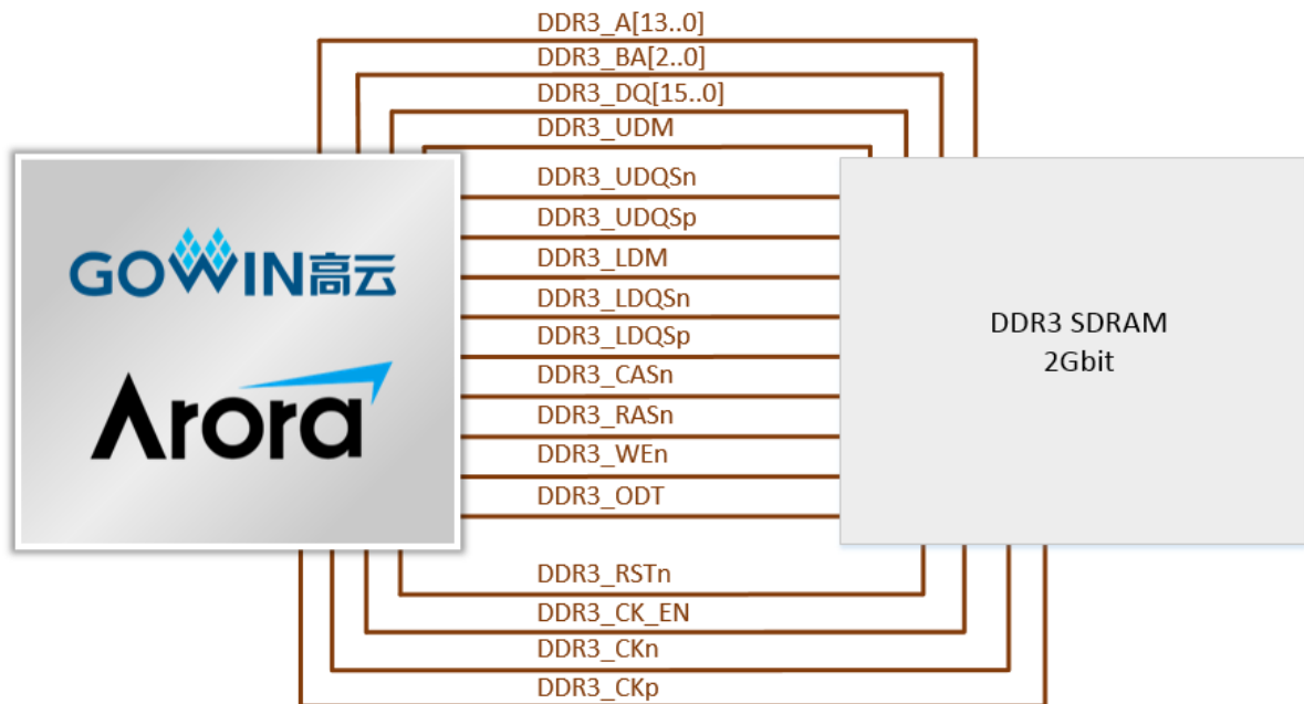
图 3-4 FPGA 与 DDR3 连接示意图
