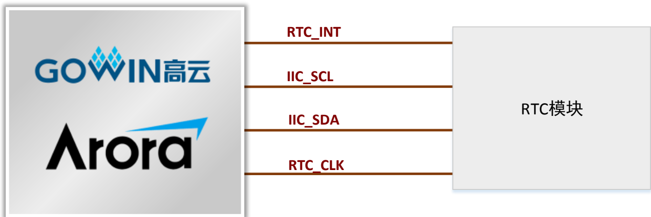
图 3-11 RTC 模块连接示意图
