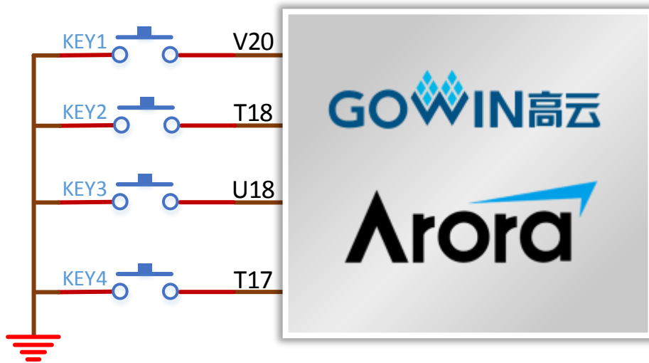
图 3-19 按键电路
