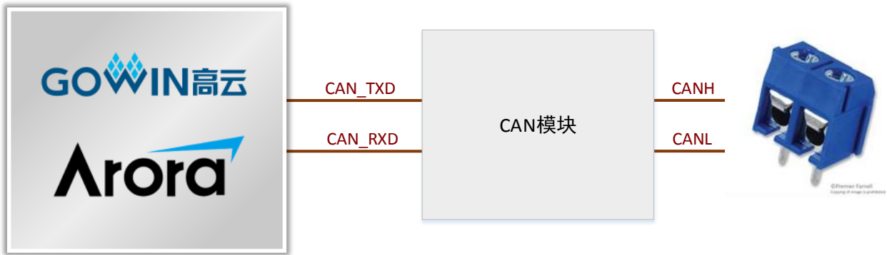
图 3-13 CAN 模块连接示意图
