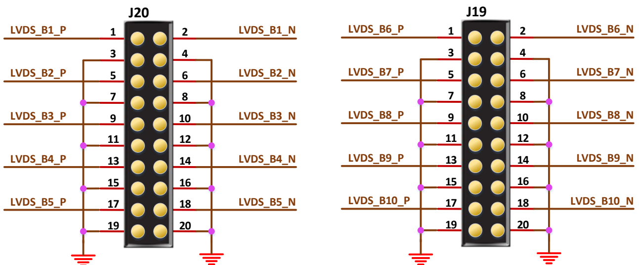
图 3-6 LVDS TX 接口示意图
