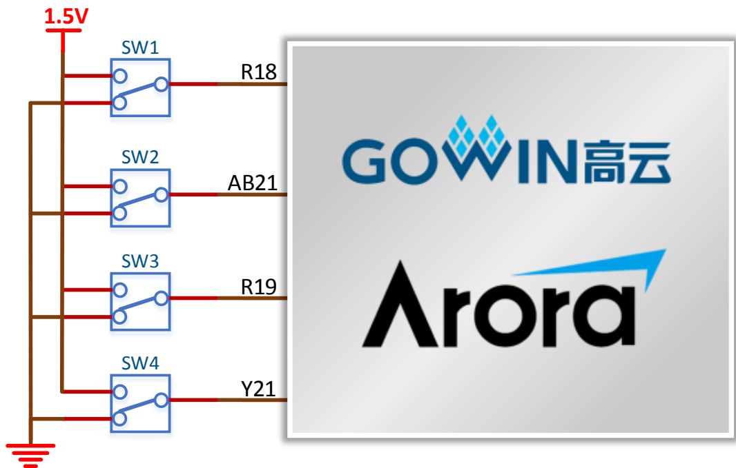
图 3-20 开关电路
