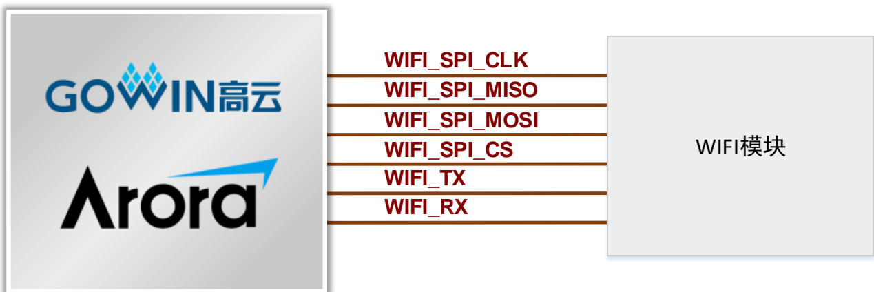
图 3-14 WIFI 模块连接示意图
