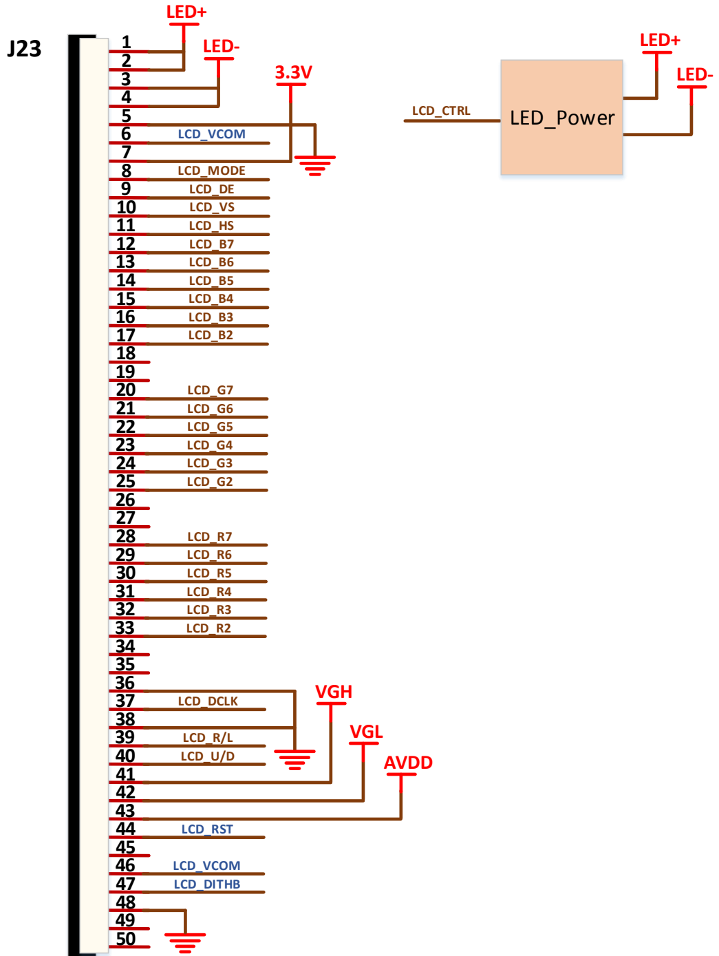
图 3-17 50pin FPC 接口示意图
