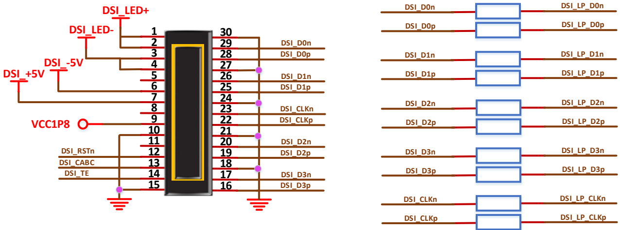
图 3-8 MIPI DSI 模块连接示意图
