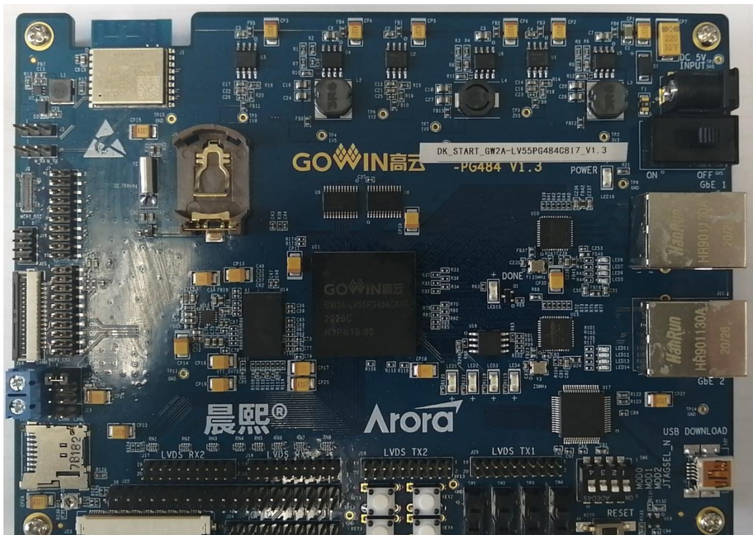
图 2-1 DK_START_GW2A-LV55PG484C8I7_V1.3 开发板
