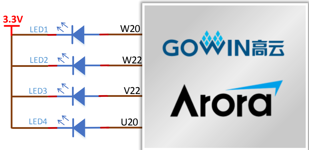
图 3-18 LED 连接示意图
