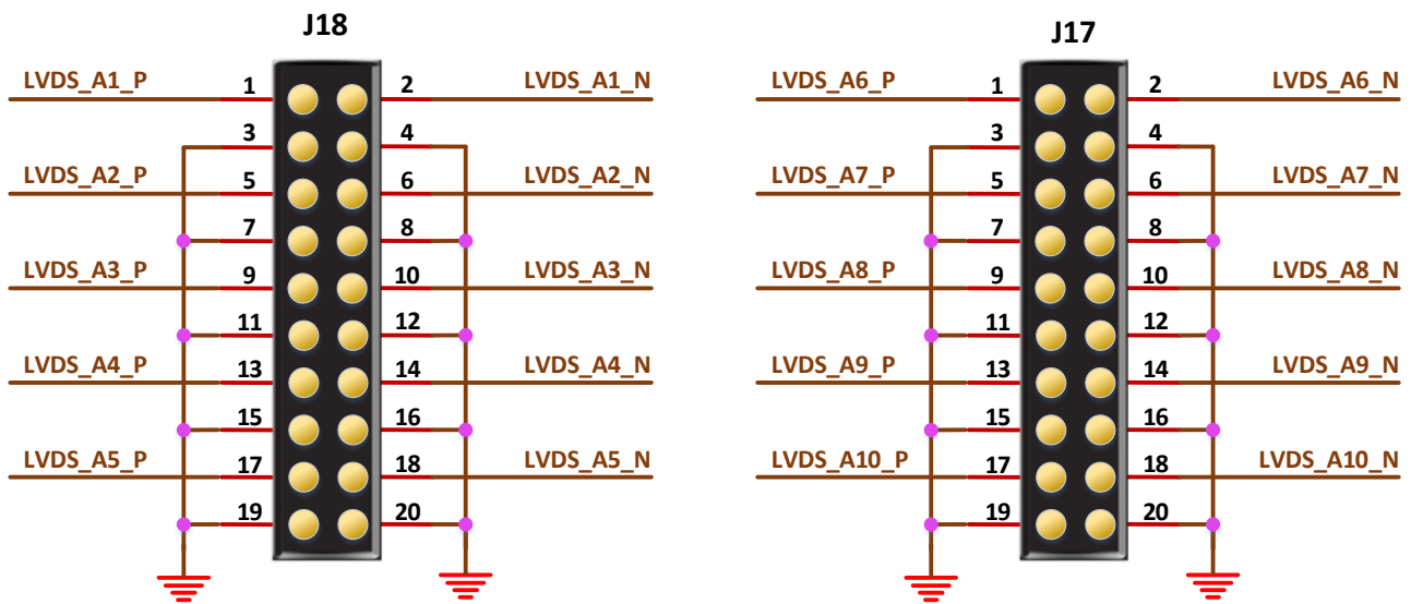
图 3-7 LVDS RX 接口示意图
