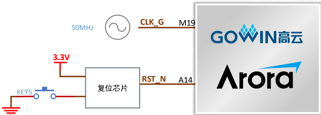
图 3-3 时钟、复位连接示意图
