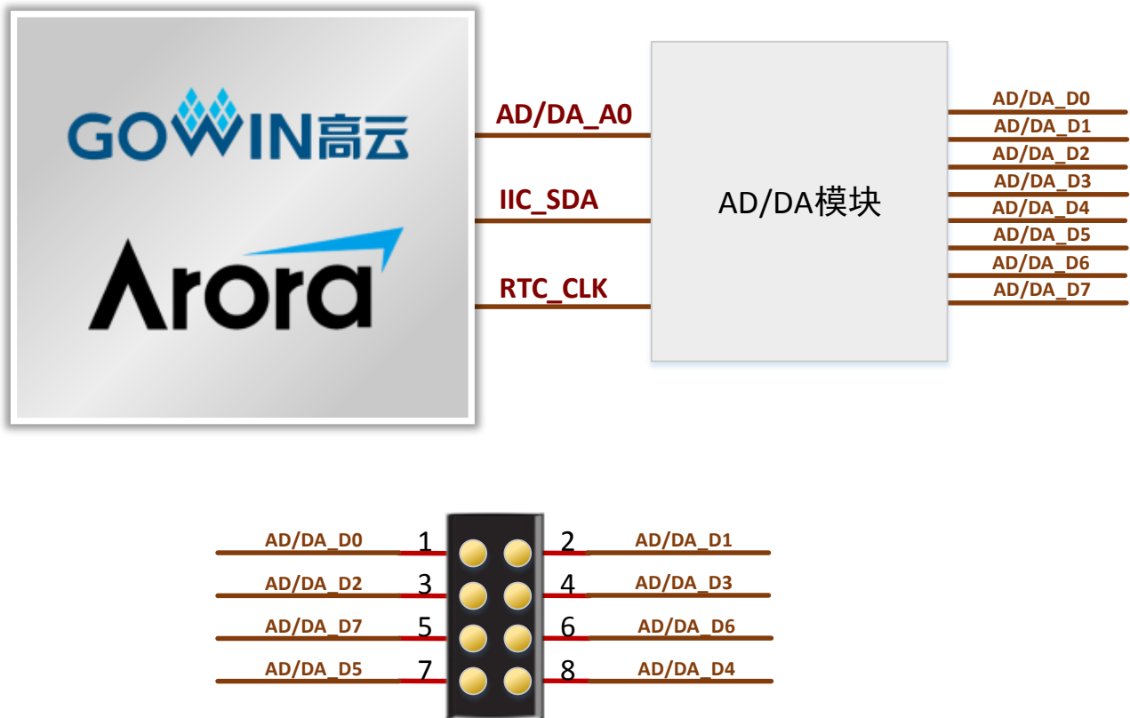
图 3-12 AD/DA 模块连接示意图
