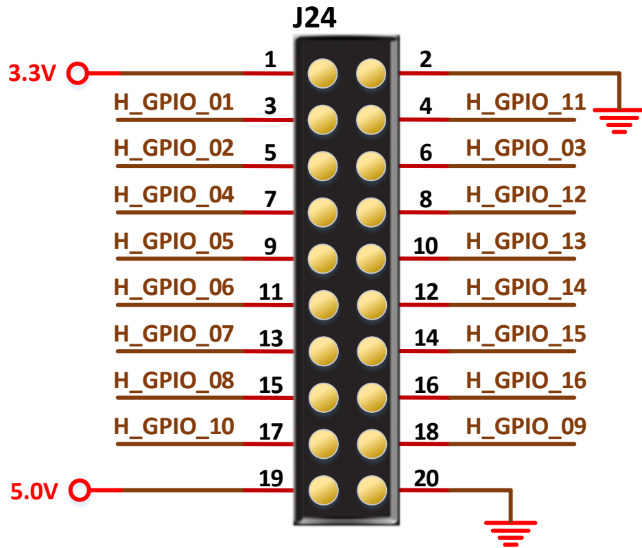
图 3-16 20pin 接口示意图
