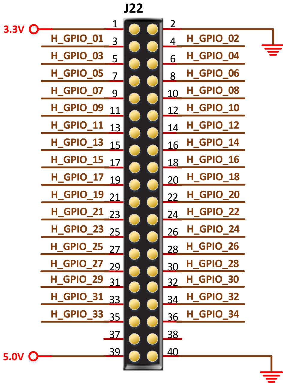
图 3-15 40pin 接口示意图
