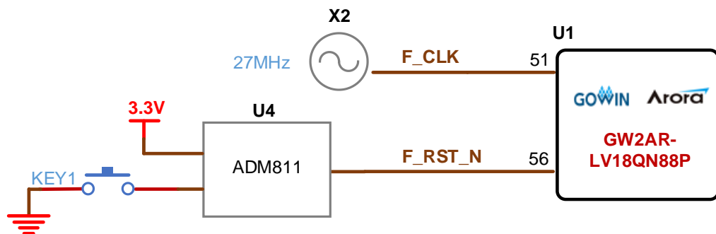
图 3-3 时钟、复位电路
