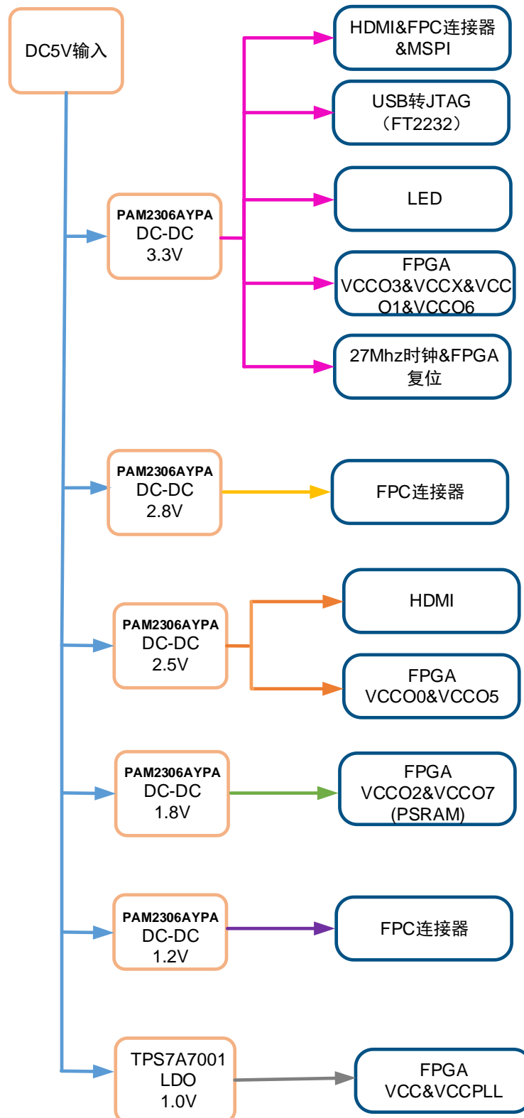
图 3-2 电源系统分配示意图
