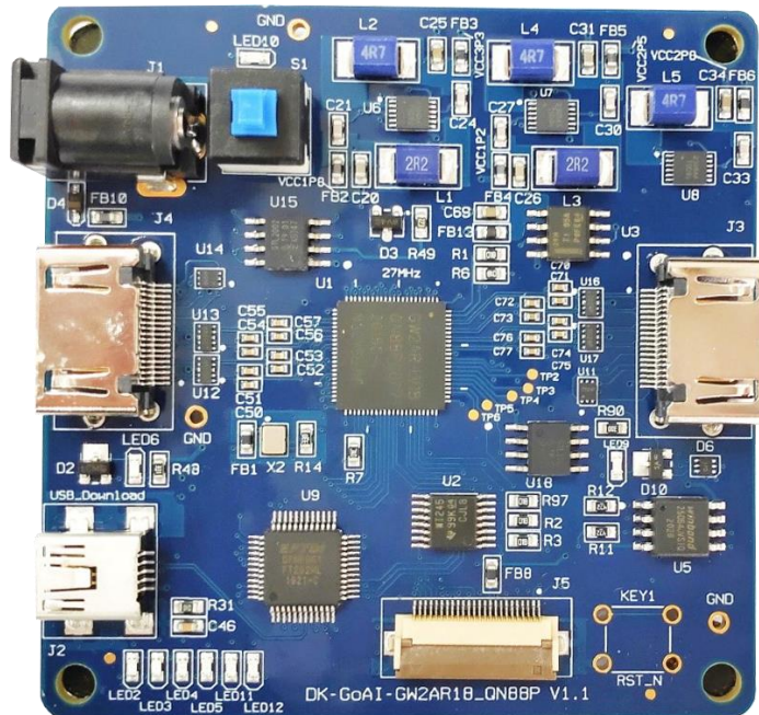
图 2-1 DK-GoAI-GW2AR18QN88P_V1.1 开发板
