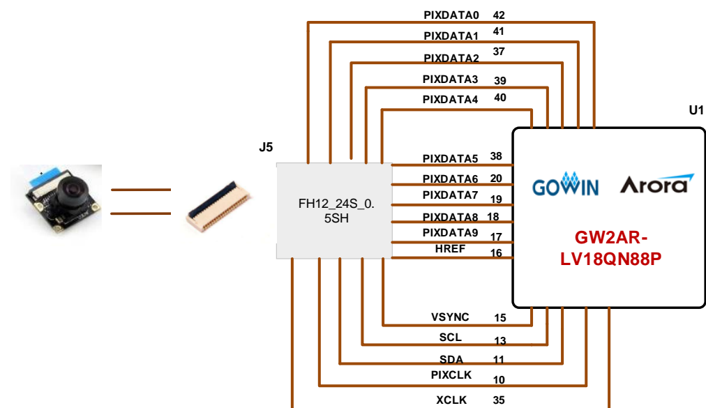
图 3-5 FPC 电路
