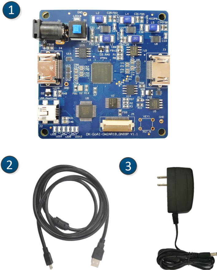
图 2-2 开发板套件
