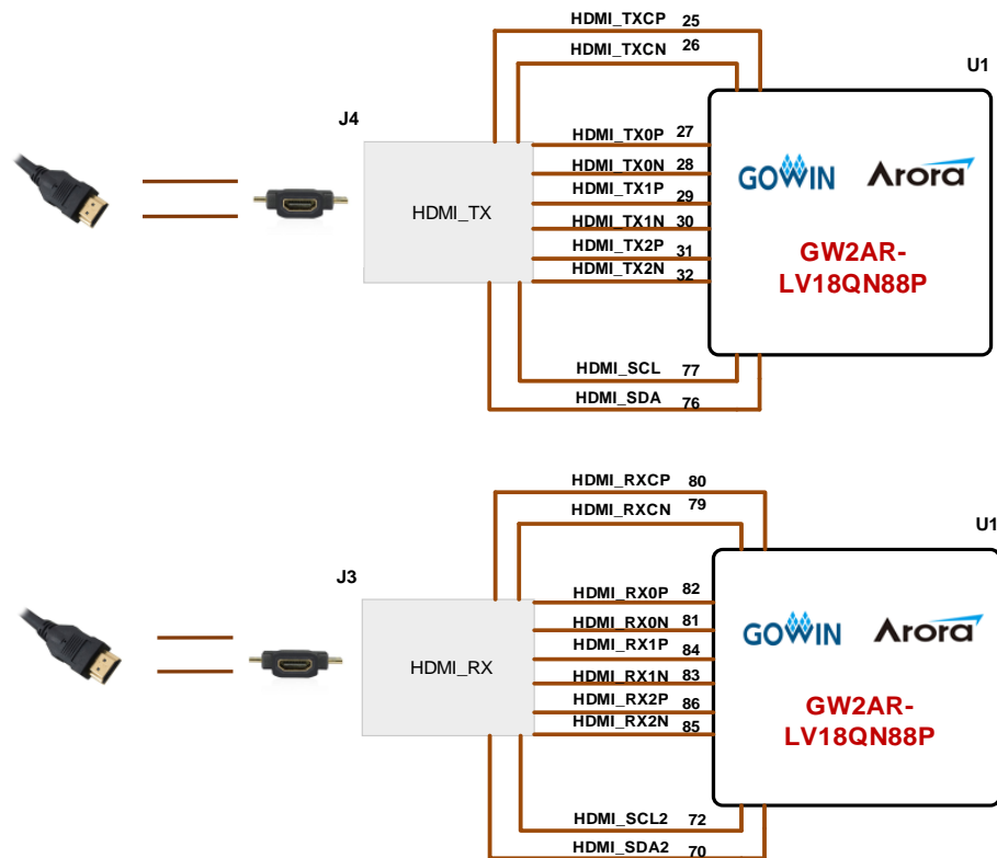
图 3-6 HDMI 连接示意图
