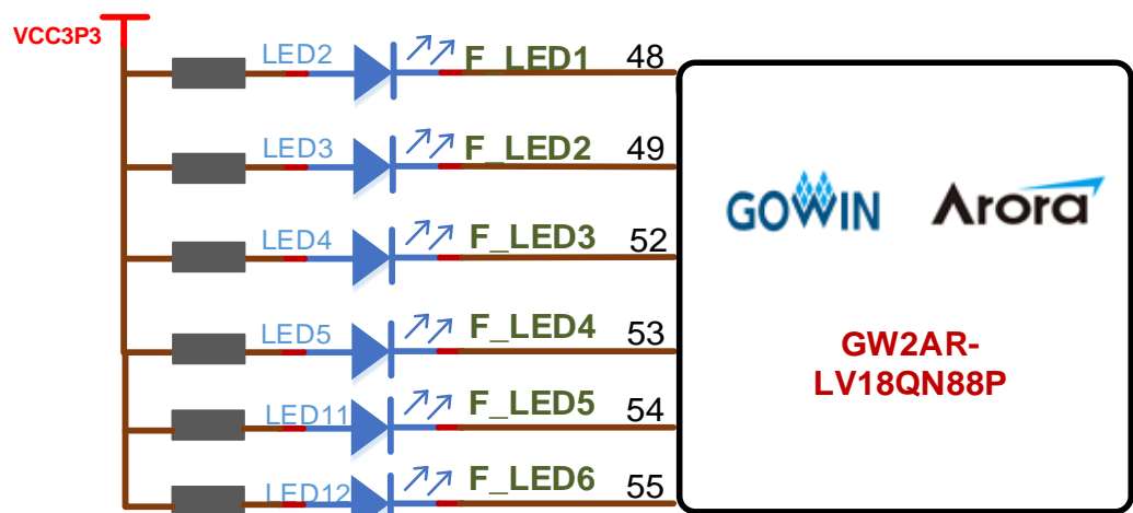
图 3-4 LED 电路
