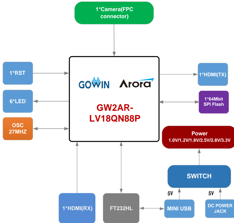
图 2-4 系统框图
