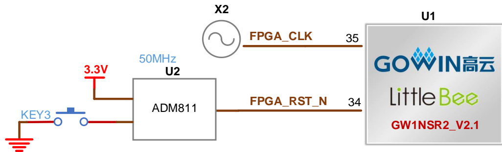
图 3-5 时钟、复位电路
