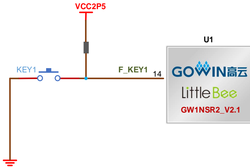
图 3-7 按键电路
