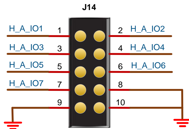
图 3-8 GPIO 电路
