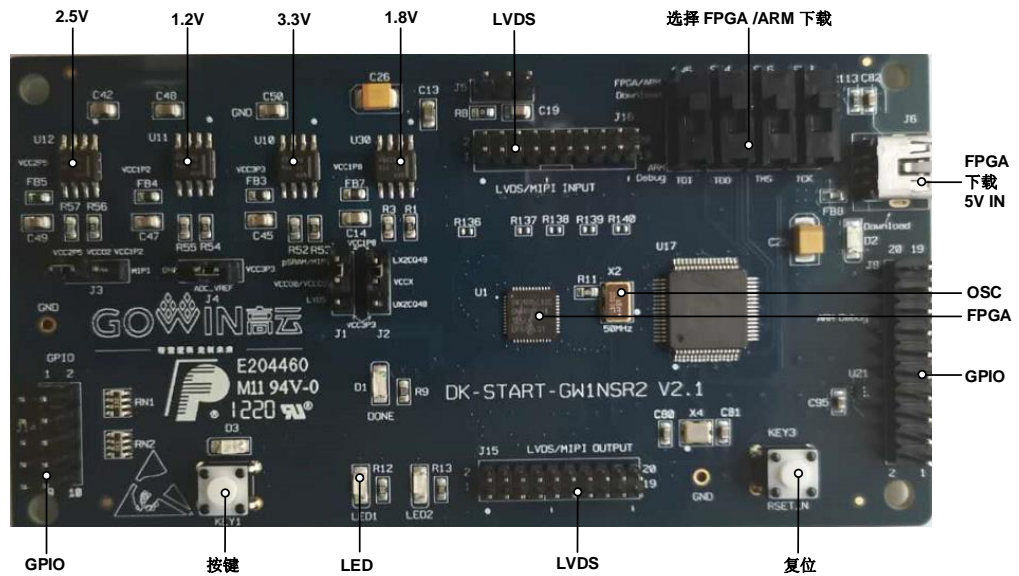
图 2-3 开发板 PCB 组件说明
