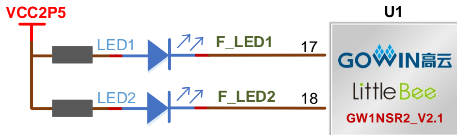
图 3-6 LED 电路
