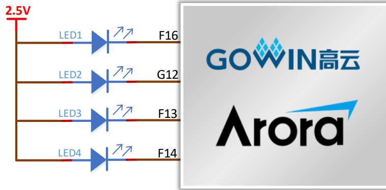
图 3-11 LED 连接示意图
