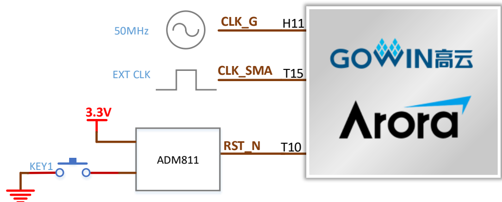
图 3-3 时钟、复位连接示意图
