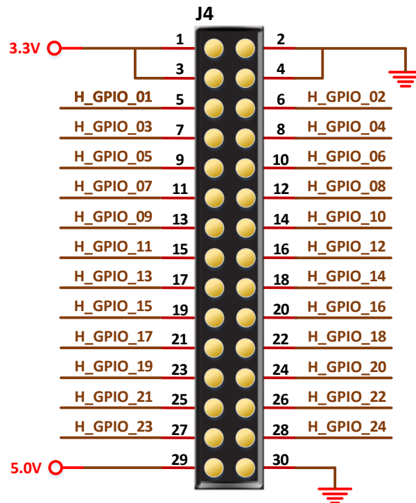
图 3-10 30pin 接口示意图
