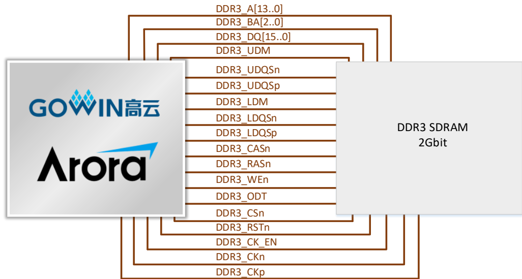
图 3-4 FPGA 与 DDR3 连接示意图
