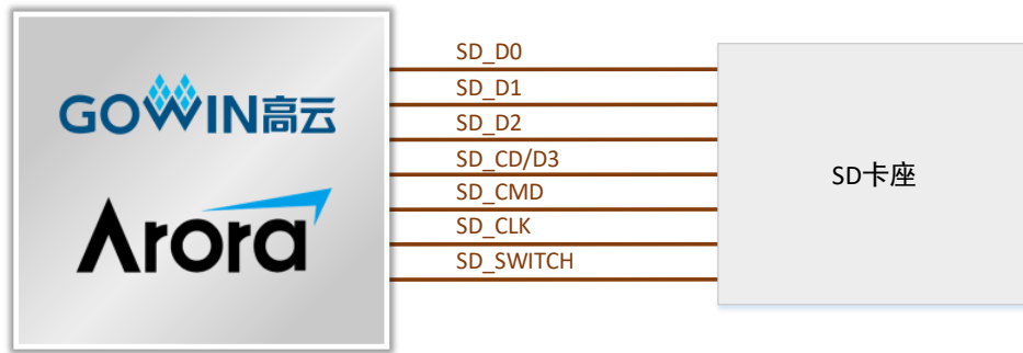
图 3-8 SD 卡模块连接示意图
