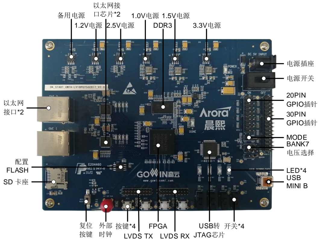
图 2-1 开发板 PCB 组件说明
