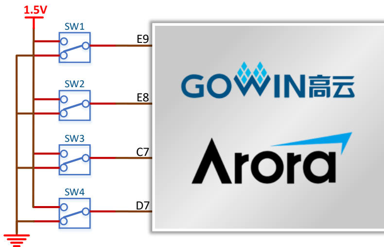
图 3-13 开关模块电路
