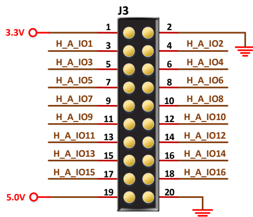
图 3-9 20pin 接口示意图
