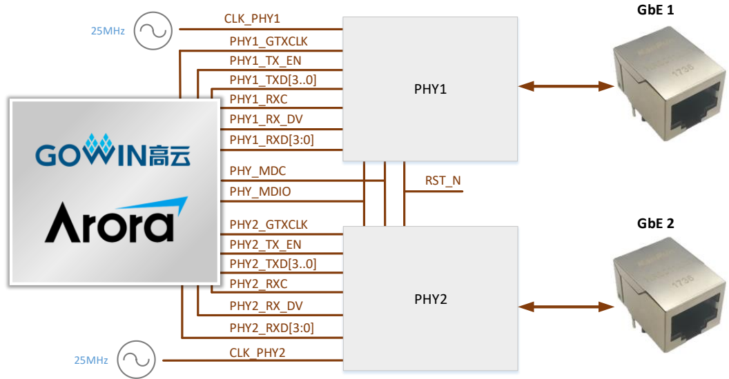
图 3-5 FPGA 与以太网模块连接示意图
