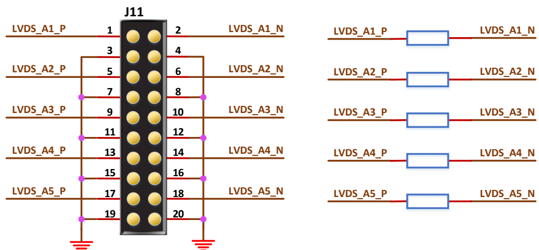
图 3-7 LVDS RX 接口示意图
