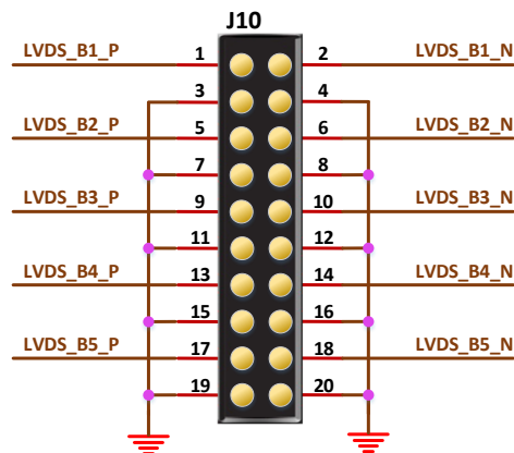
图 3-6 LVDS TX 接口示意图
