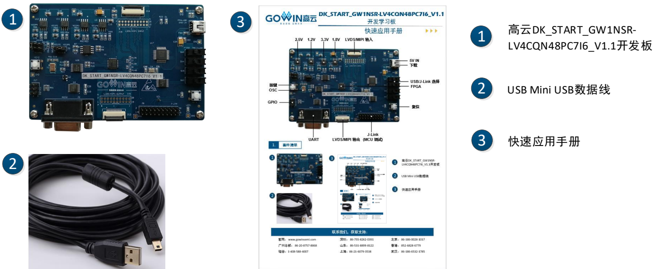
图 2-2 开发板套件
