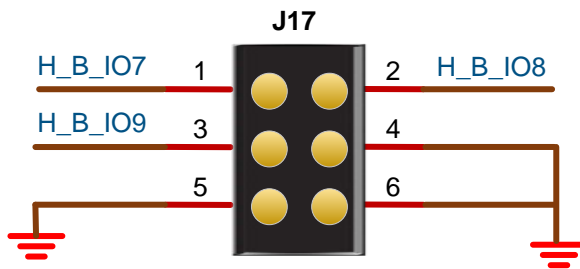
图 3-7 GPIO 电路
