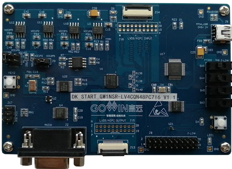
图 2-1 DK_START_GW1NSR-LV4CQN48PC716_V1.1 开发板
