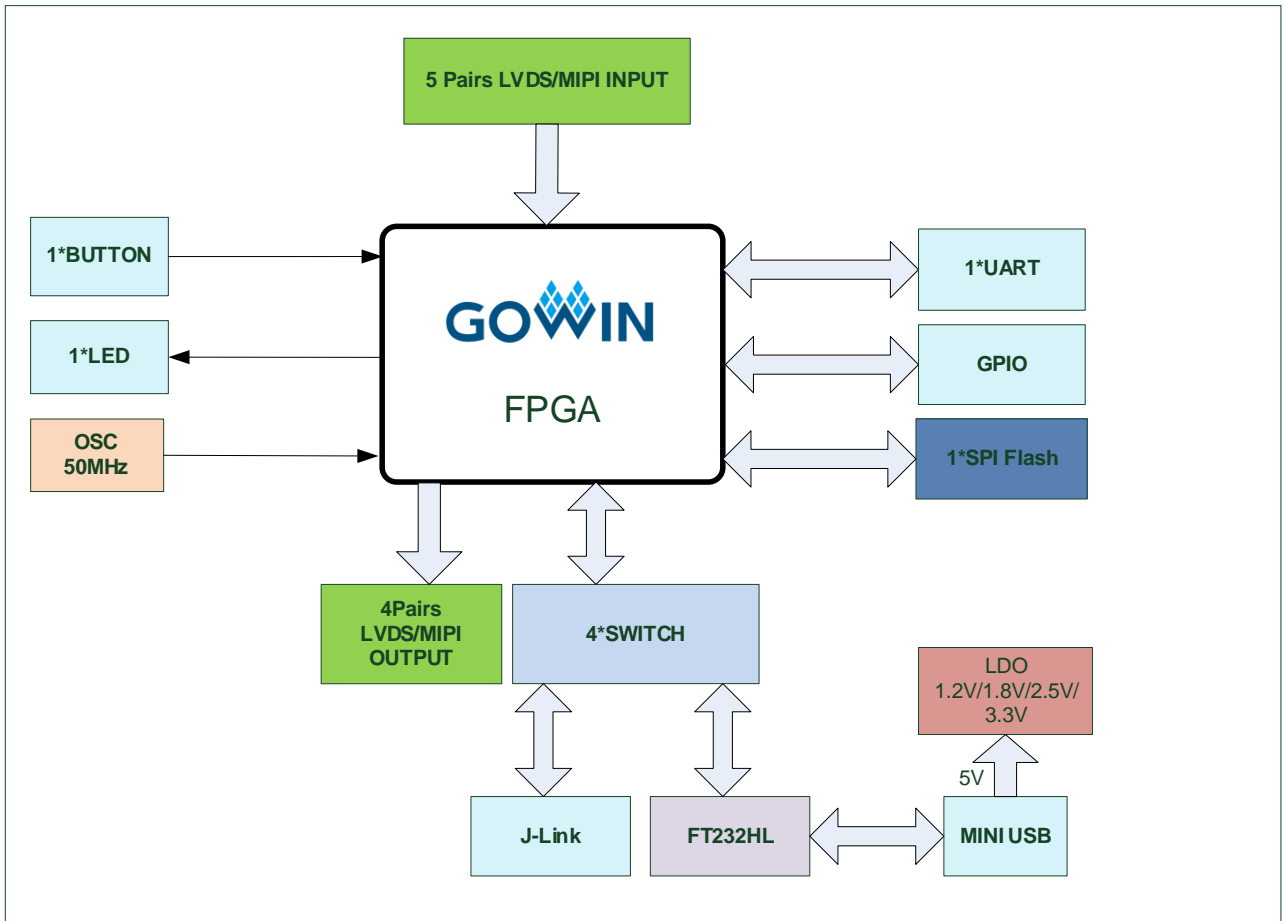
图 2-4 系统框图
