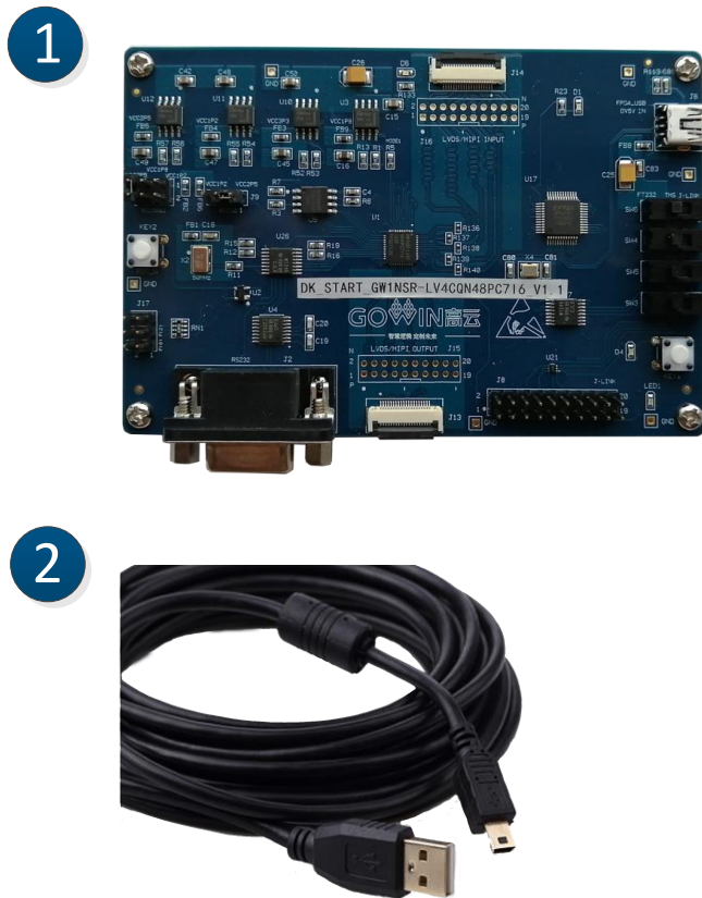
图 2-2 开发板套件
