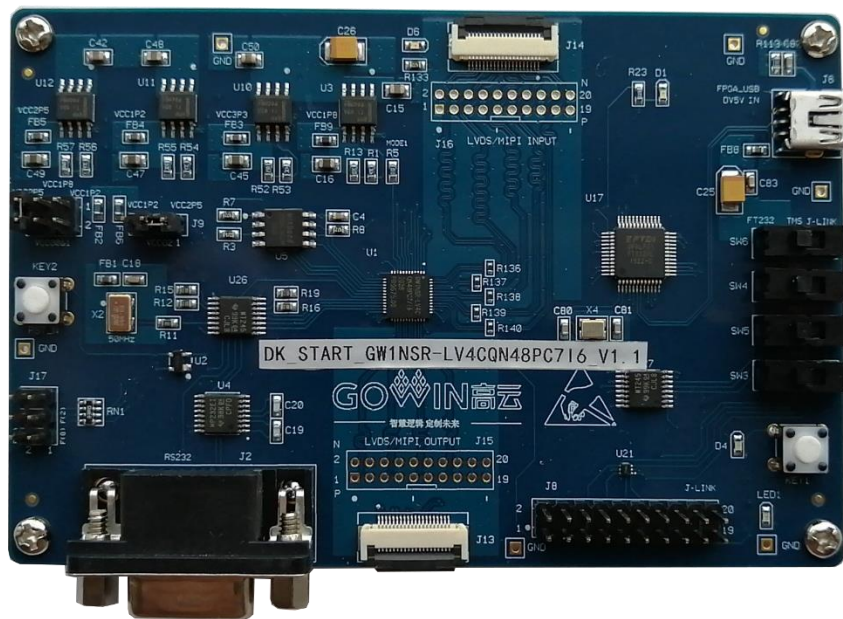
图 2-1 DK_START_GW1NSR-LV4CQN48PC716_V1.1 开发板
