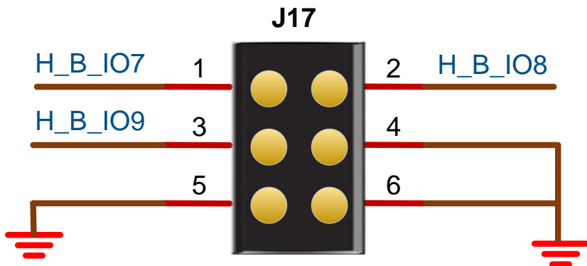
图 3-7 GPIO 电路
