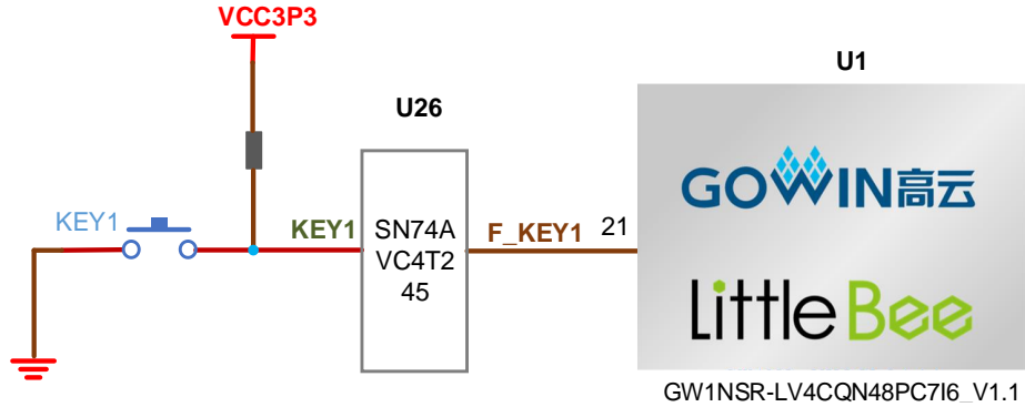
图 3-6 按键电路
