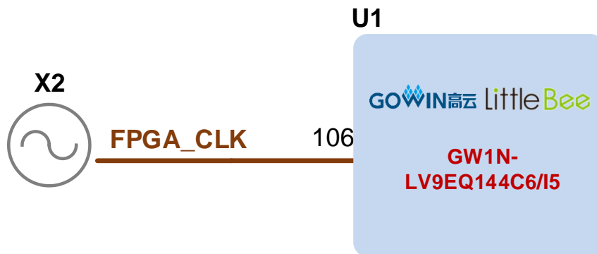
图 3-3 时钟电路
