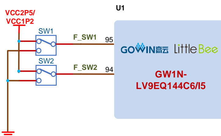
图 3-5 开关电路
