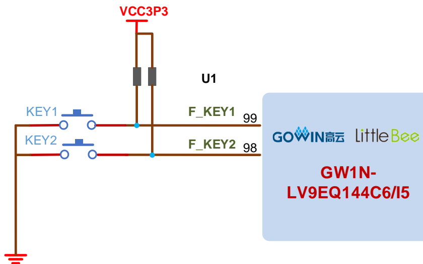
图 3-6 按键电路
