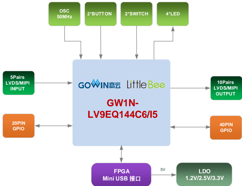
图 2-4 系统框图
