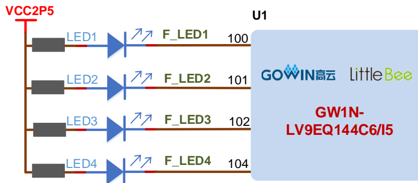
图 3-4 LED 电路
