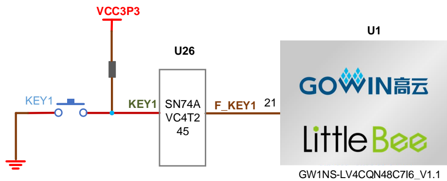
图 3-6 按键电路
