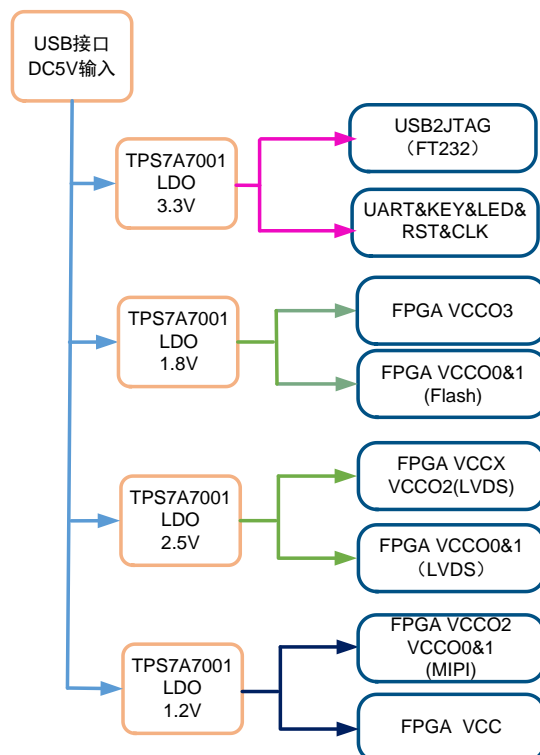
图 3-3 电源系统分配示意图
