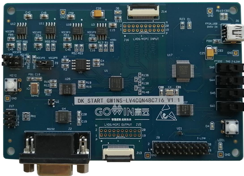
图 2-1 DK_START_GW1NS-LV4CQN48C7I6_V1.1 开发板
