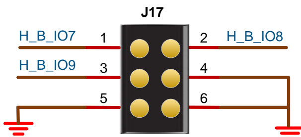
图 3-7 GPIO 电路
