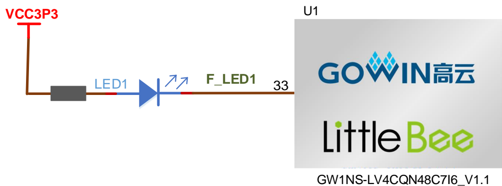
图 3-5 LED 电路
