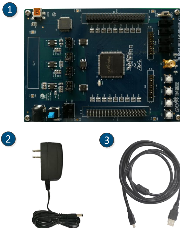
图 2-2 开发板套件
