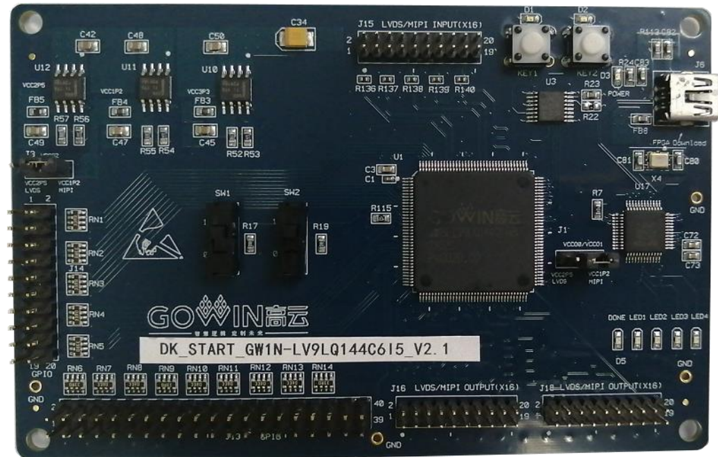
图 2-1 DK_START_GW1N-LV9LQ144C6I5_V2.1 开发板
