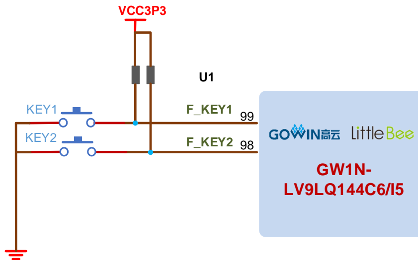
图 3-6 按键电路
