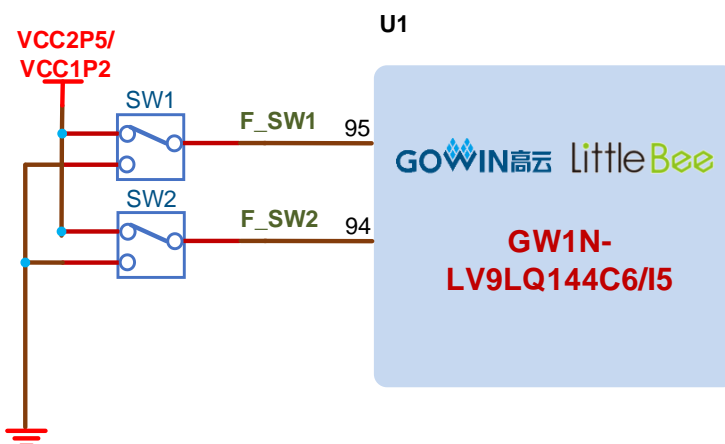
图 3-5 开关电路
