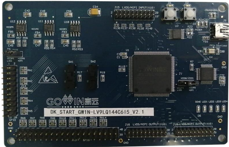
图 2-2 开发板套件
