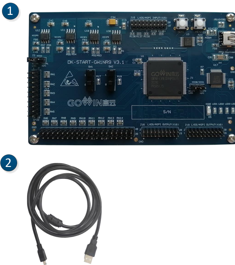
图 2-2 开发板套件
