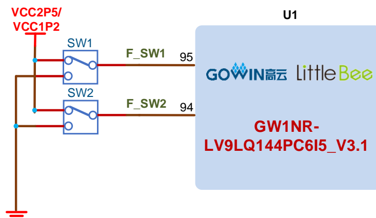
图 3-5 开关电路
