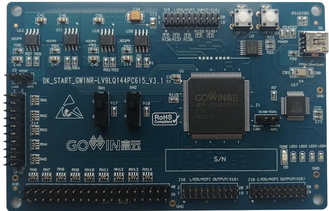
图 2-1 DK_START_GW1NR-LV9LQ144PC6I5_V3.1 开发板
