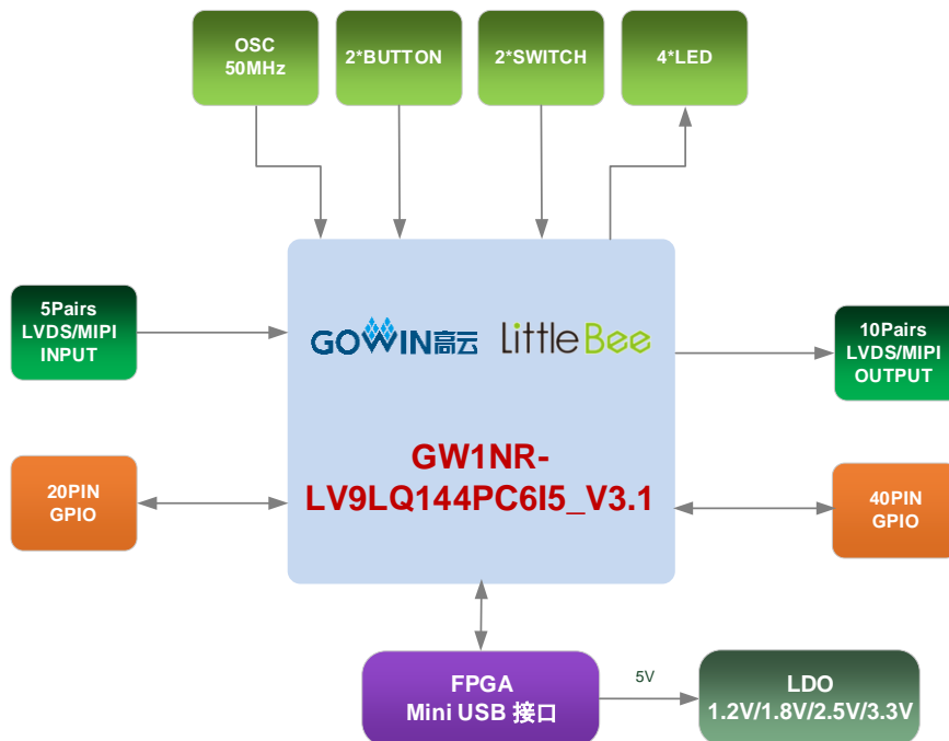
图 2-4 系统框图
