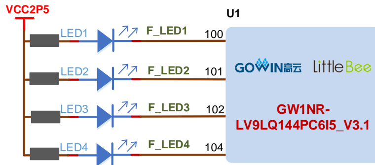
图 3-4 LED 电路
