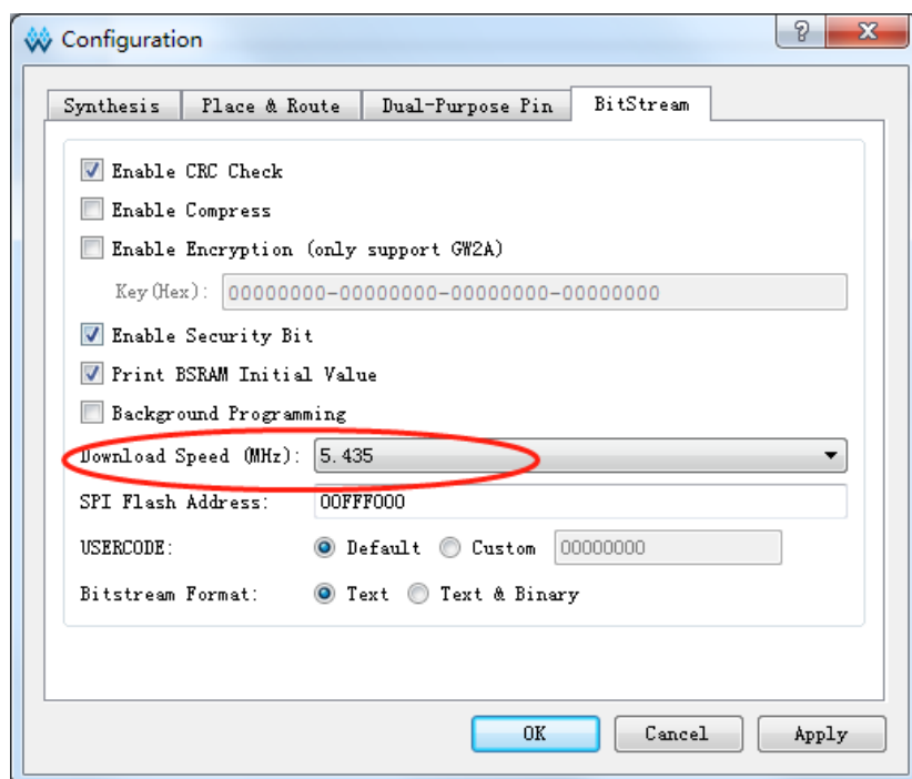
图 4-1 Download Speed 配置
