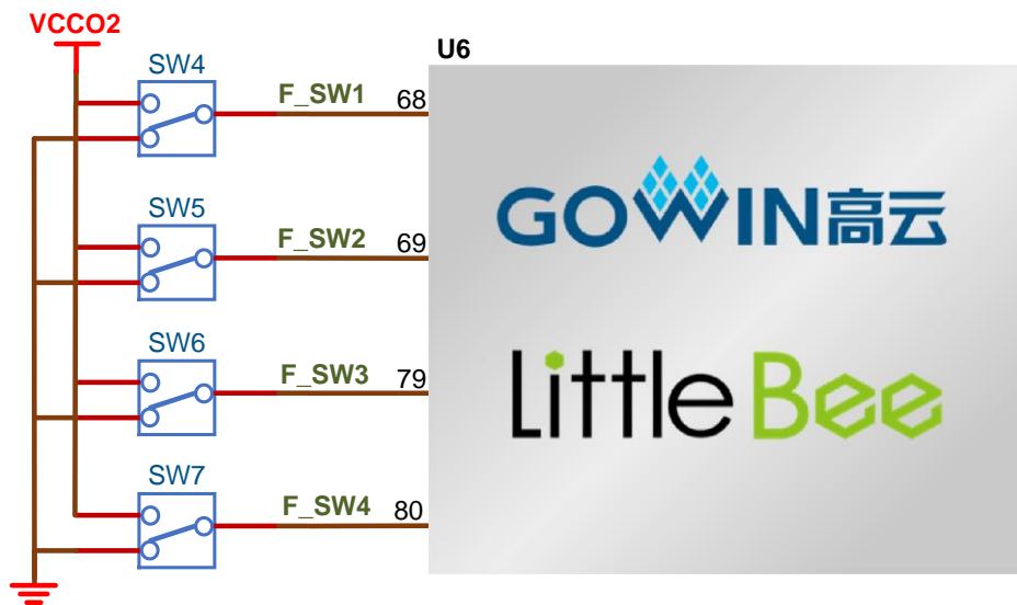
图 3-5 开关电路
