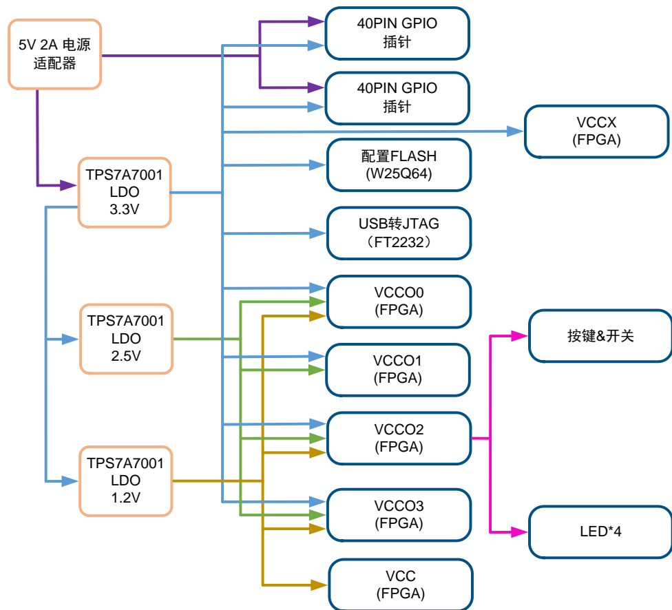
图 3-2 电源系统分配示意图
