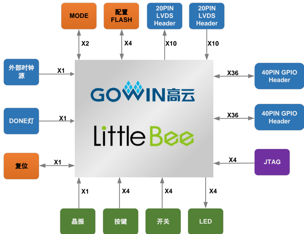
图 2-4 系统框图
