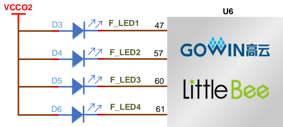
图 3-4 LED 电路
