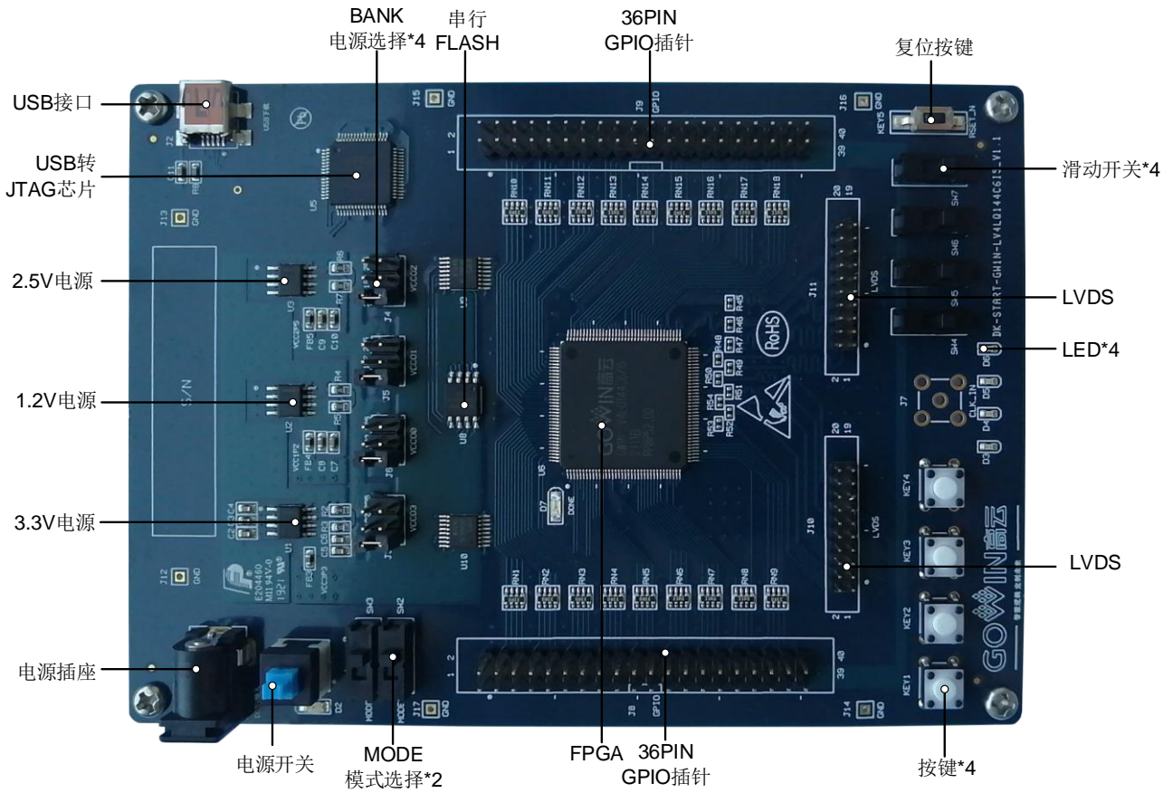
图 2-3 开发板 PCB 组件说明
