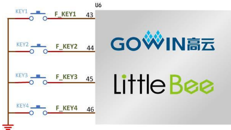
图 3-6 按键电路
