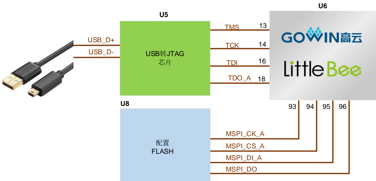
图 3-1 FPGA USB 下载与配置连接示意图
