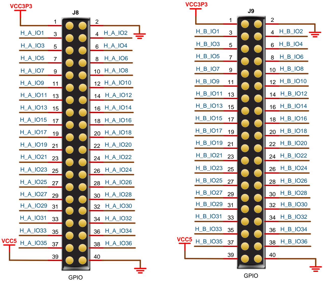
图 3-7 GPIO 电路
