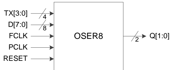
图 3-23 I/O 逻辑的 OSER8 输出示意图
