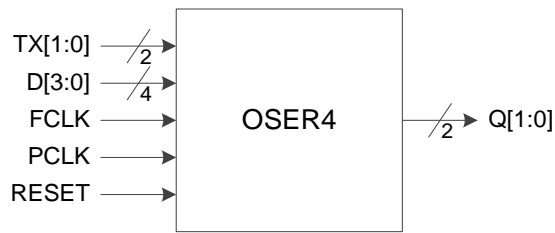
图 3-19 I/O 逻辑的 OSER4 输出示意图
