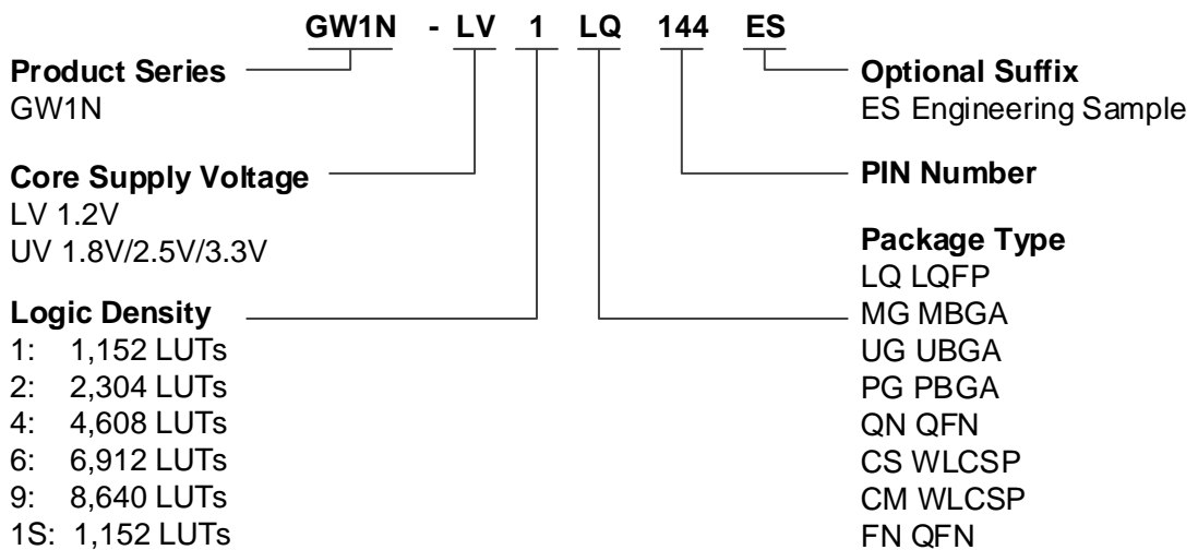
图 5-1 器件命名方法 - ES
