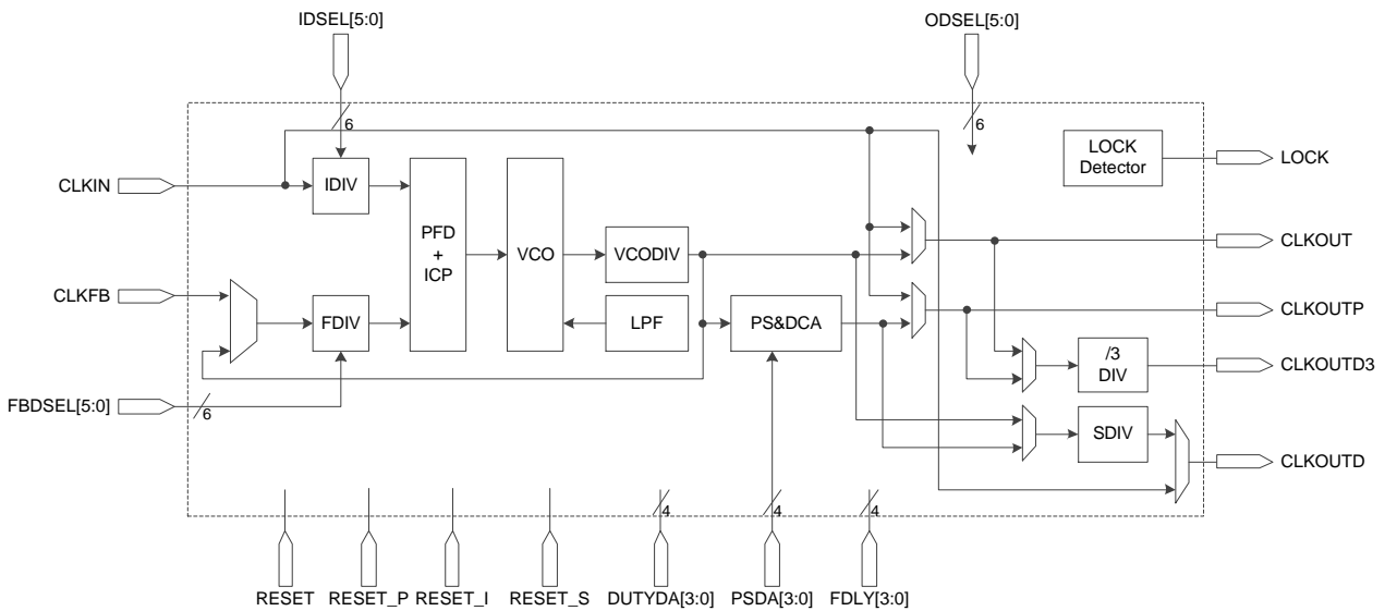
图 3-44 PLL 示意图
