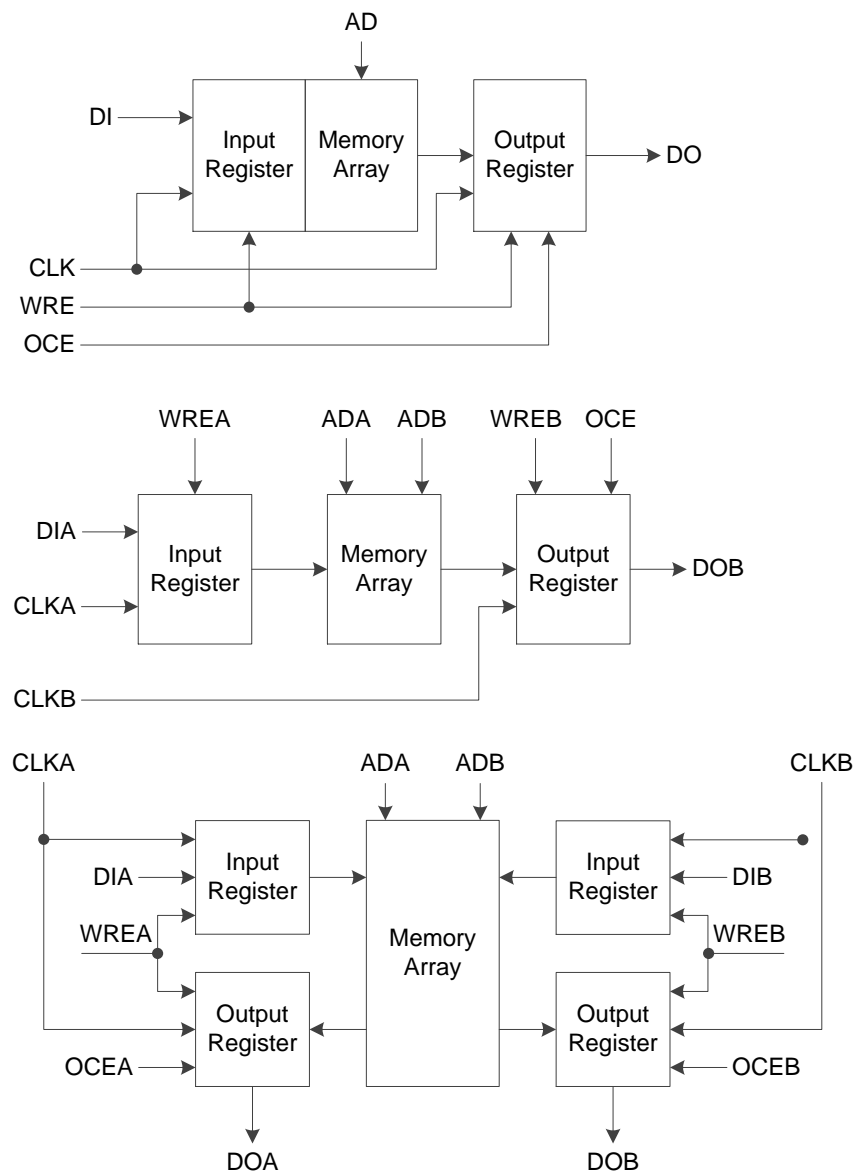
图 3-32 单端口、伪双端口及双端口模式下的流水线模式
