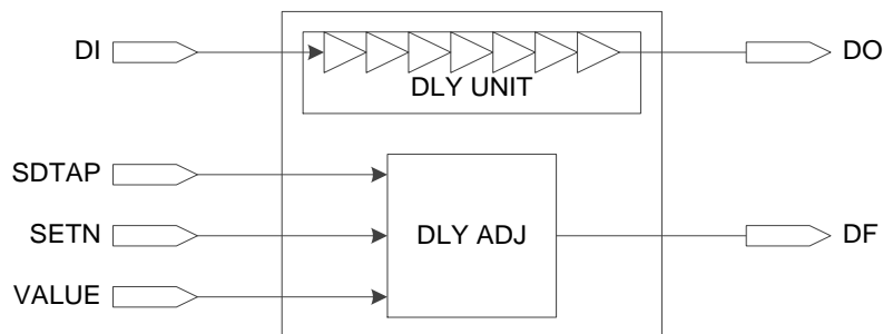
图 3-11 IODELAY 示意图
