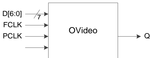
图 3-21 I/O 逻辑的 OVideo 输出示意图
