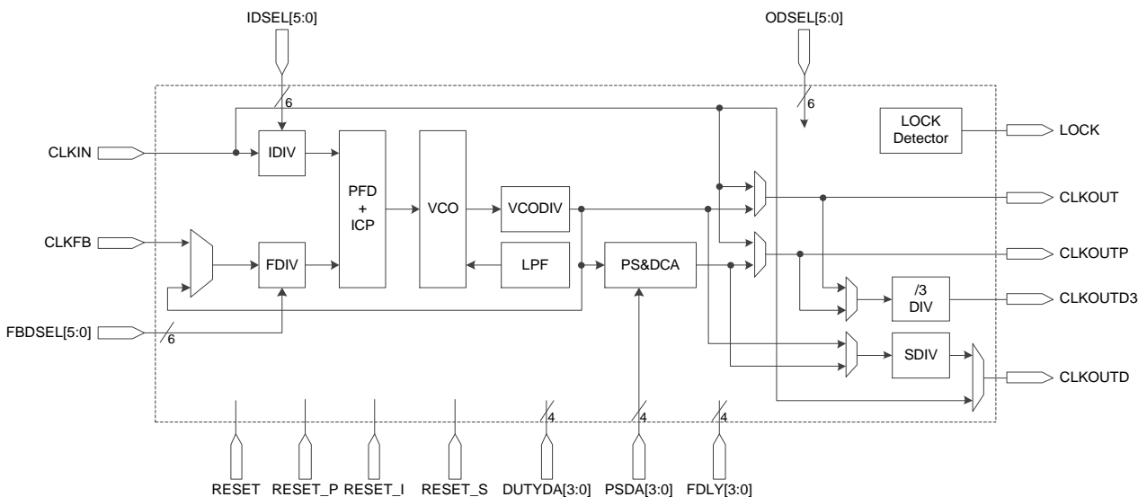
图 3-44 PLL 示意图
