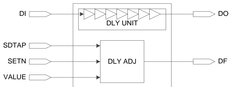
图 3-11 IODELAY 示意图
