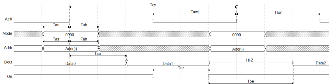
图 4-1 读操作模式
