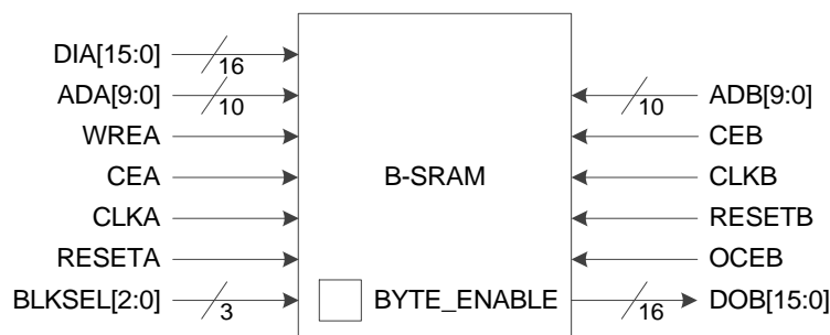
图 3-30 伪双端口存储模式框图 1
