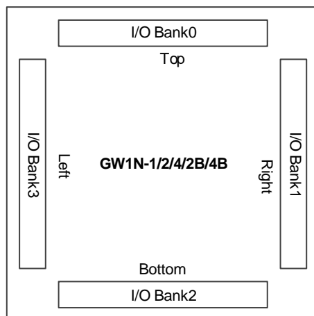
图 3-5 GW1N-1/2/4/2B/4B I/O Bank 分布示意图
