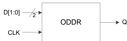
图 3-19 I/O 逻辑的 DDR 输出示意图
