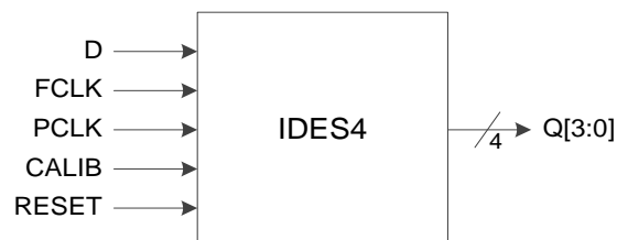
图 3-20 I/O 逻辑的 IDES4 输入示意图
