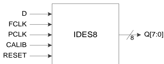
图 3-24 I/O 逻辑的 IDE8 输入示意图
