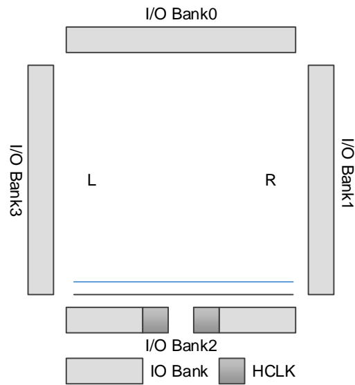
图 3-45 GW1N-2 HCLK 示意图
