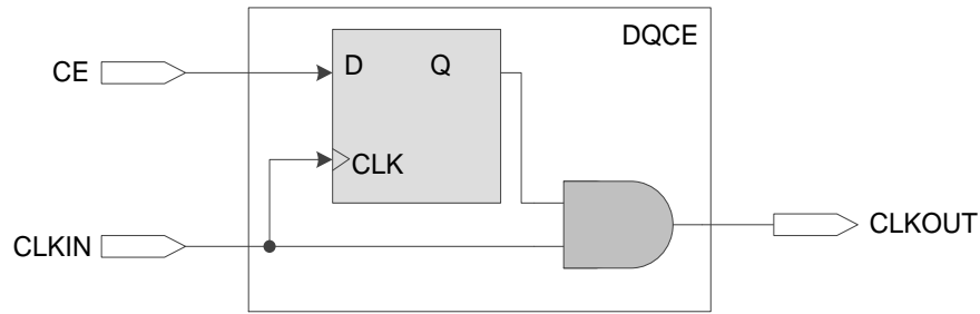
图 3-38 DQCE 结构示意图
