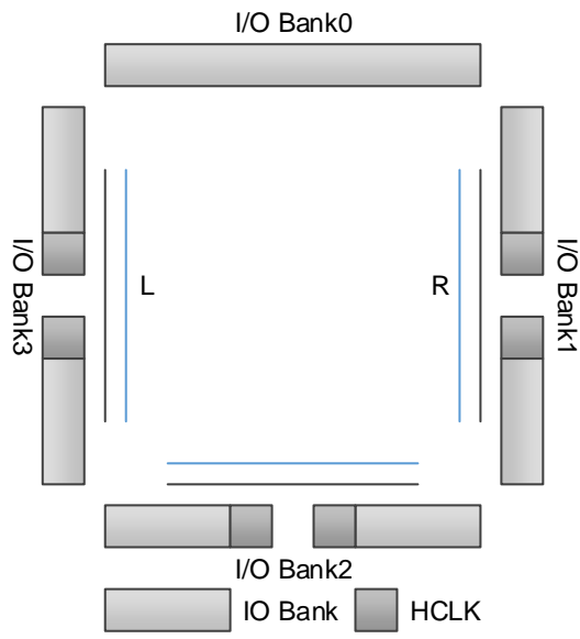
图 3-46 GW1N-4 HCLK 示意图
