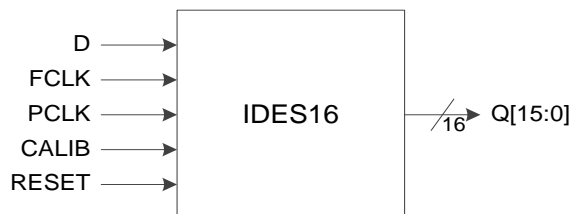
图 3-28 I/O 逻辑的 IDES16 输入示意图
