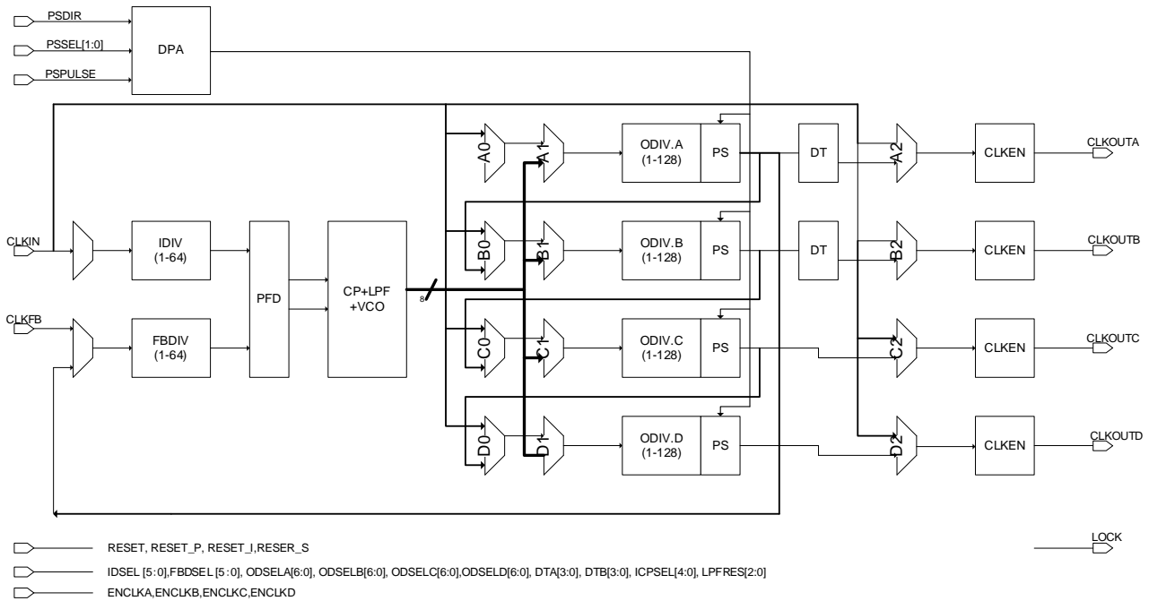
图 3-43 PLL 示意图
