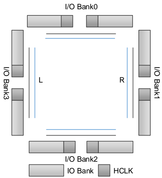
图 3-47 GW1N-9 HCLK 示意图
