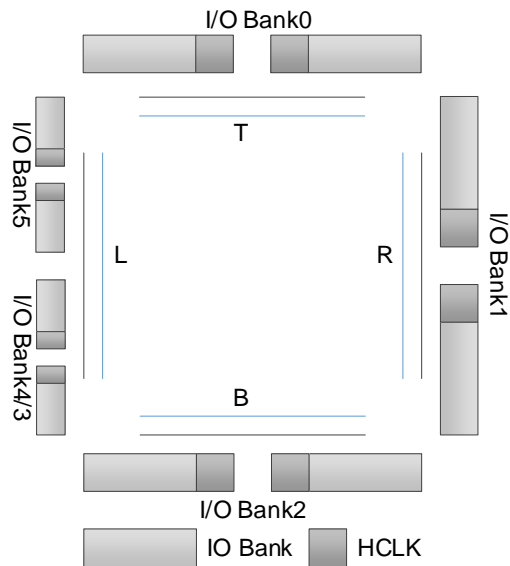
图 3-45 GW1N-2 HCLK 示意图
