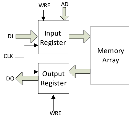
图 3-33 单端口时钟模式
