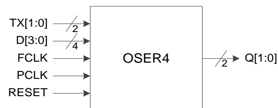
图 3-21 I/O 逻辑的 OSER4 输出示意图
