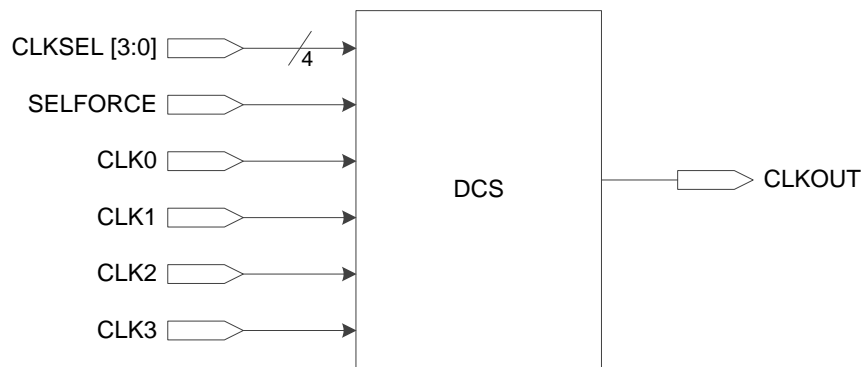
图 3-39 DCS 接口示意图
