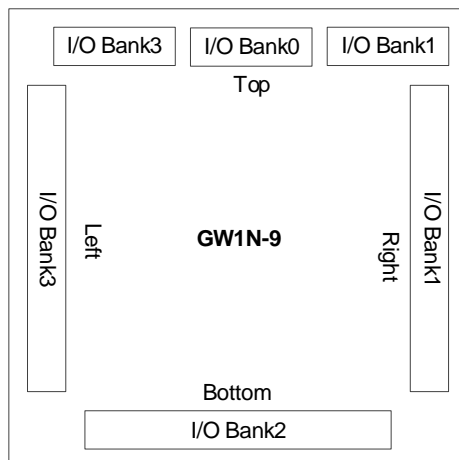
图 3-9 GW1N-9 器件 I/O Bank 分布示意图
