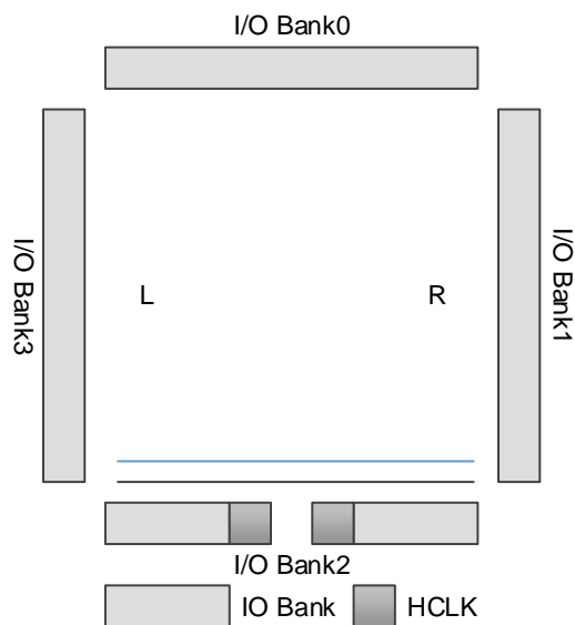
图 3-44 GW1N-1 HCLK 示意图
