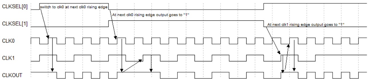
图 3-40 DCS Rising Edge 模式下的时序示意图
