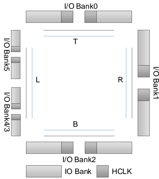
图 3-46 GW1N-4 HCLK 示意图
