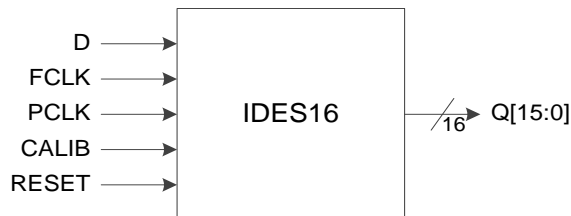
图 3-28 I/O 逻辑的 IDES16 输入示意图
