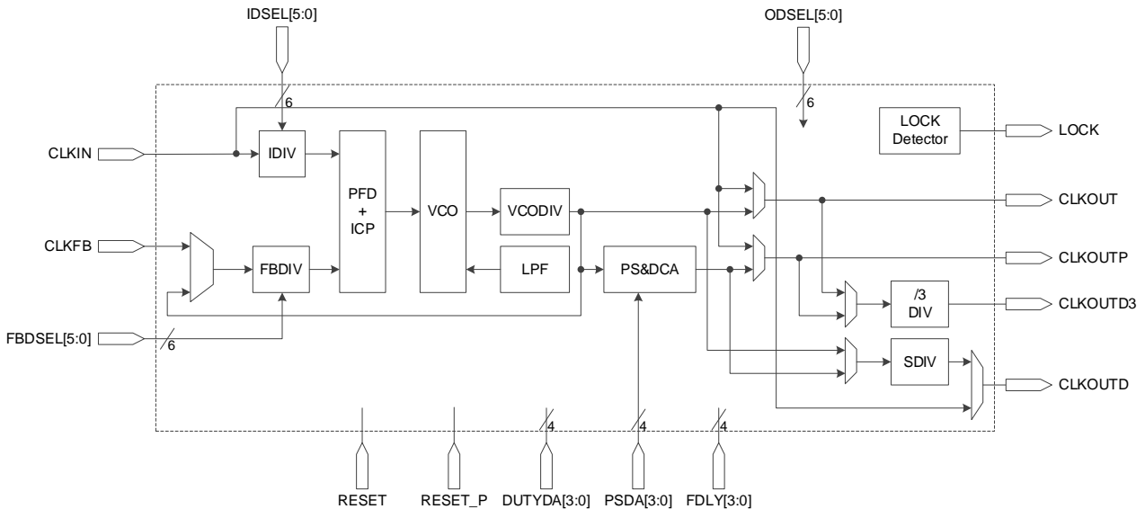
图 3-42 PLL 示意图
