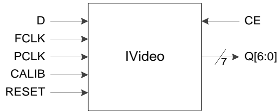
图 3-22 I/O 逻辑的 IVideo 输入示意图
