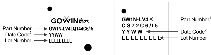
图 5-4 器件封装标识示例
