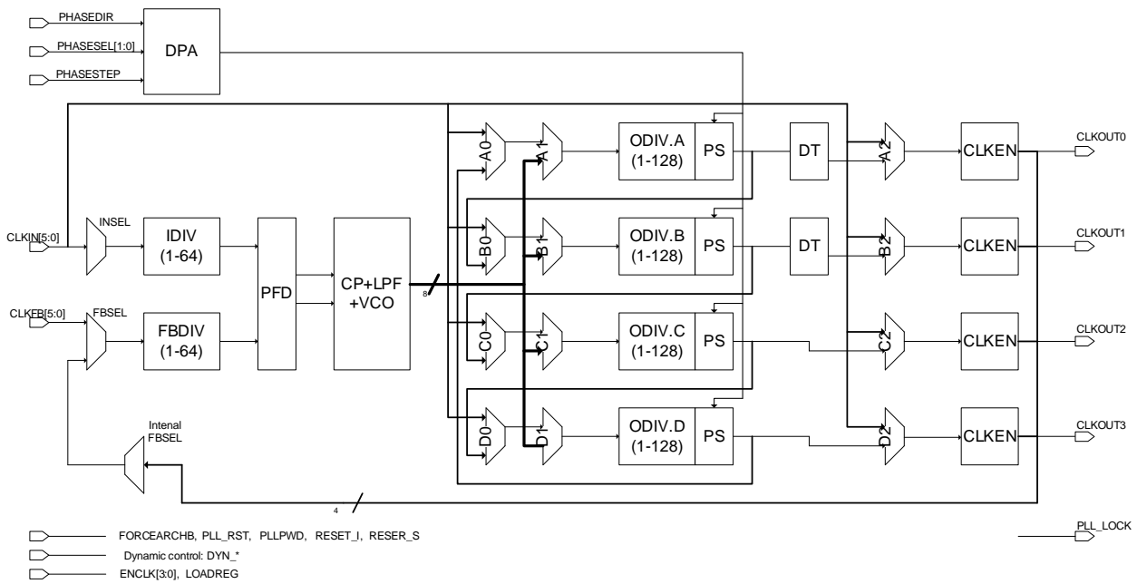
图 3-43 PLL 示意图
