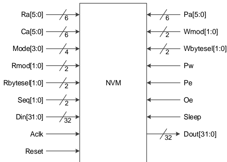
图 3-34 用户闪存端口信号
