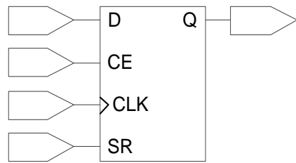
图 3-14 GW1N 的 I/O 寄存器示意图
