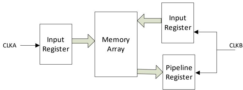
图 3-18 读写时钟模式
