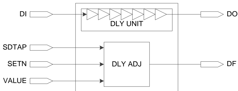
图 3-13 IODELAY 示意图
