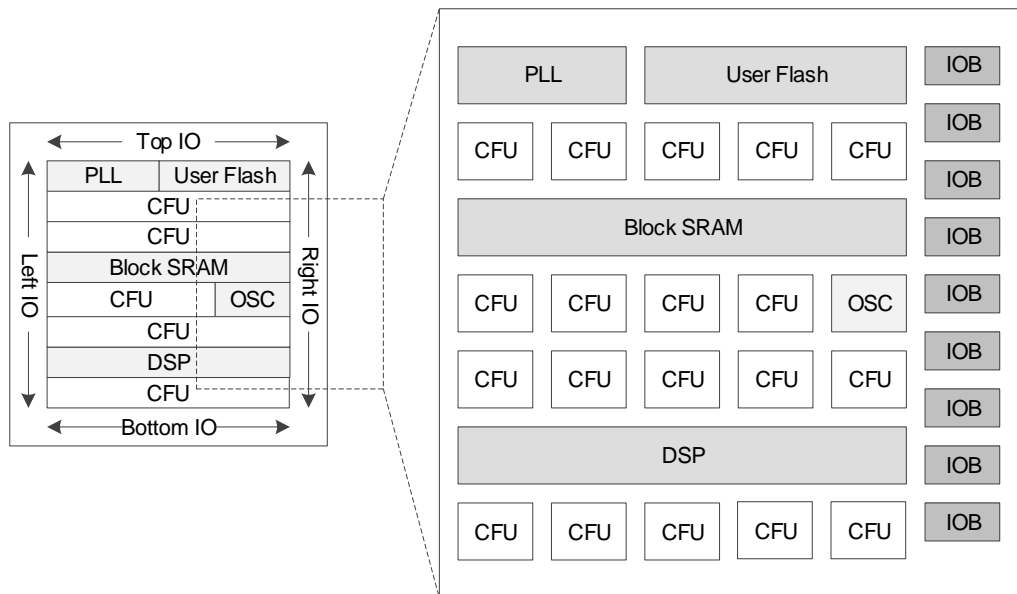
图 3-1 GWIN 系列 FPGA 器件结构示意图 (GWIN-1/1S/4/9)
