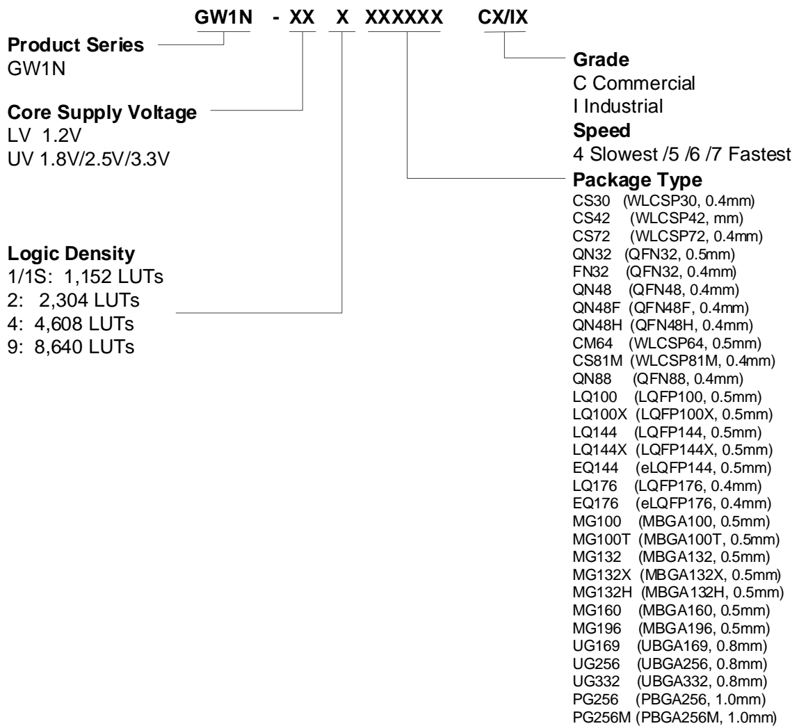
图 5-2 器件命名方法 - Production
