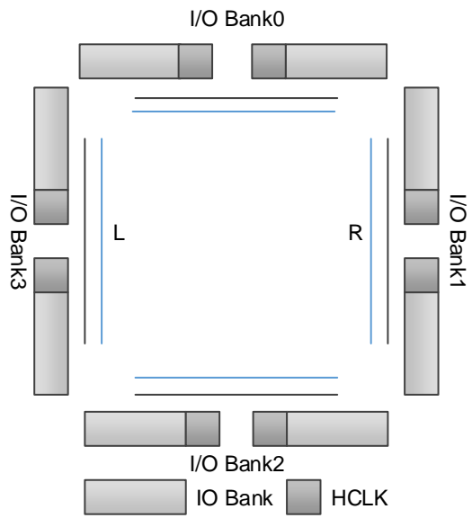
图 3-23 GW1N-9 HCLK 示意图
