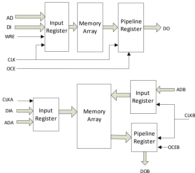
图 3-16 单端口、伪双端口及双端口模式下的流水线模式
