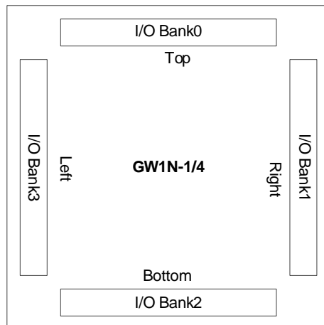
图 3-5 GW1N-1/4 I/O Bank 分布示意图
