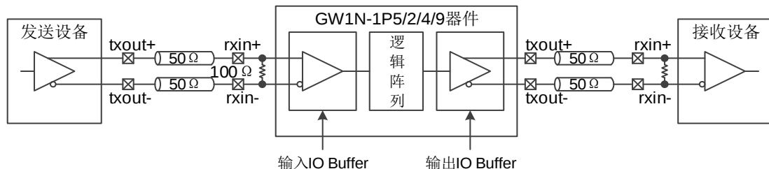
图 2-12 真 LVDS 设计参考框图
