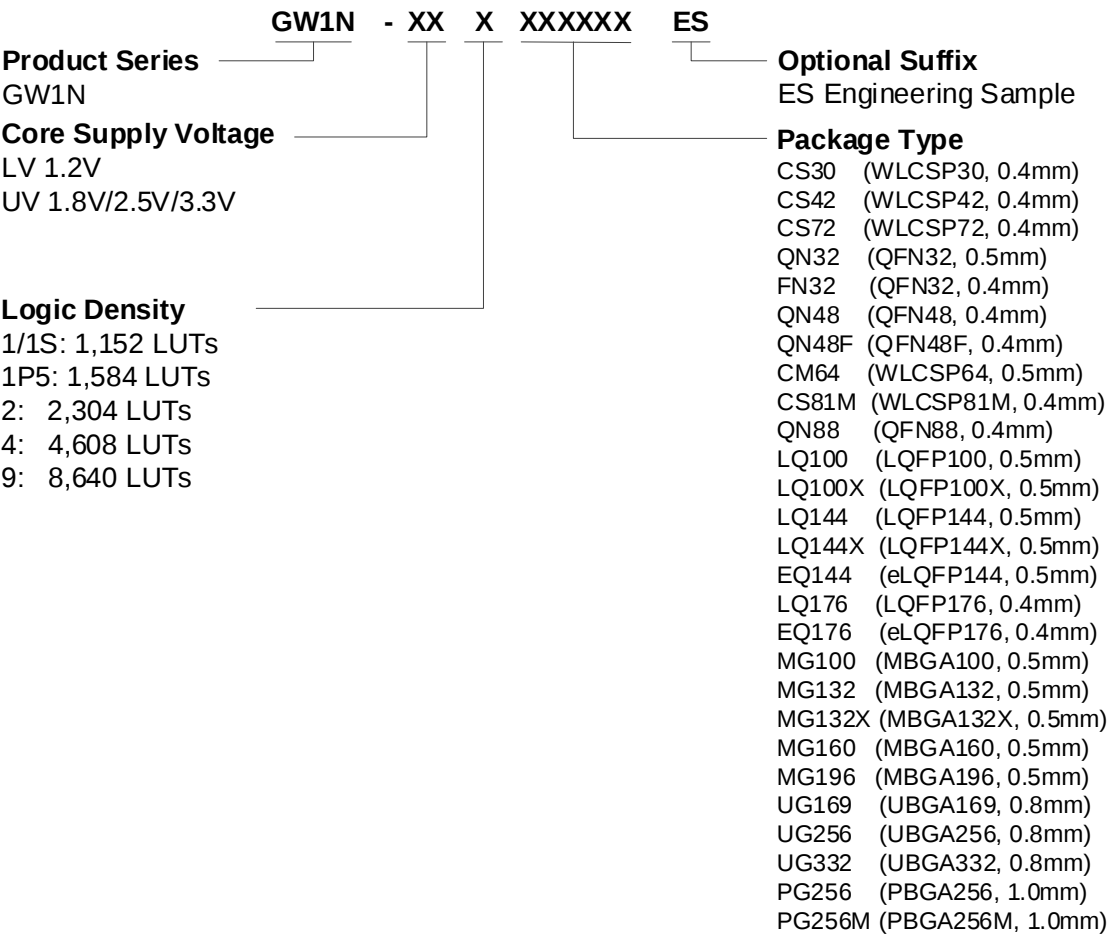
图 4-1 器件命名方法示例 - ES
