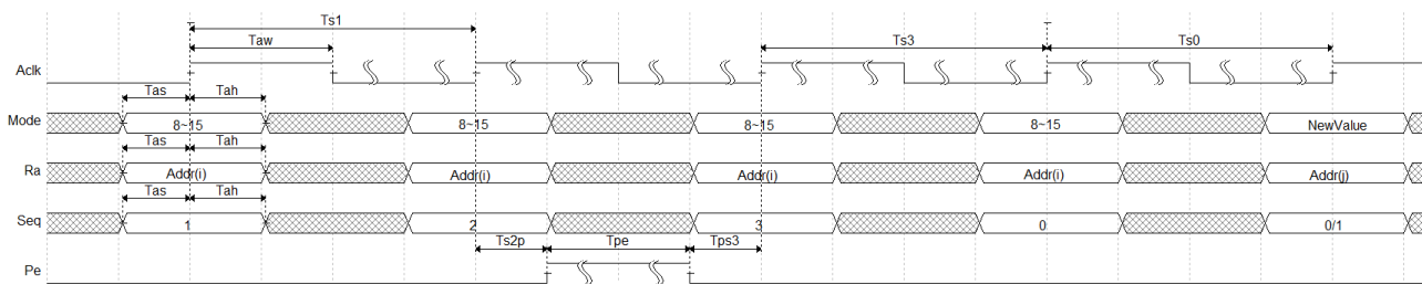
图 3-4 高电平周期
