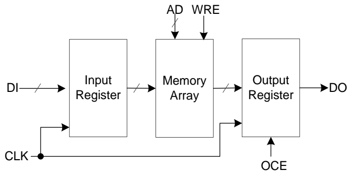
图 3-37 单端口时钟模式
