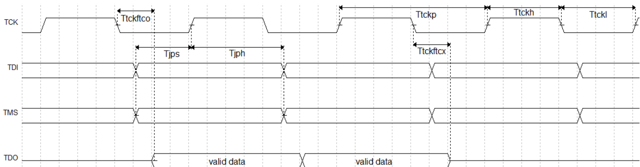
图 4-1 JTAG 编程模式时序示意图
