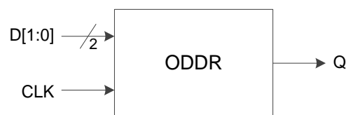
图 3-14 I/O 逻辑的 DDR 输出示意图
