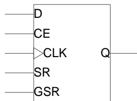
图 3-3 CLS 中的寄存器示意图
