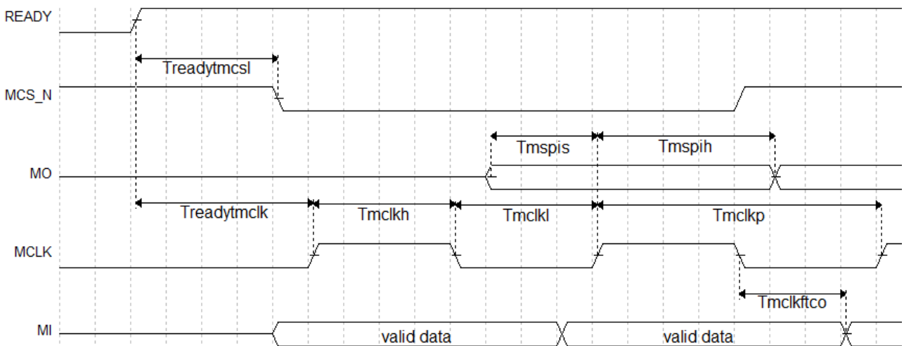
图 4-4 MSPI 编程模式时序示意图
