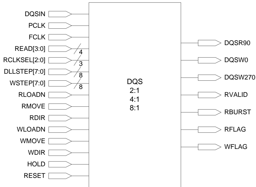
图 3-47 DQS 示意图
