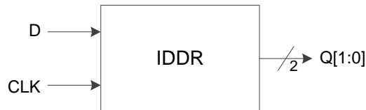
图 3-13 I/O 逻辑的 DDR 输入示意图
