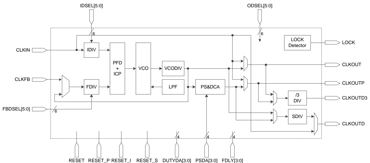
图 3-45 PLL 示意图
