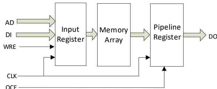
图 3-10 单端口、伪双端口及双端口模式下的流水线模式
