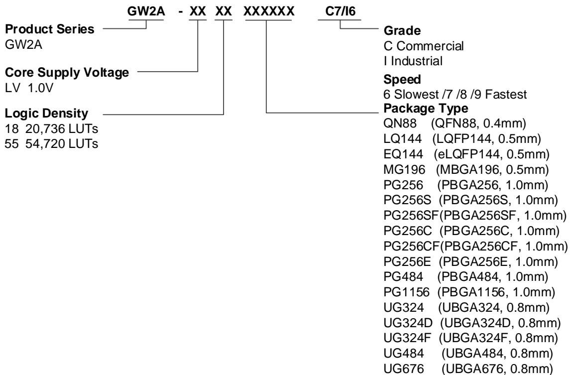
图 5-2 器件命名方法示例-Production
