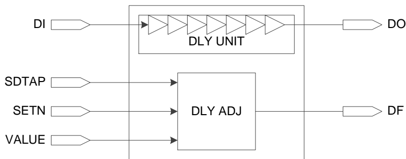
图 3-7 IODELAY 示意图
