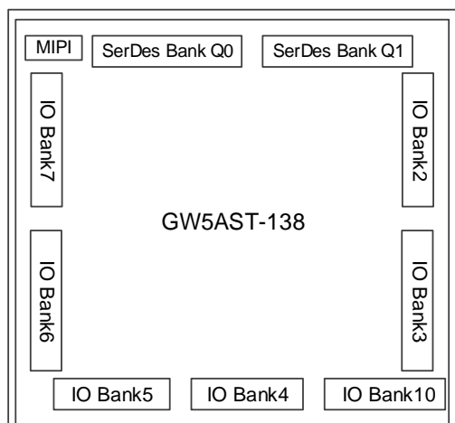
图 2-4 GW5AST-138 GPIO Bank 分布示意图
