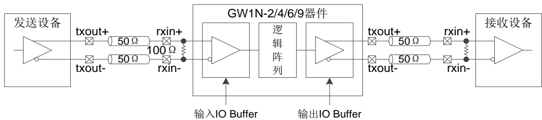
图 3-6 真 LVDS 设计参考框图
