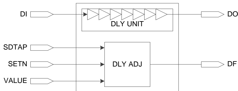
图 3-9 IODELAY 示意图
