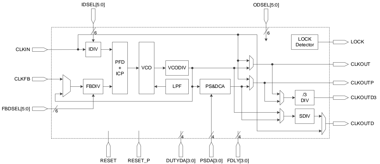
图 3-38 PLL 示意图
