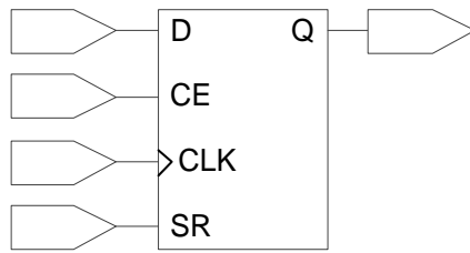
图 3-10 GW1NR 的 I/O 寄存器示意图
