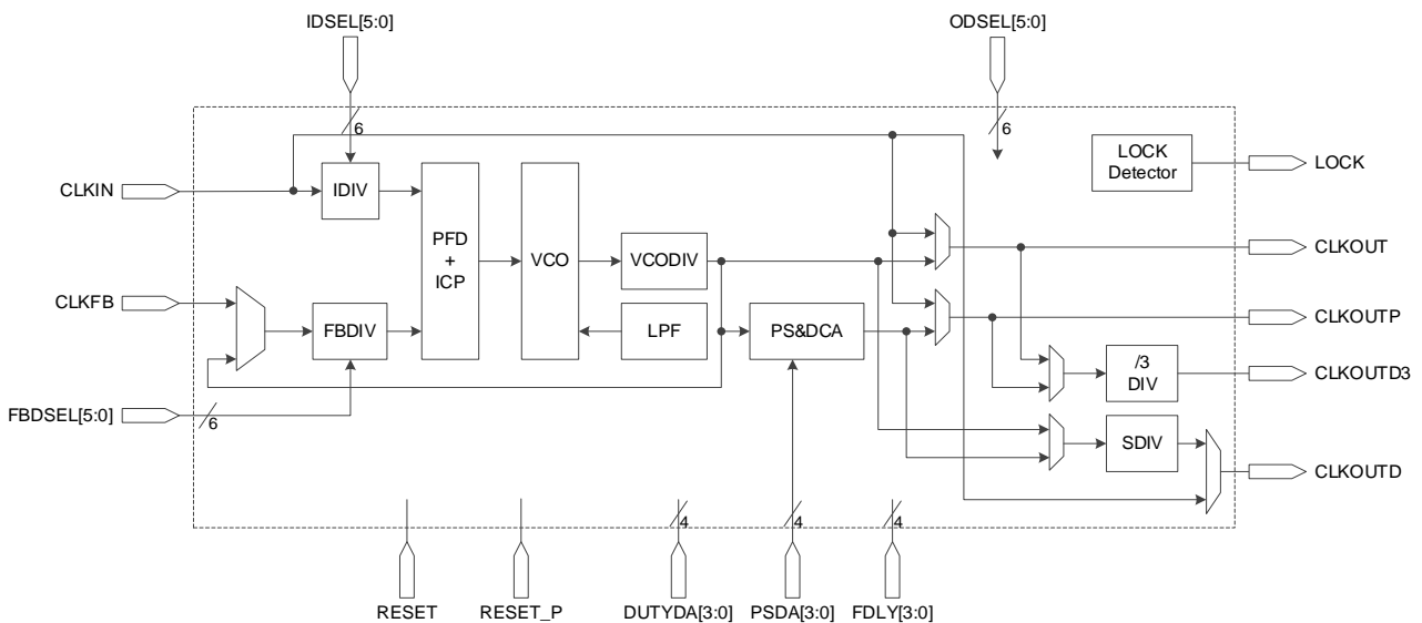
图 3-33 PLL 示意图
