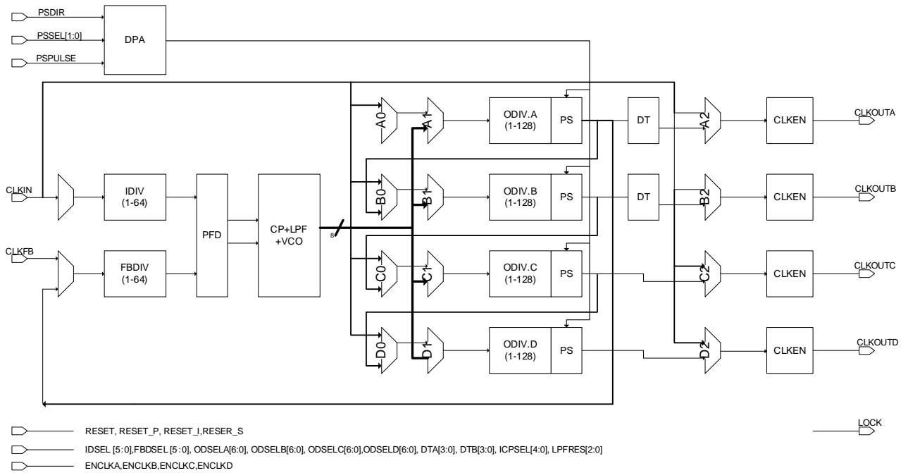
图 3-34 PLL 示意图
