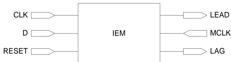
图 3-13 GW1NR 的 IEM 示意图
