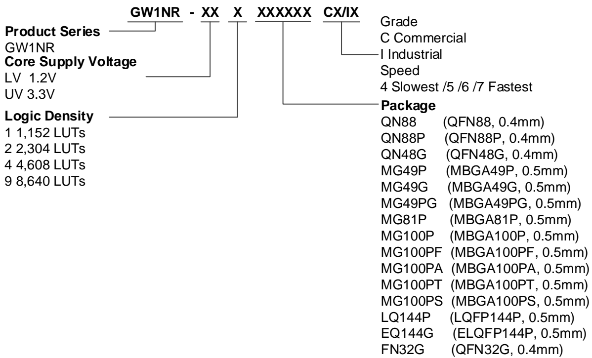
图 5-2 GW1NR 器件命名方法-Production
