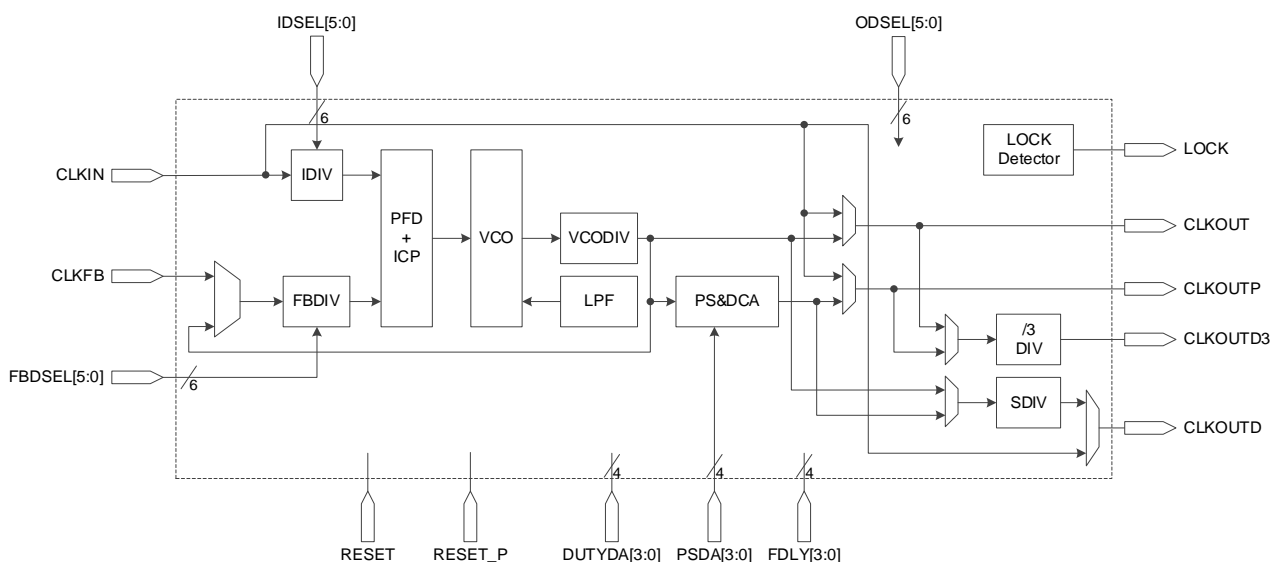
图 3-33 PLL 示意图
