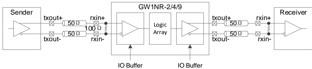
图 3-8 真 LVDS 设计参考框图
