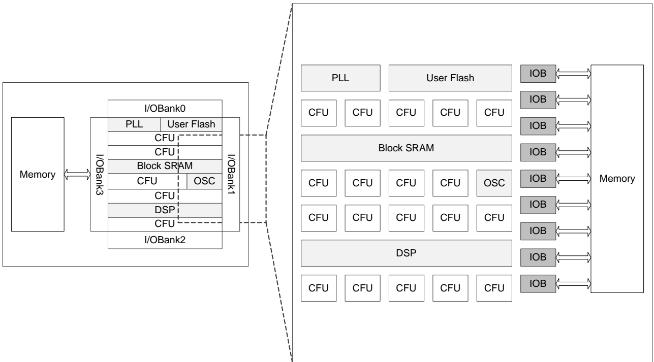
图 3-1 GW1NR-1/4/9 器件结构示意图
