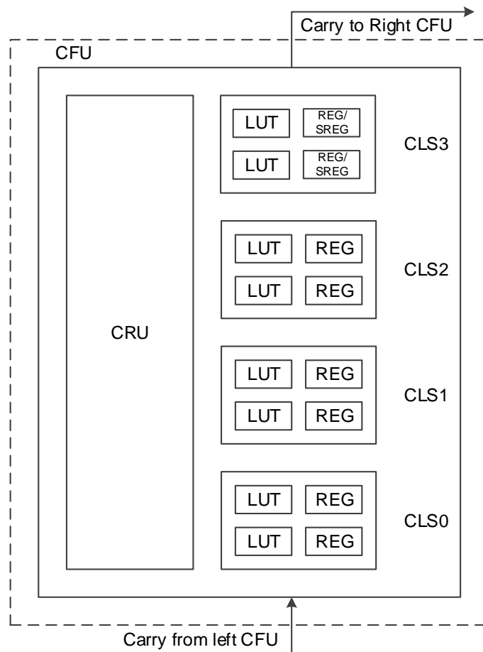
图 3-3 CFU 结构示意图
