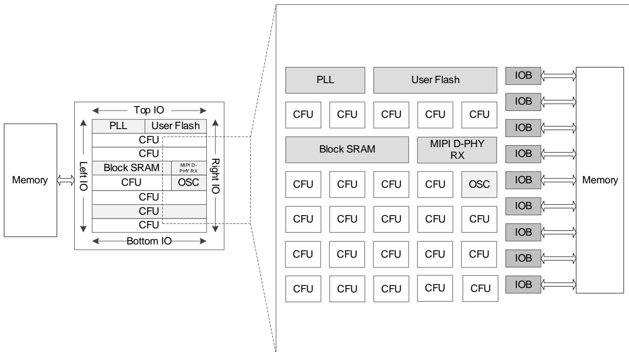
图 3-2 GW1NR-2 器件结构示意图
