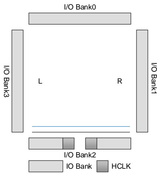
图 3-36 GW1NR-2 HCLK 示意图
