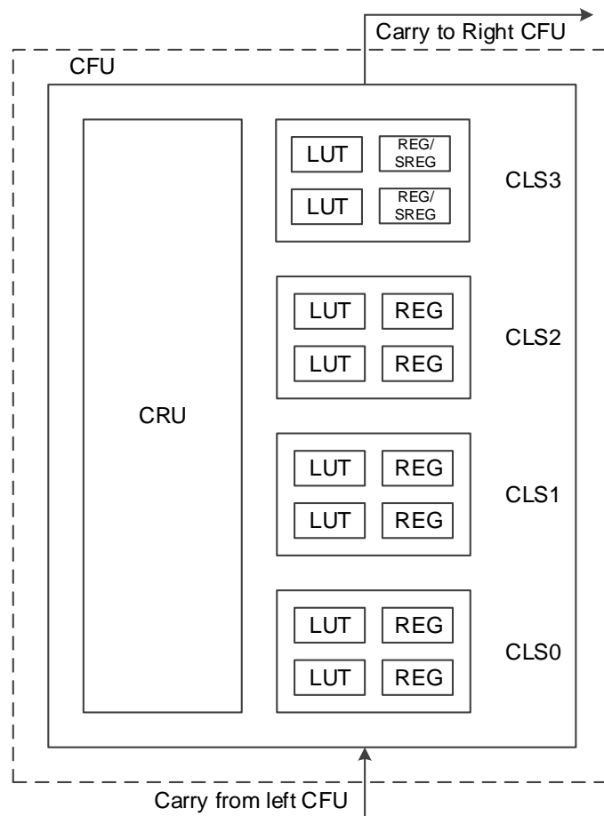
图 3-5 CFU 结构示意图
