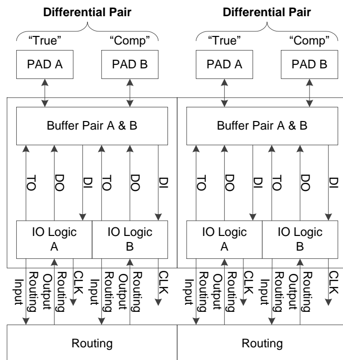
图 3-7 IOB 结构示意图
