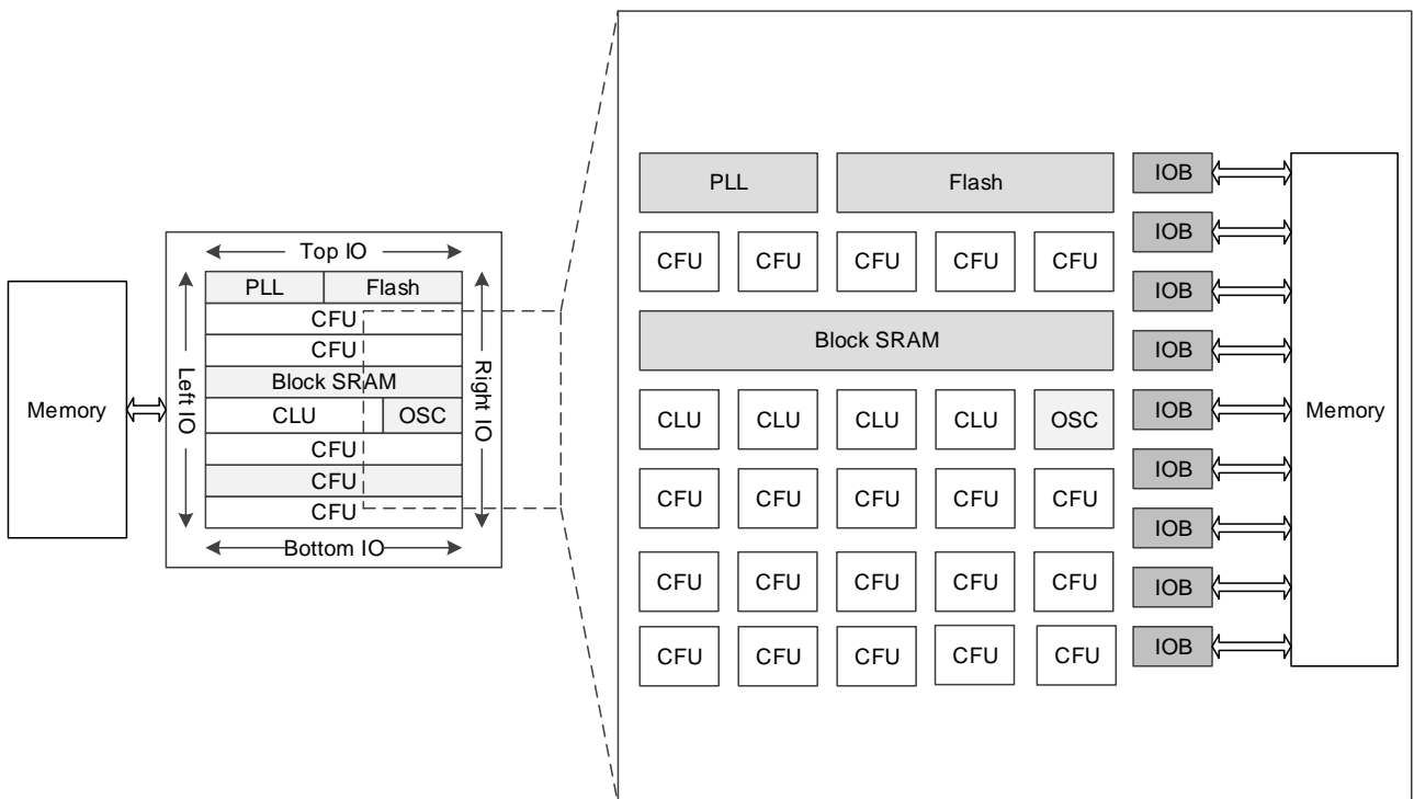
图 3-1 GW1NR-1 器件结构示意图
