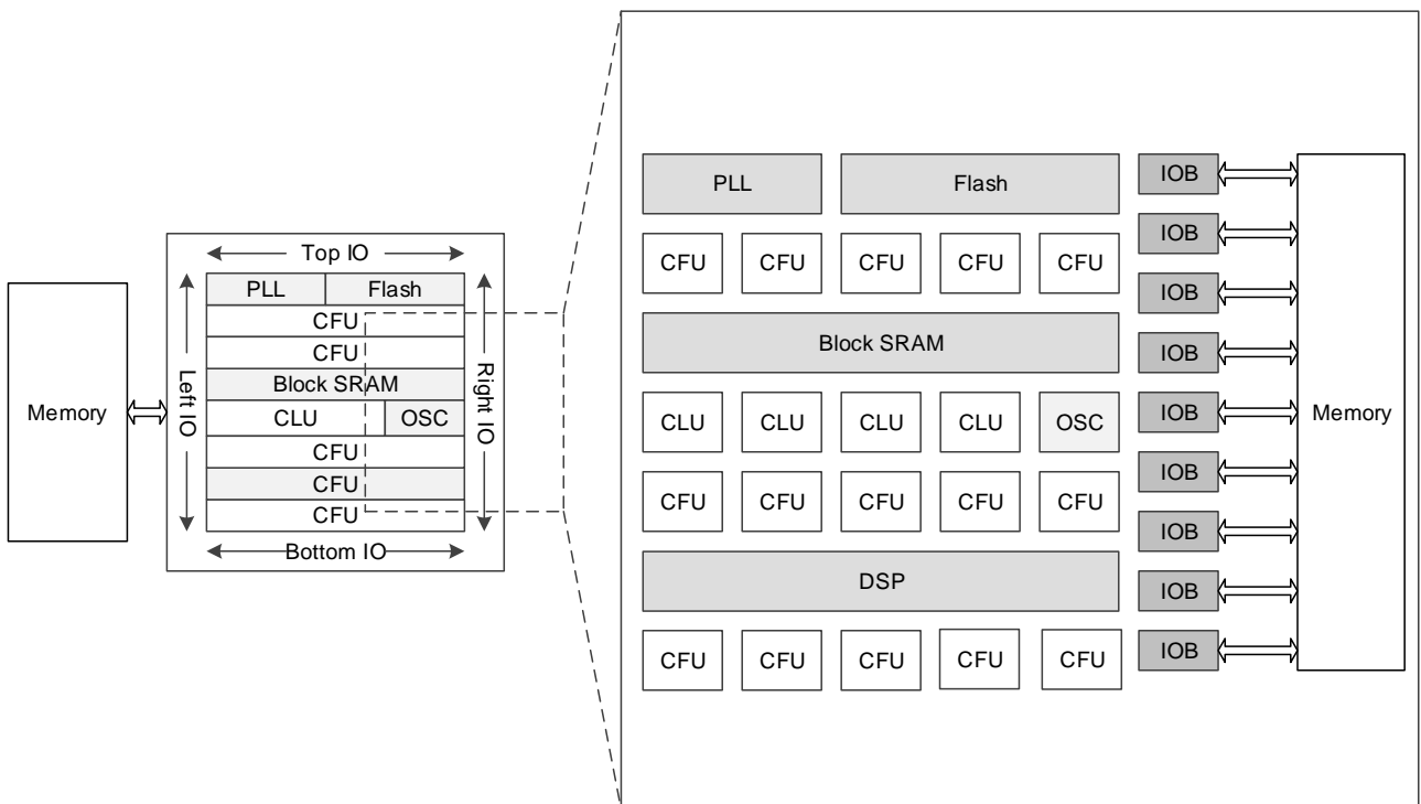
图 3-3 GW1NR-9 器件结构示意图
