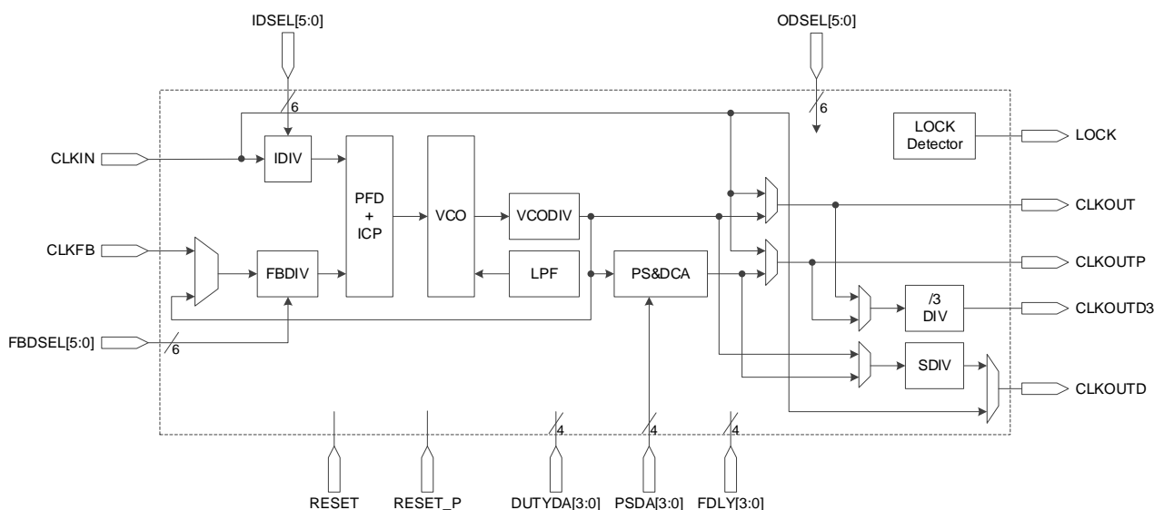
图 3-35 PLL 示意图
