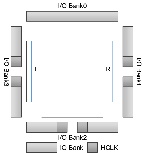
图 3-39 GW1NR-4 HCLK 示意图
