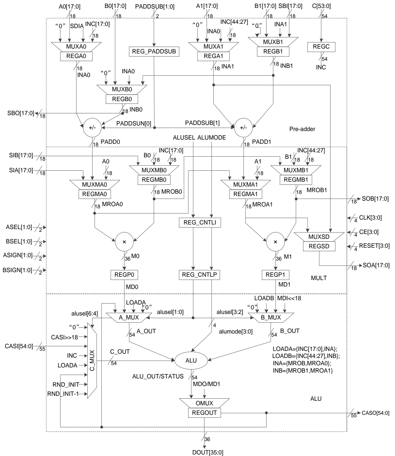
图 3-34 DSP 宏单元
