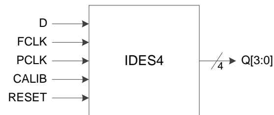
图 3-20 I/O 逻辑的 IDES4 输入示意图
