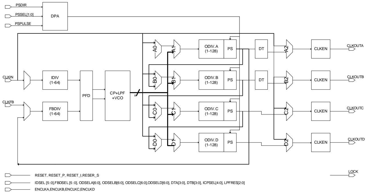
图 3-36 PLL 示意图
