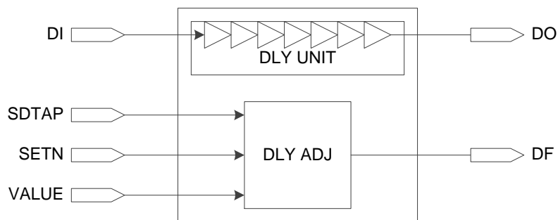
图 3-13 IODELAY 示意图
