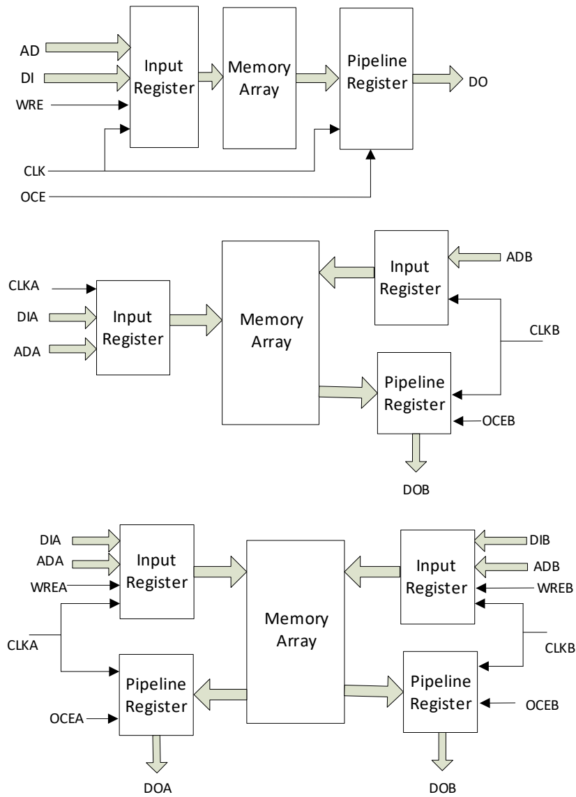
图 3-12 单端口、伪双端口及双端口模式下的流水线模式
