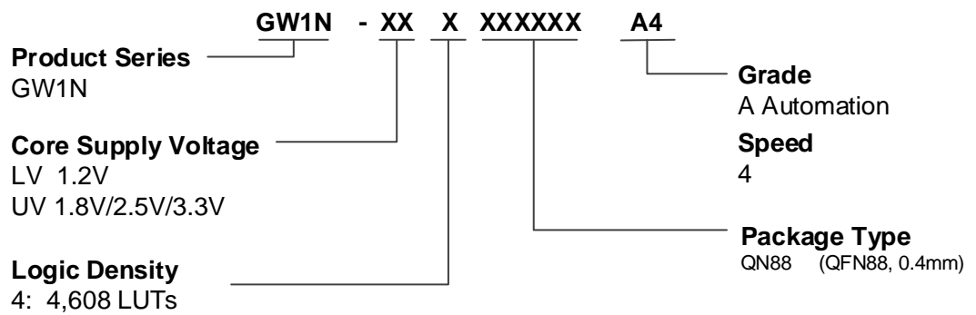
图 5-1 器件命名方法 - Production
