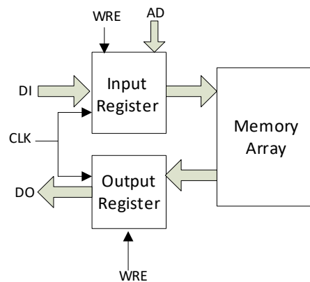
图 3-15 单端口时钟模式
