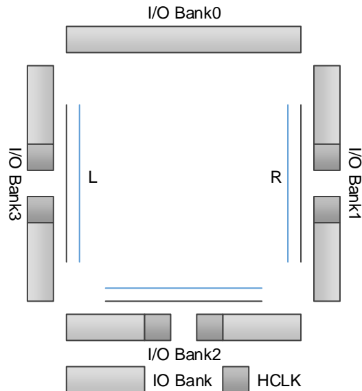
图 3-17 GW1N-4 HCLK 示意图
