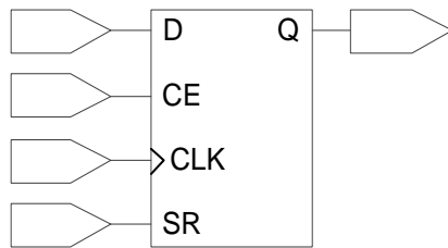
图 3-12 GW1N 的 I/O 寄存器示意图
