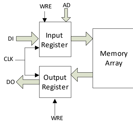
图 3-17 单端口时钟模式
