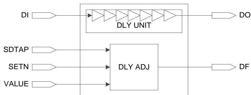
图 3-11 IODELAY 示意图
