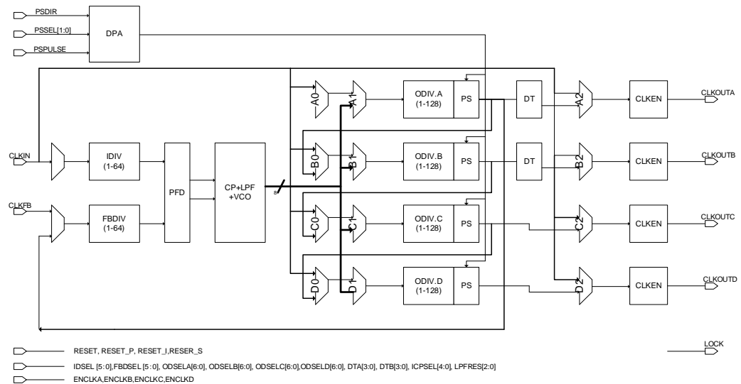
图 3-18 PLL 示意图(GW1N-2)
