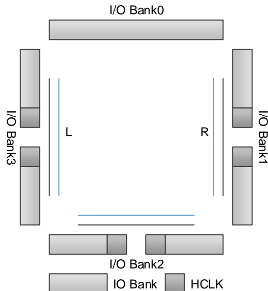
图 3-21 GW1N-4 HCLK 示意图
