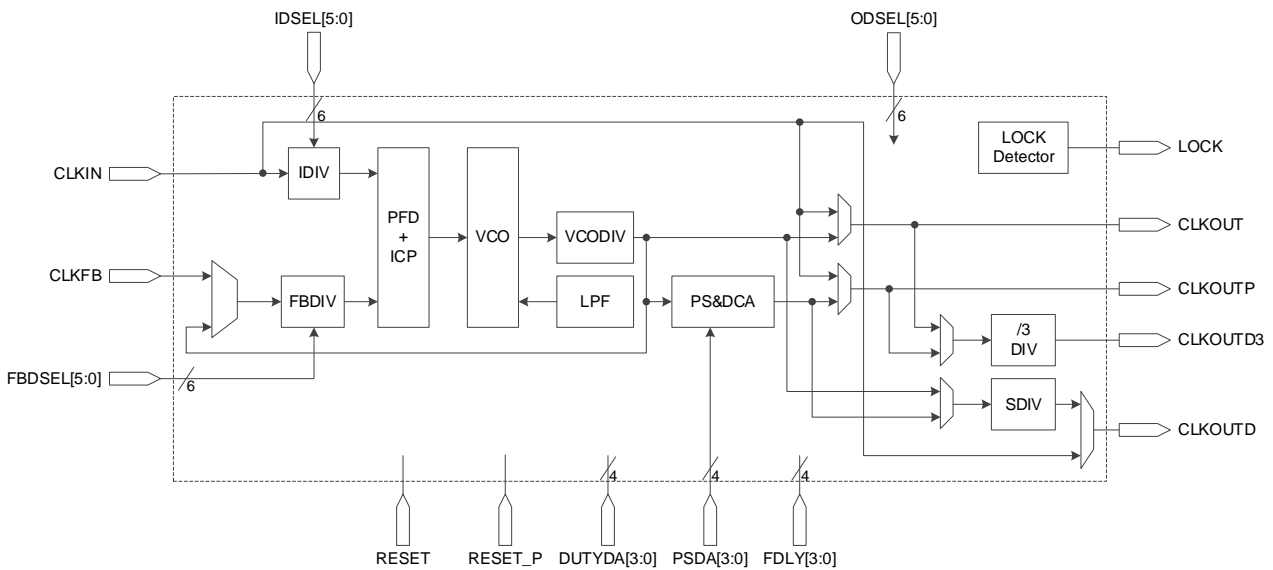
图 3-19 PLL 示意图(GWIN-4)
