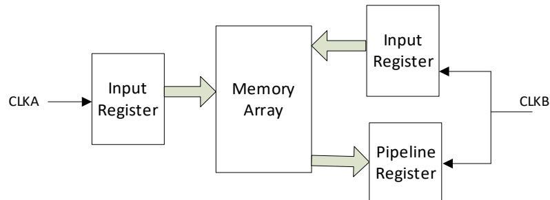
图 3-16 读写时钟模式
