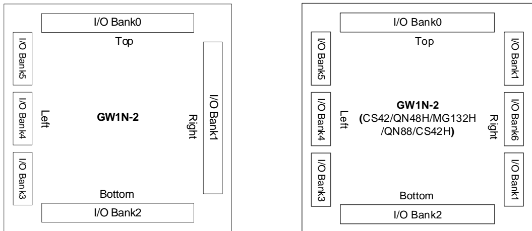
图 3-6 GW1N-2 I/O Bank 分布示意图
