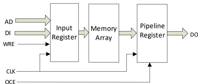
图 3-14 单端口、伪双端口及双端口模式下的流水线模式
