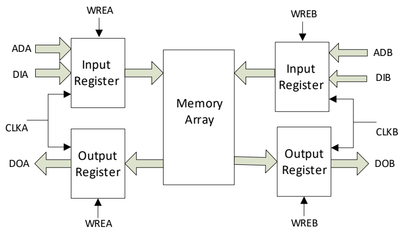
图 3-15 独立时钟模式
