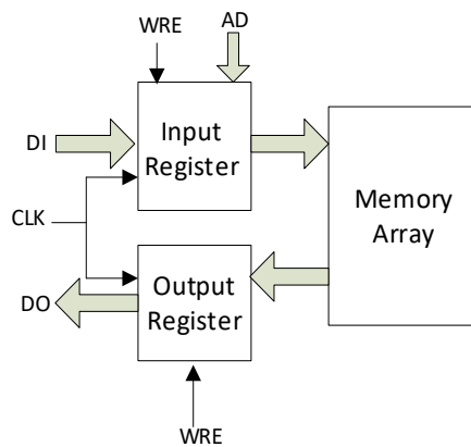
图 3-14 单端口时钟模式
