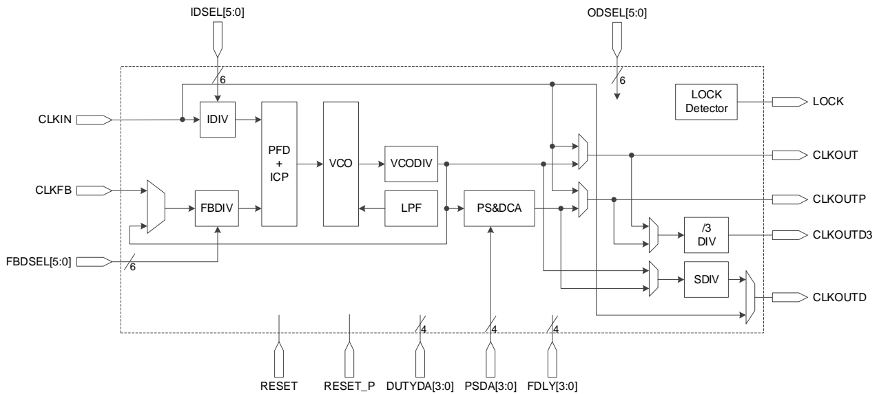
图 3-22 PLL 示意图
