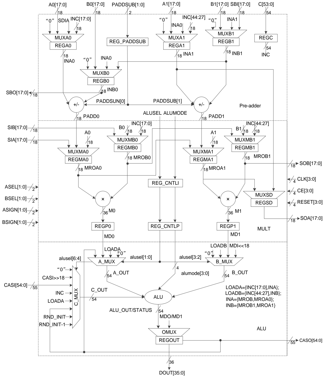
图 3-15 DSP 宏单元
