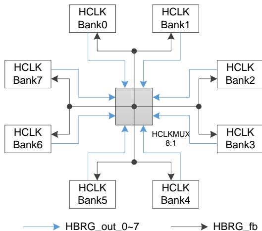
图 3-23 GW2A HCLK 示意图
