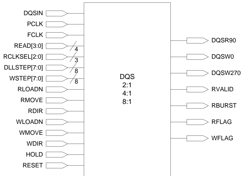
图 3-24 DQS 示意图
