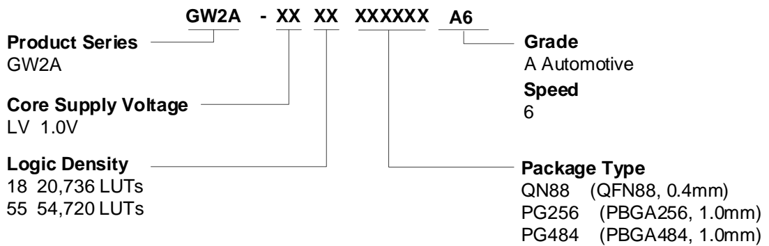
图 5-1 器件命名方法示例-Production
